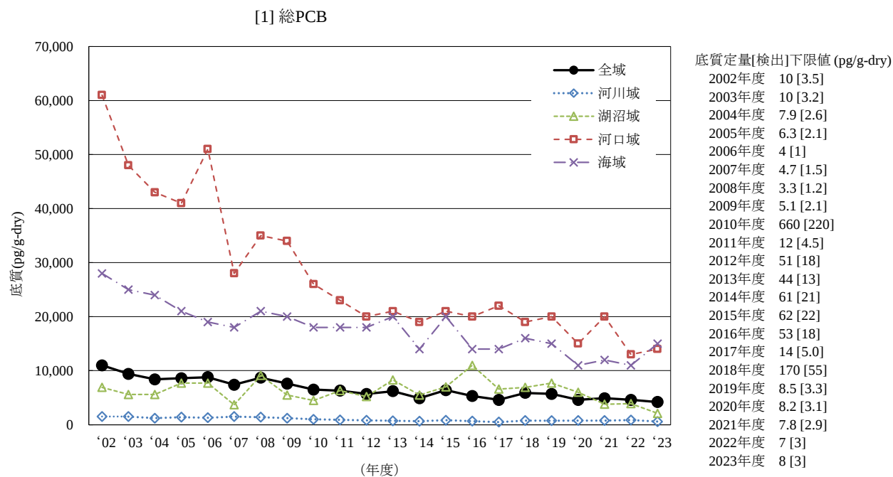
図 3-1-2 総 PCB の底質の経年変化 (幾何平均値)
