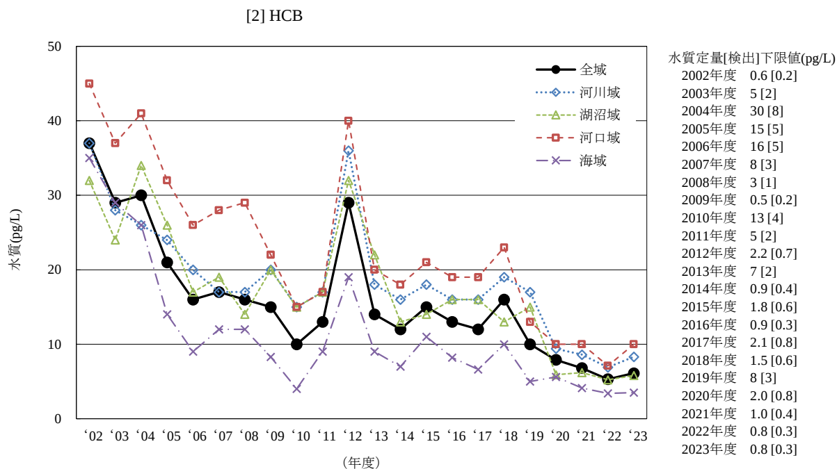
図 3-2-1 HCB の水質の経年変化 (幾何平均値)
