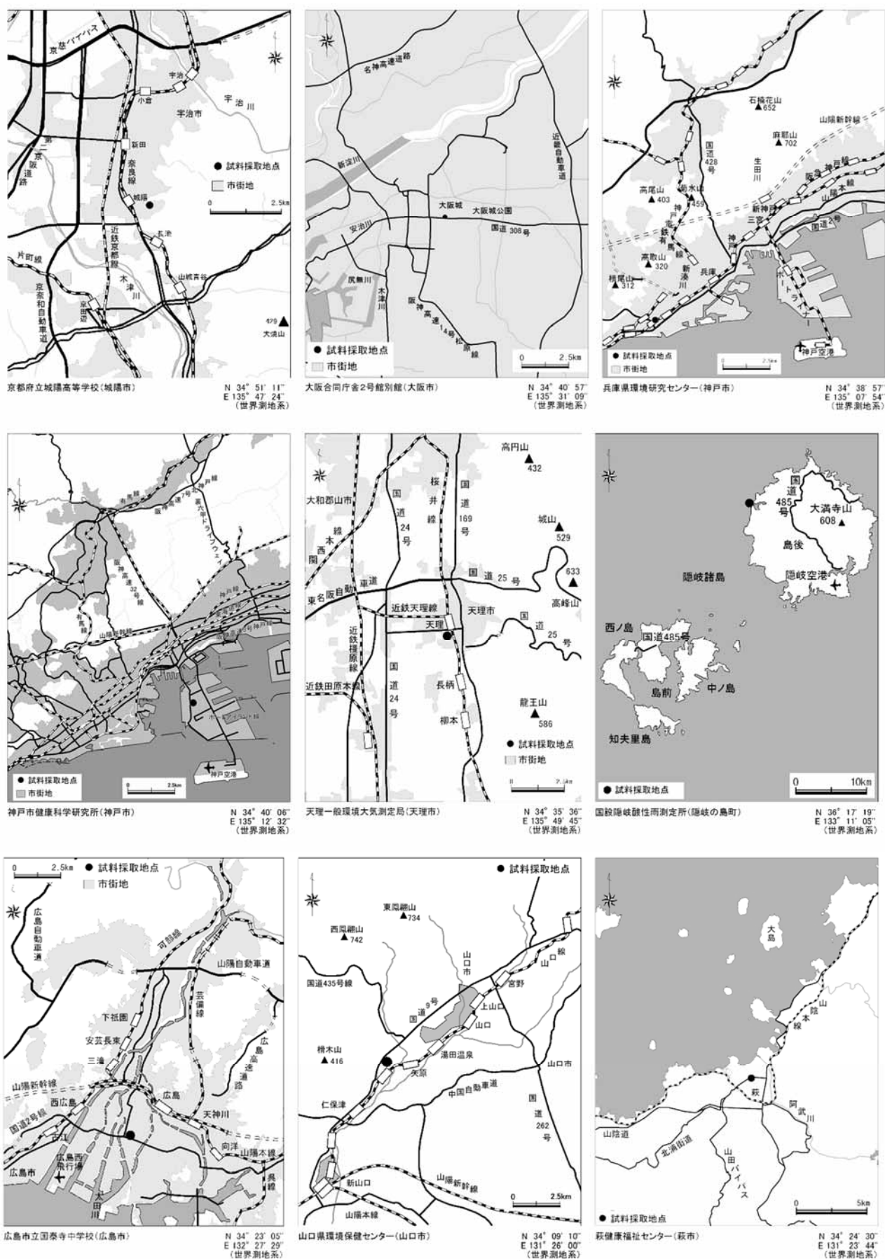
図 1-8 (3/4) 2023 年度モニタリング調査地点 (大気) 詳細
