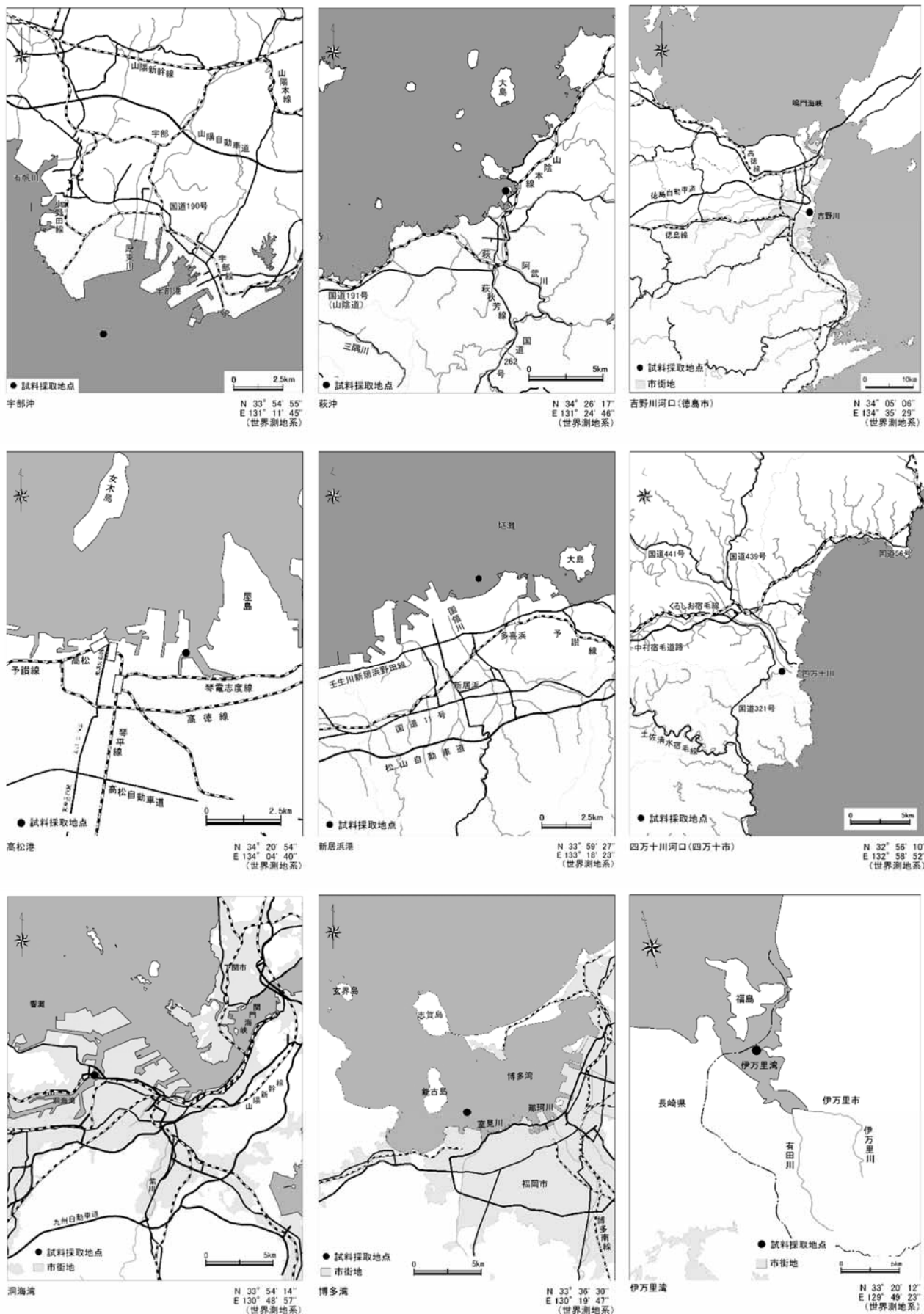
図 1-4 (6/7) 2023 年度モニタリング調査地点 (底質) 詳細
