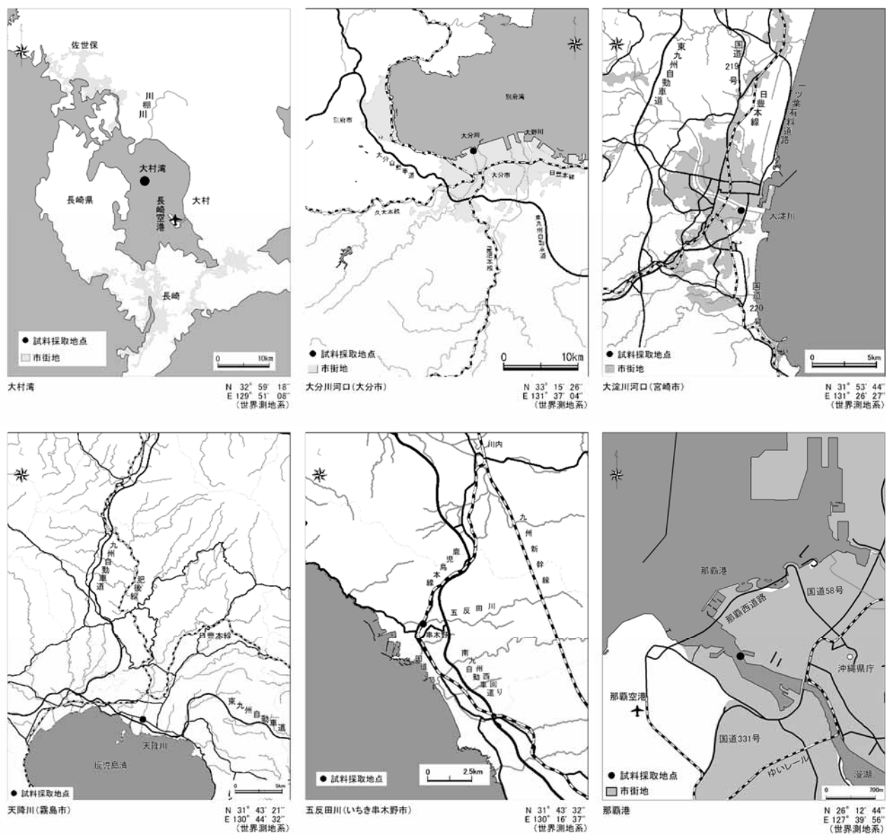
図 1-4 (7/7) 2023 年度モニタリング調査地点 (底質) 詳細
