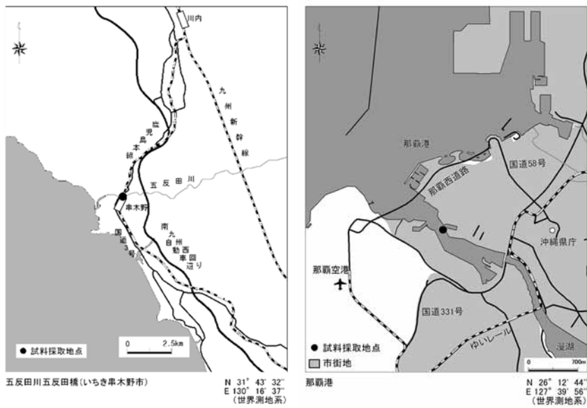
図 1-2 (6/6) 2023 年度モニタリング調査地点 (水質) 詳細
