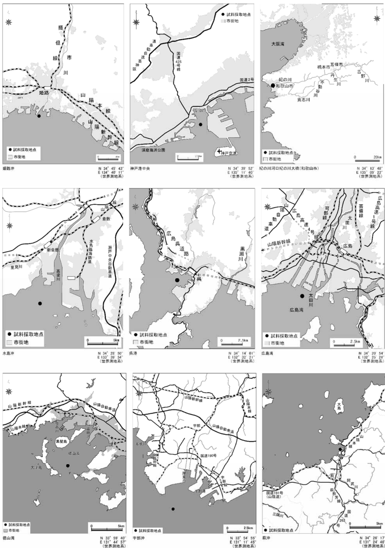
図 1-2 (4/6) 2023 年度モニタリング調査地点 (水質) 詳細
