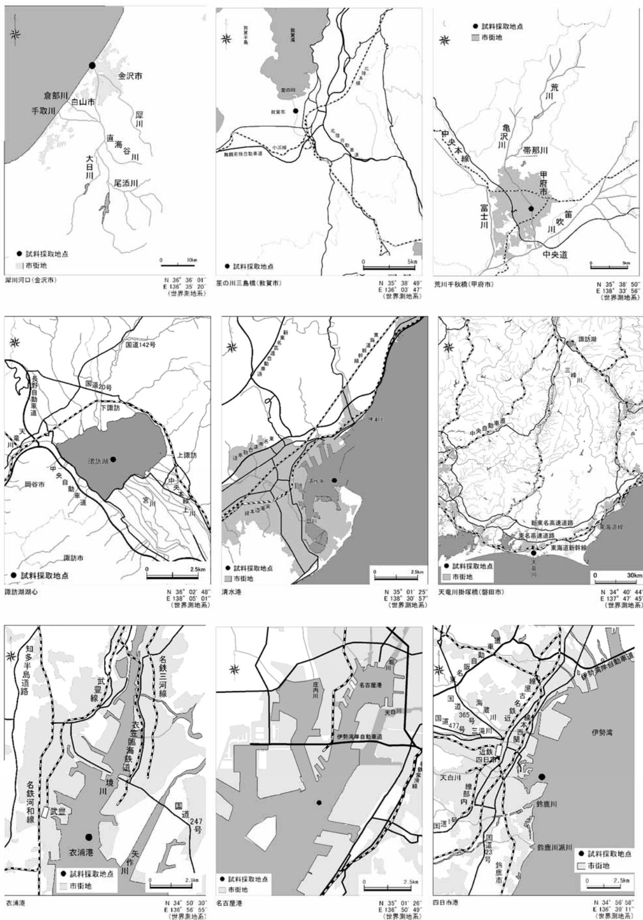
図 1-4 (3/7) 2023 年度モニタリング調査地点 (底質) 詳細
