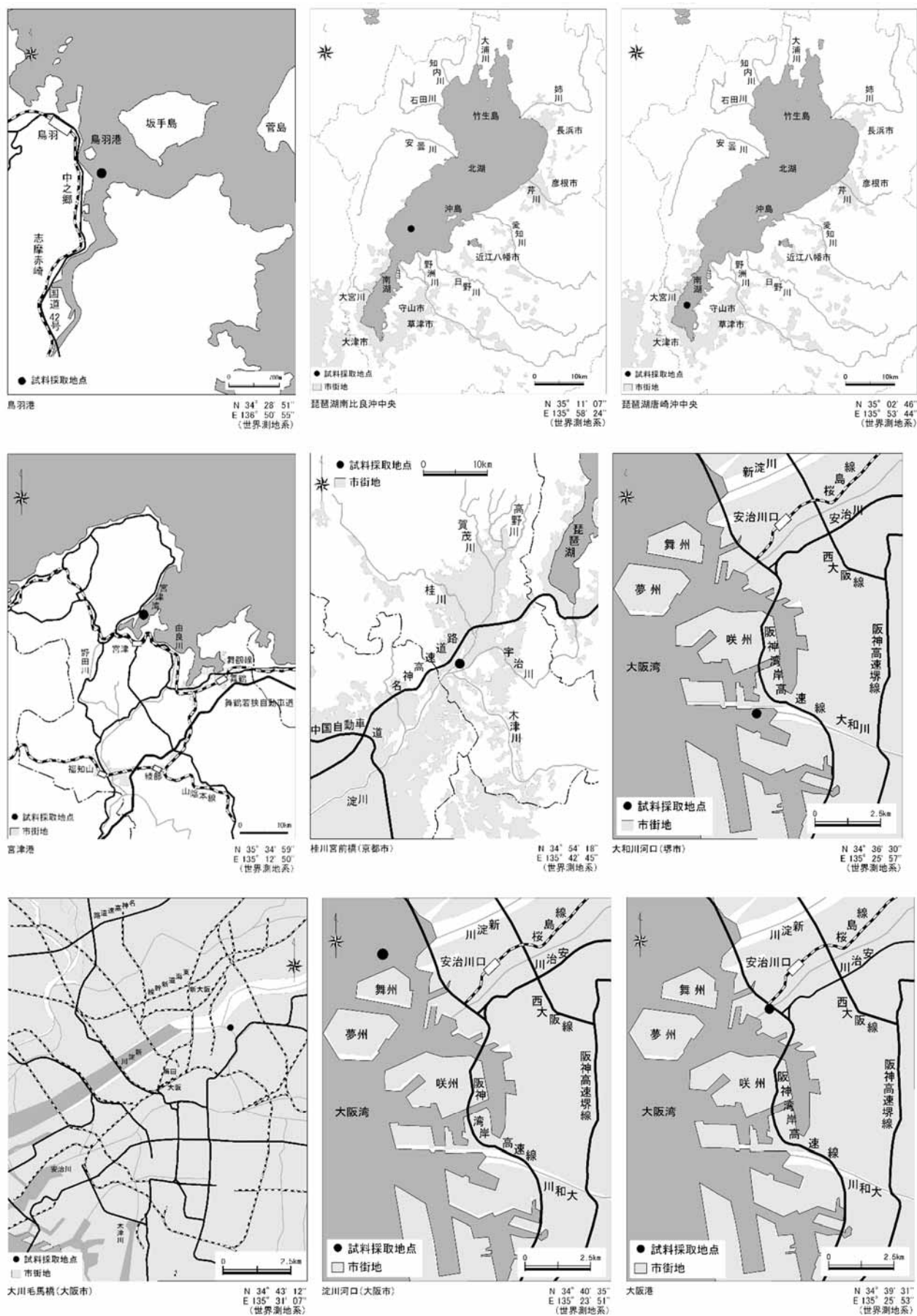
図 1-4 (4/7) 2023 年度モニタリング調査地点 (底質) 詳細
