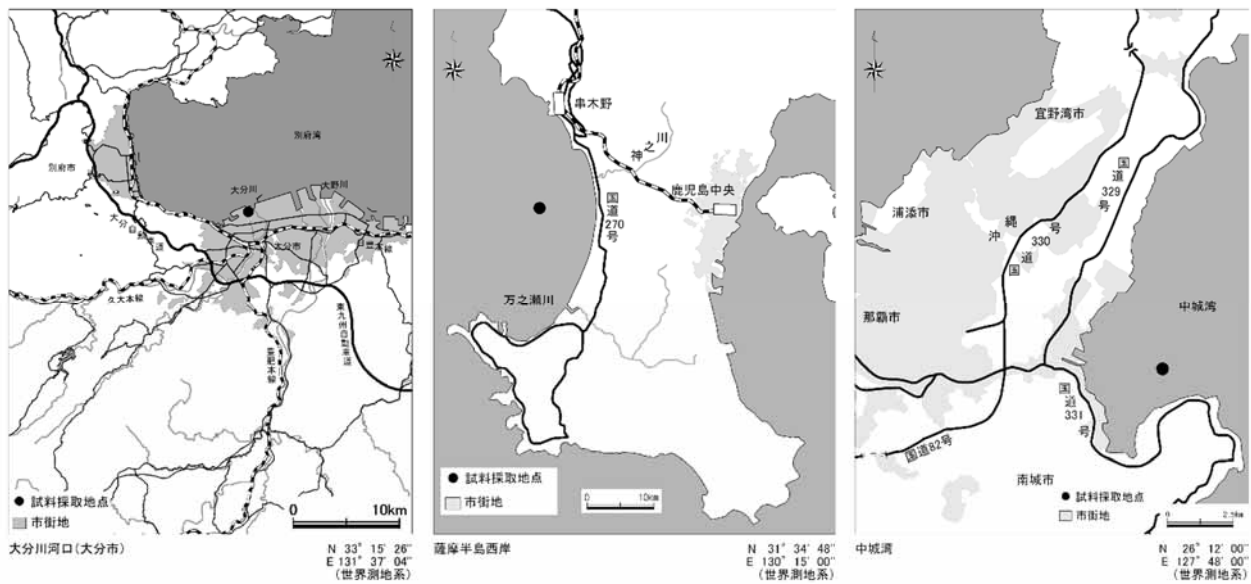
図 1-6 (3/3) 2023 年度モニタリング調査地点 (生物) 詳細
