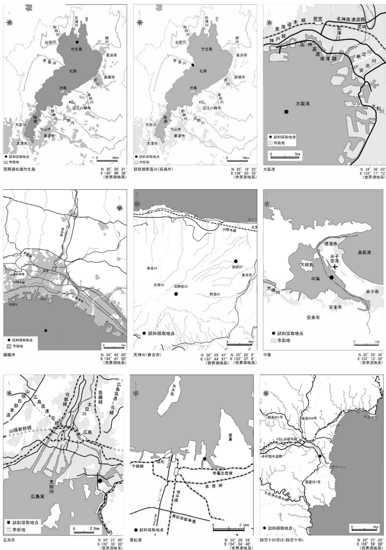
図 1-6 (2/3) 2023 年度モニタリング調査地点 (生物) 詳細
