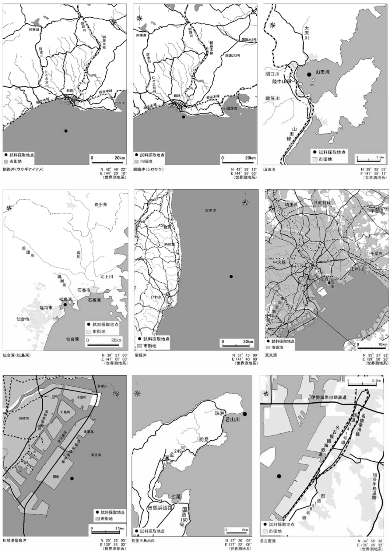
図 1-6 (1/3) 2023 年度モニタリング調査地点 (生物) 詳細
