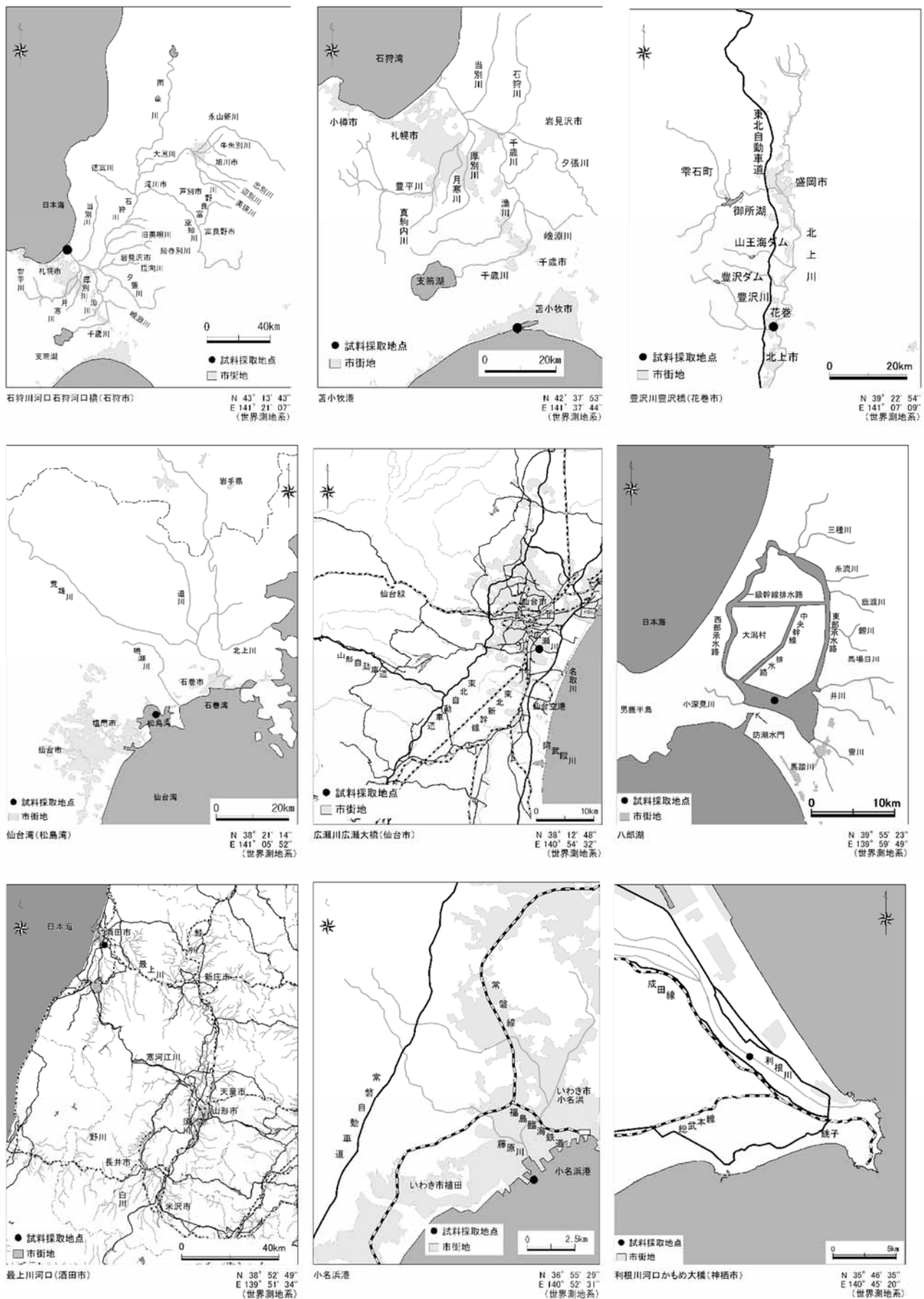
図 1-4 (1/7) 2023 年度モニタリング調査地点(底質) 詳細
