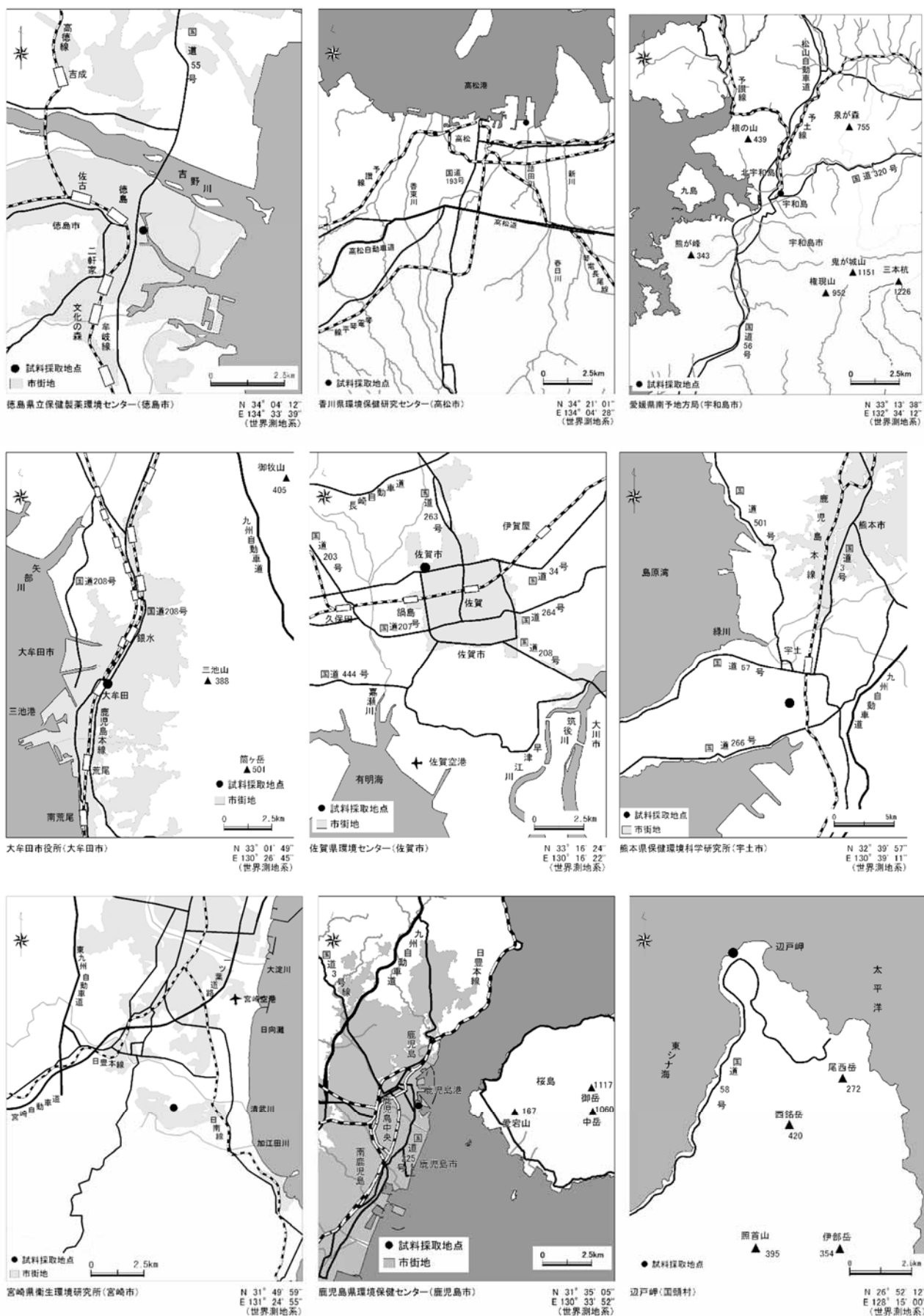
図 1-8 (4/4) 2023 年度モニタリング調査地点 (大気) 詳細
