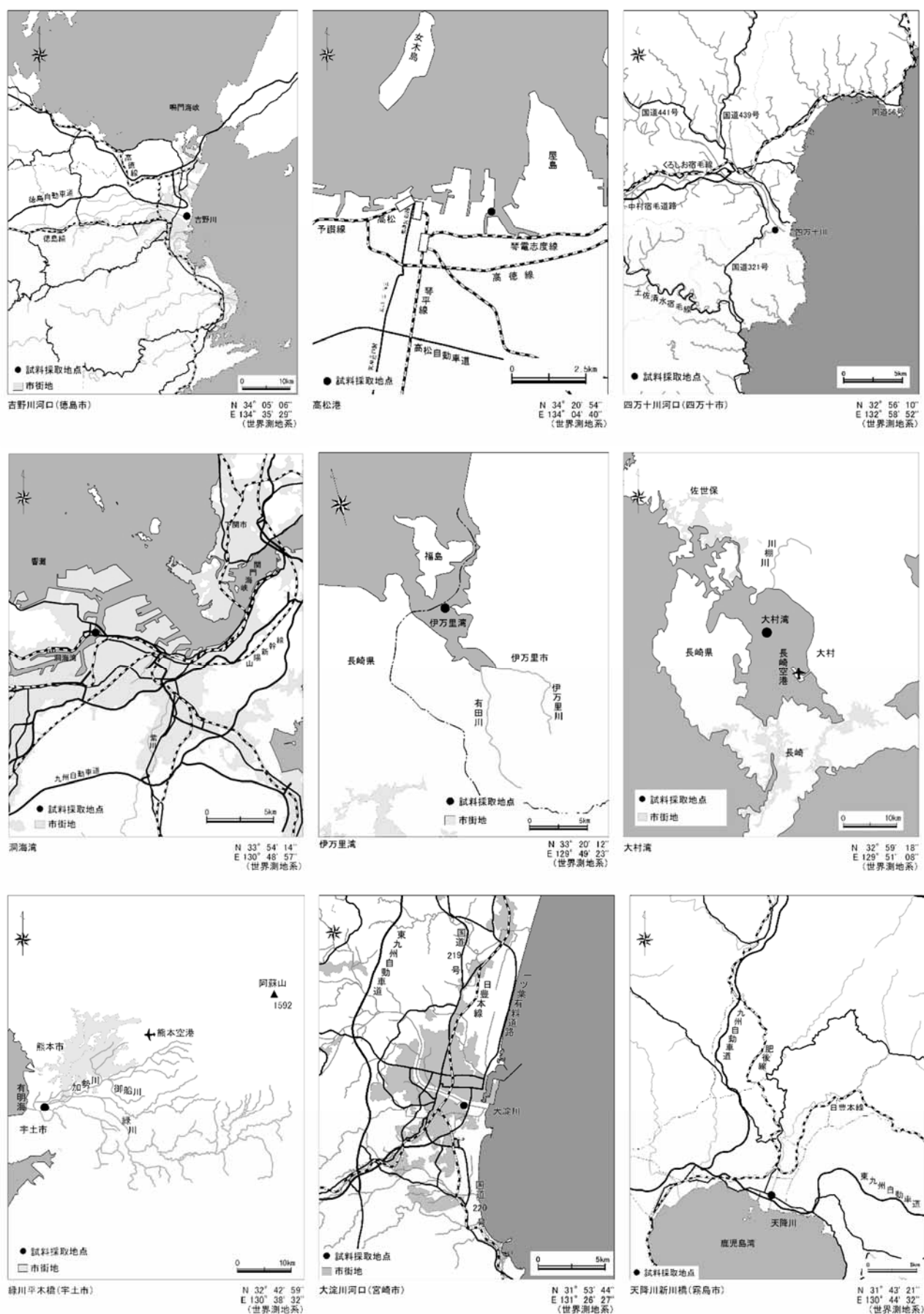
図 1-2 (5/6) 2023 年度モニタリング調査地点 (水質) 詳細
