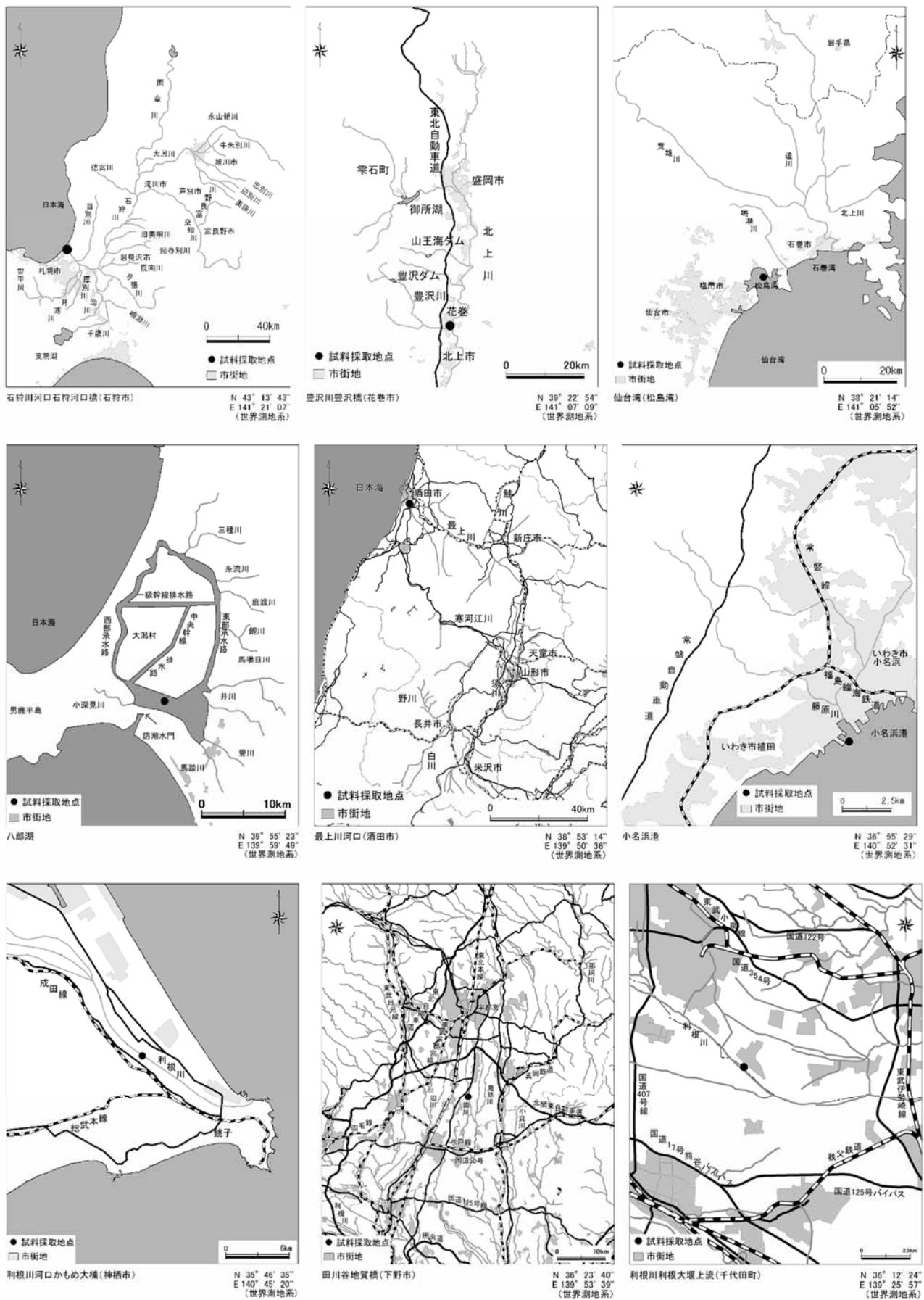
図 1-2 (1/6) 2023 年度モニタリング調査地点 (水質) 詳細
