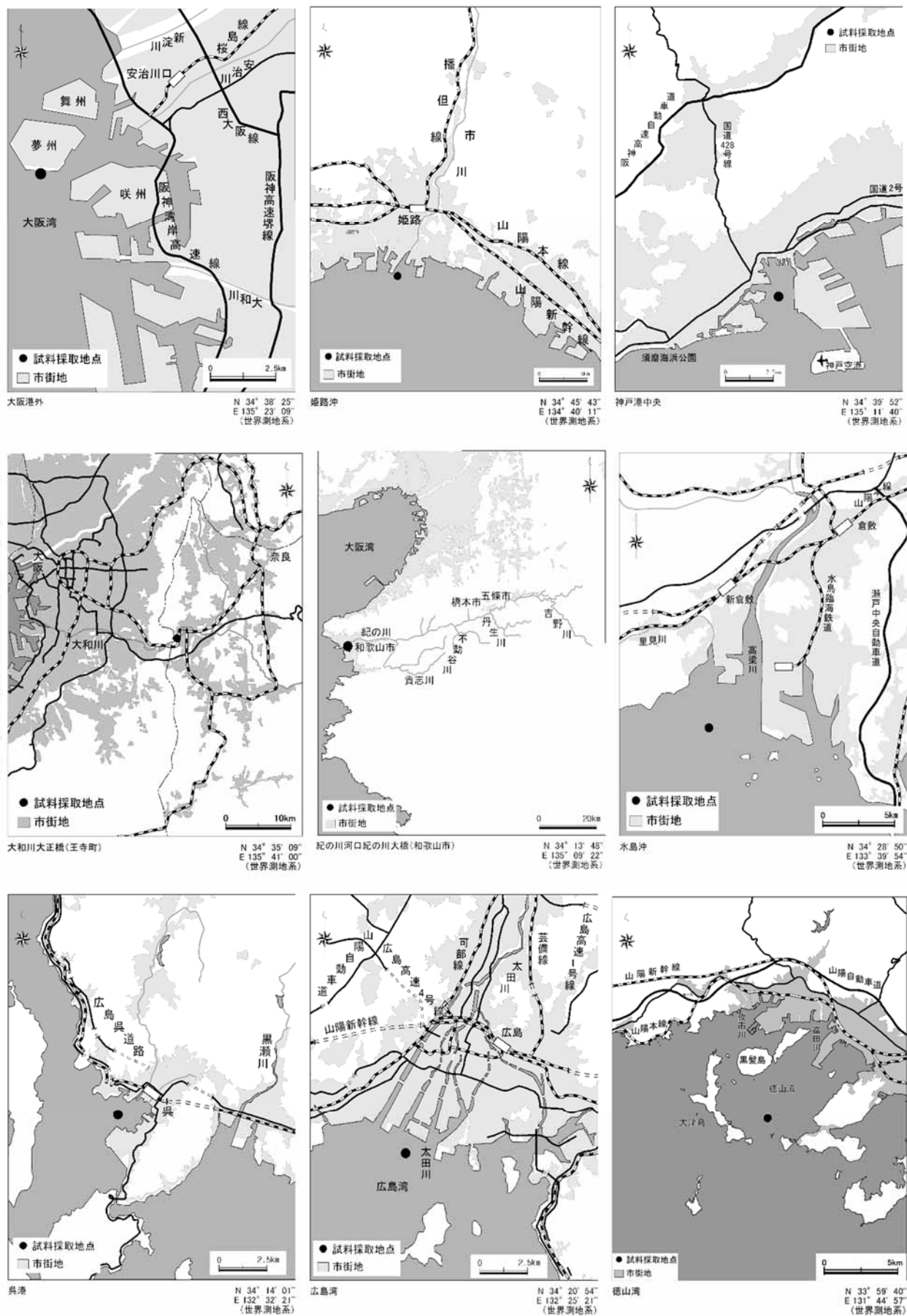
図 1-4 (5/7) 2023 年度モニタリング調査地点(底質) 詳細
