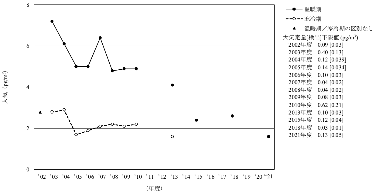
[6-2] p,p' -DDE
