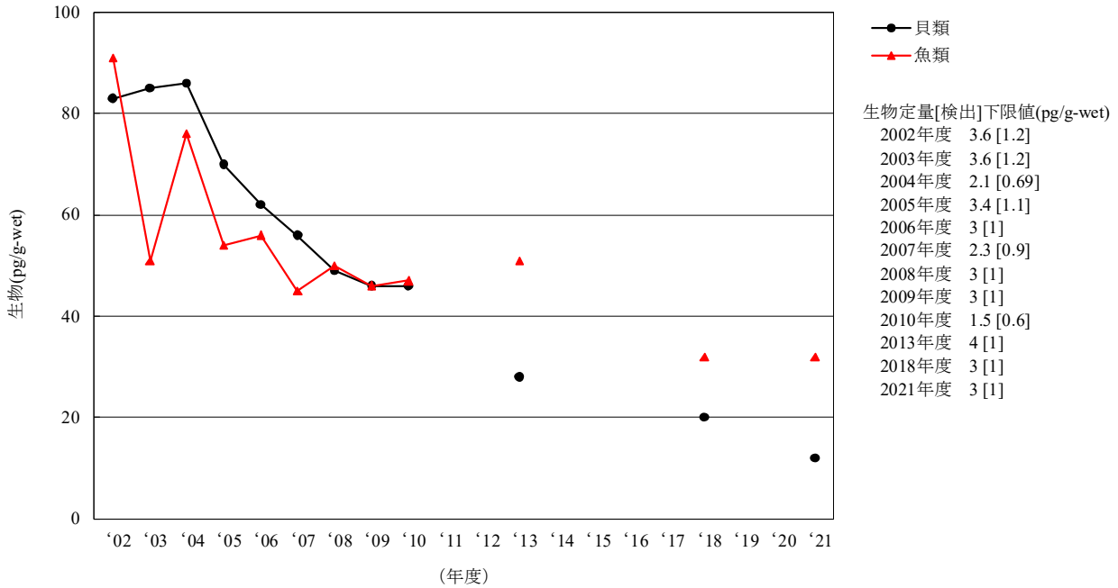
[6-5] o,p' -DDE
