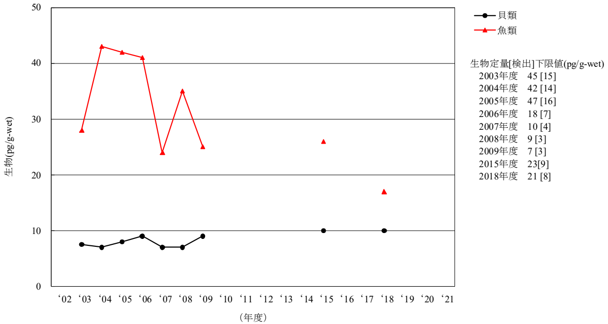
[9-1] Parlar-26
