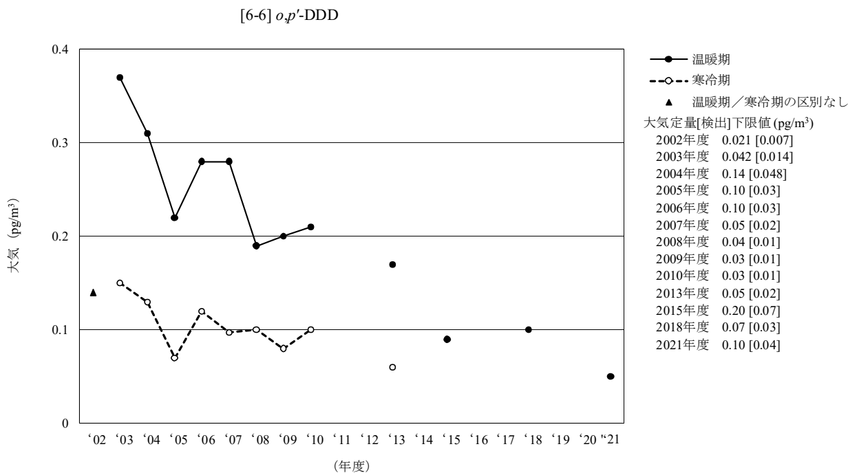
図 3-6-6-4 o,p' -DDD の大気の大気経年変化 (幾何平均値)
