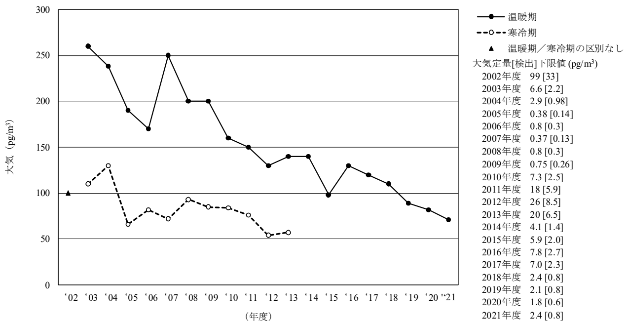
図 3-1-4 総 PCB の大気の大気経年変化（幾何平均値）
