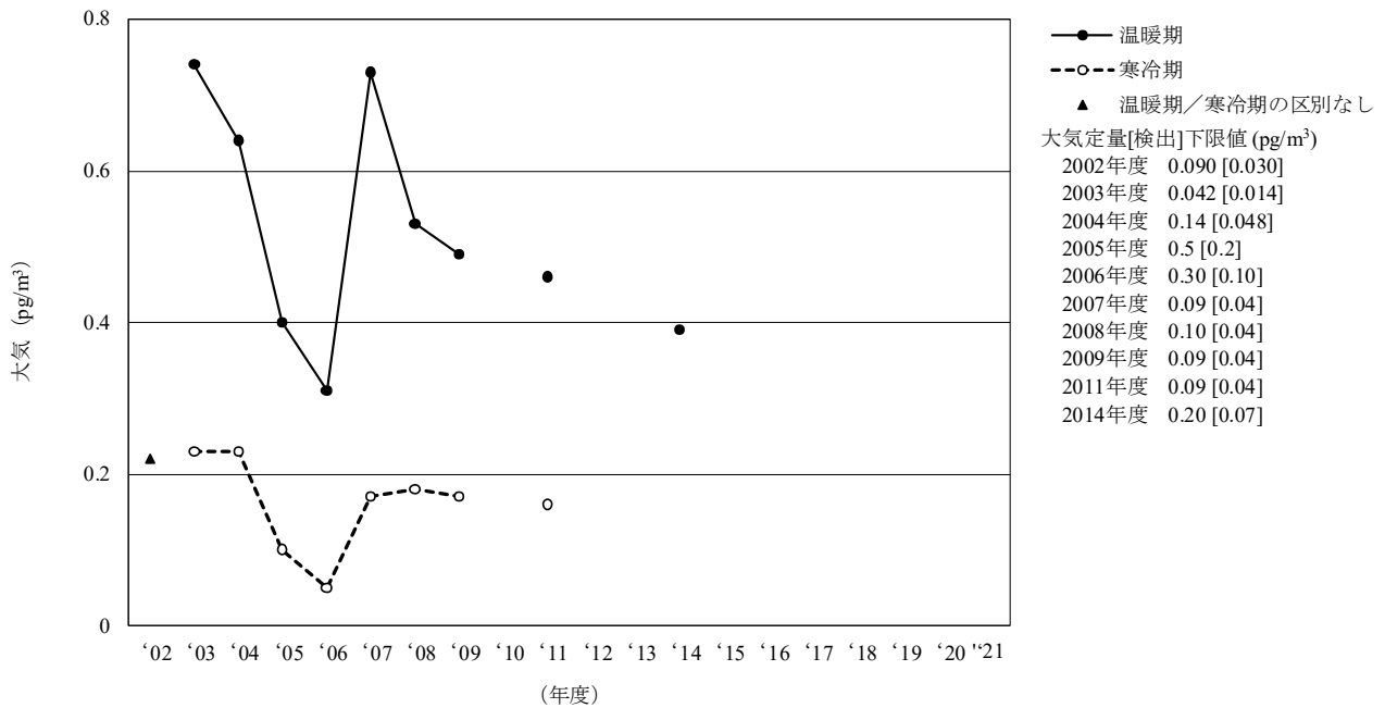
[5] エンドリン
