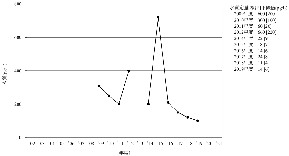
図3-14-7-1 デカブロモジフェニルエーテルの水質の経年変化（幾何平均値）
