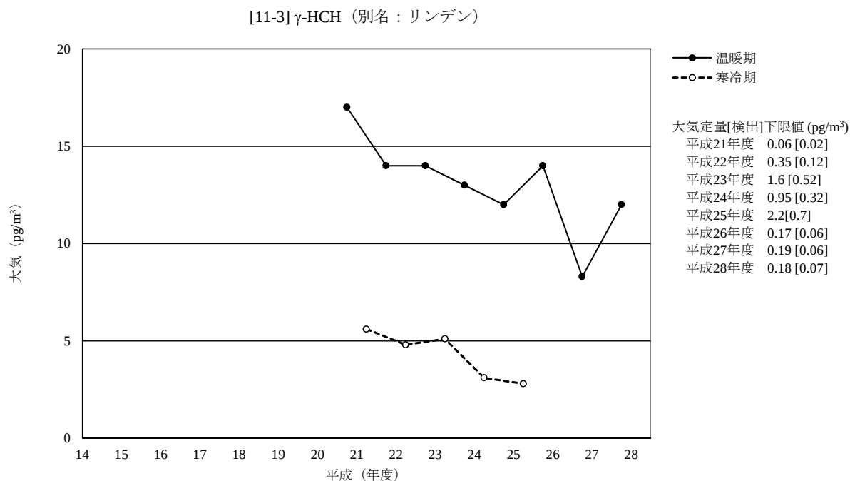
図 3-11-3-4 \gamma -HCH (別名：リンデン) の大気の経年変化 (幾何平均値)
