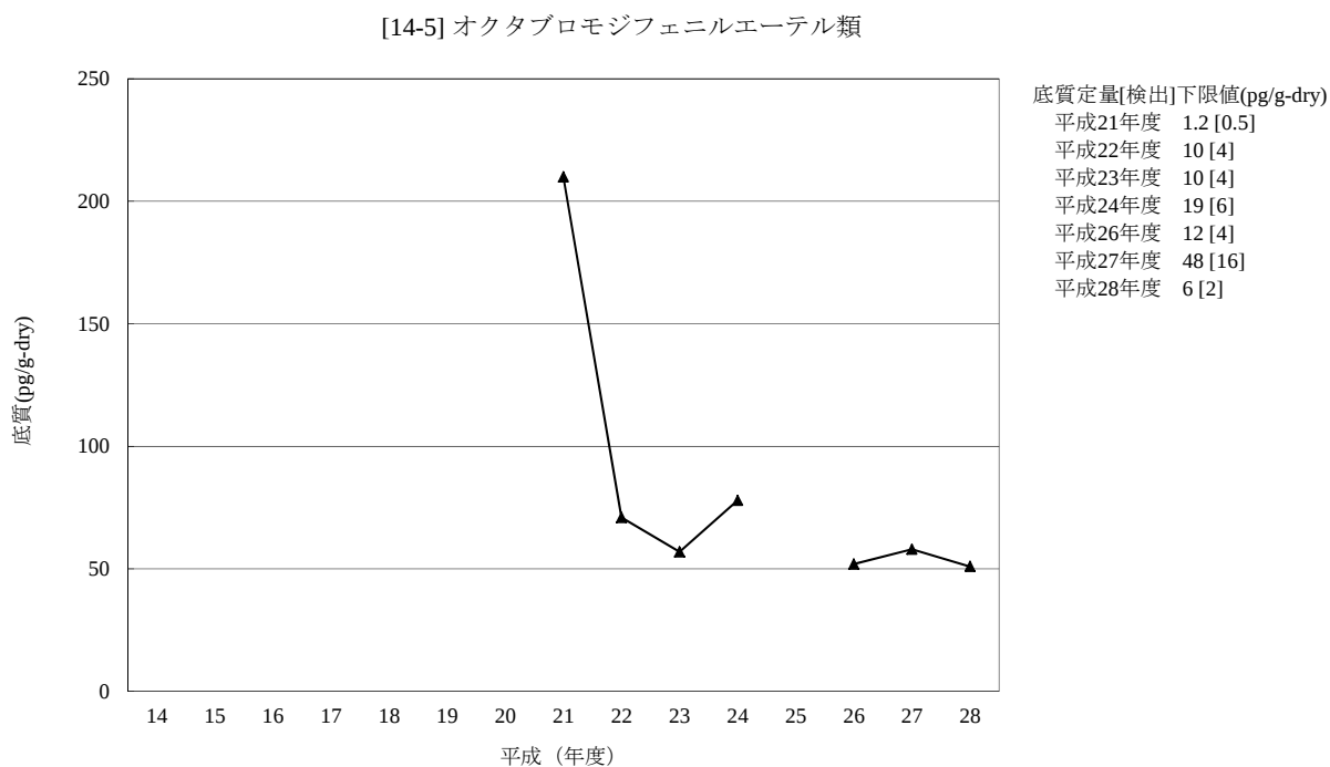
図 3-14-5-2 オクタブロモジフェニルエーテル類の底質の経年変化 (幾何平均値)
