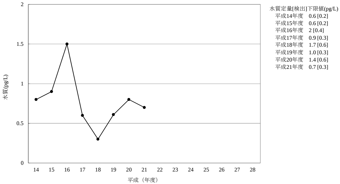
[3] アルドリン
