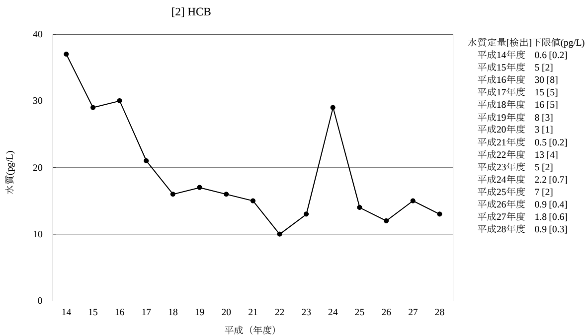
図 3-2-1 HCB の水質の経年変化（幾何平均値）
