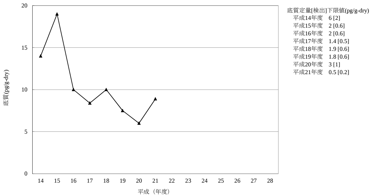
[3] アルドリン
