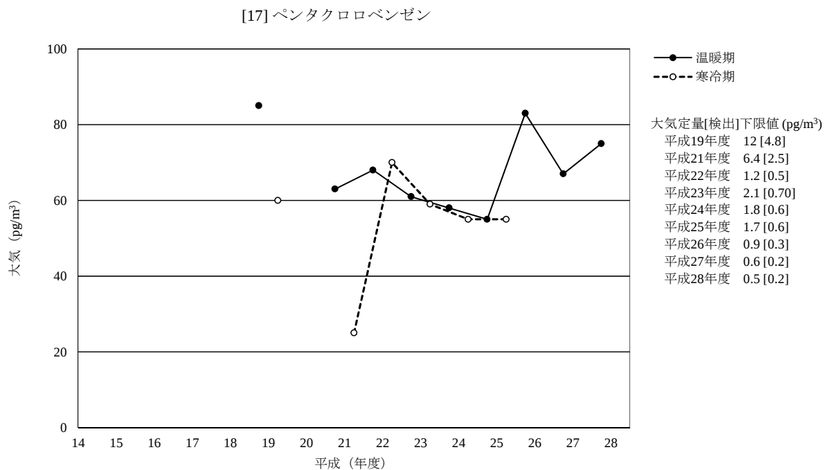
図 3-17-3 ペンタクロロベンゼンの大気の経年変化 (幾何平均値)
