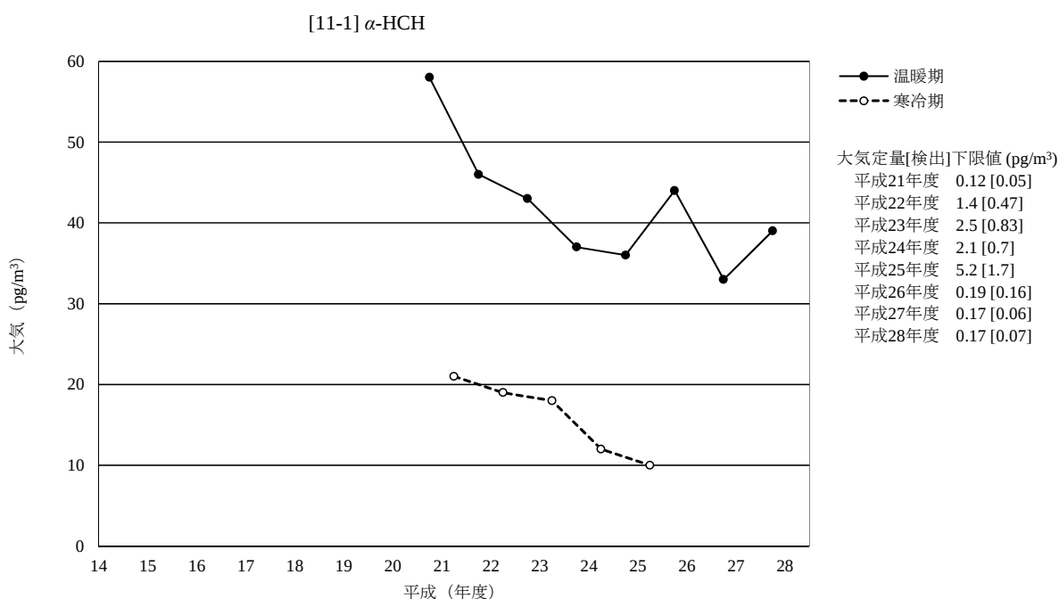
図 3-11-1-4 \alpha -HCH の大気の経年変化 (幾何平均値)
