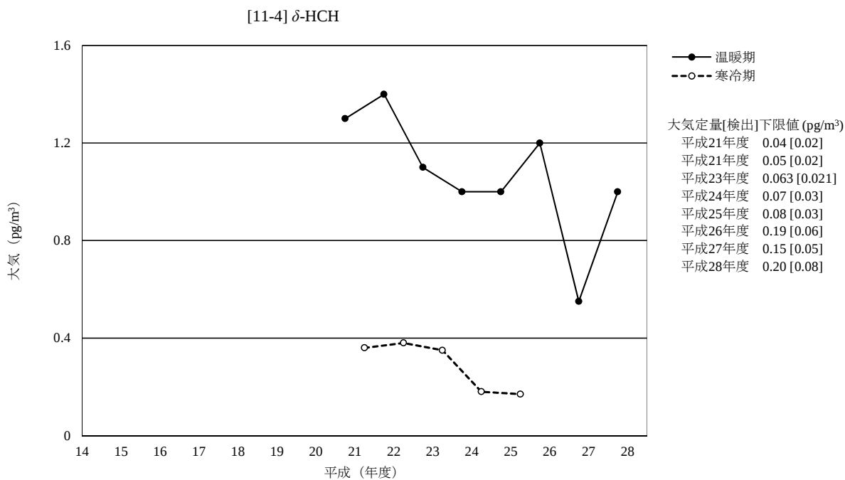
図 3-11-4-4 \delta -HCH の大気の経年変化 (幾何平均値)
