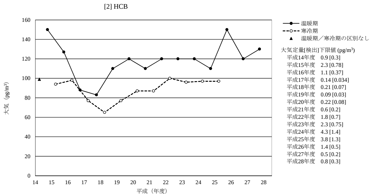
図 3-2-4 HCB の大気の経年変化 (幾何平均値)
