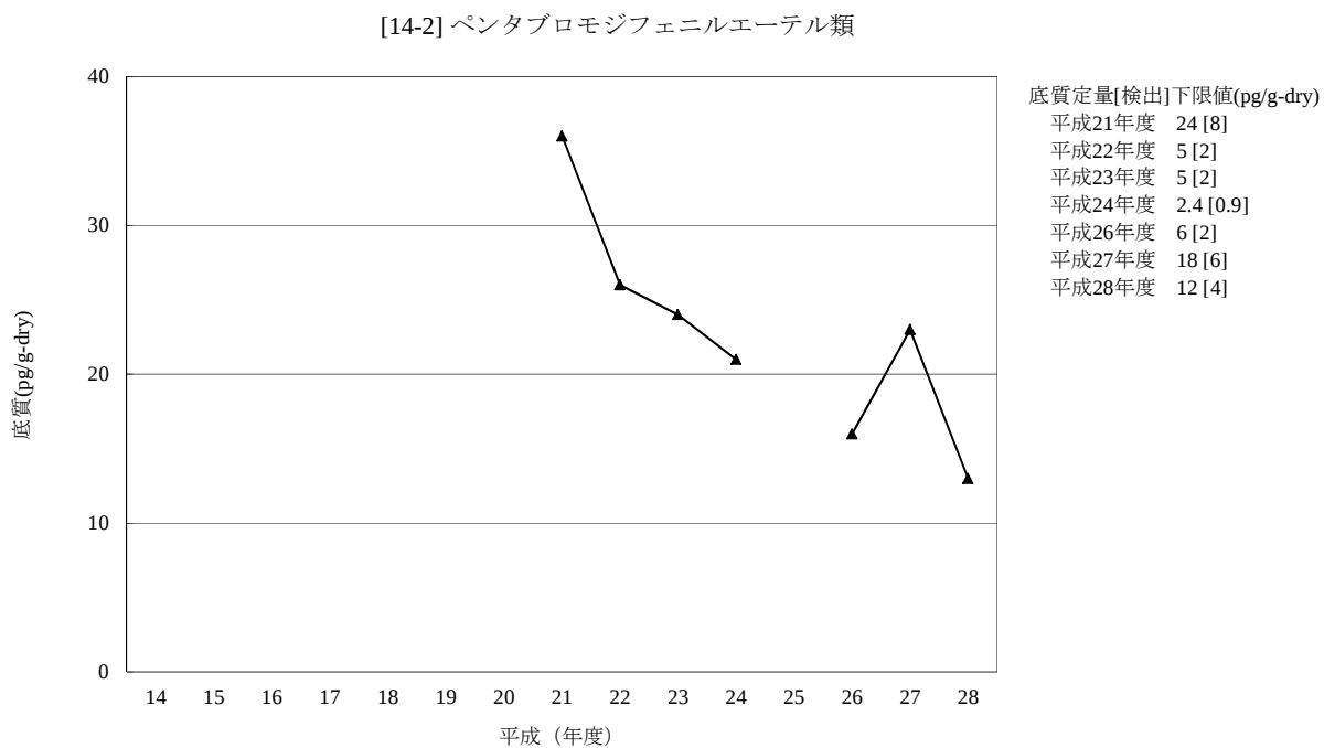
図 3-14-2-2 ペンタブロモジフェニルエーテル類の底質の経年変化 (幾何平均値)
