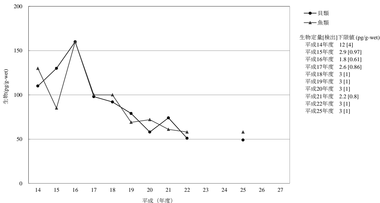
[6-4] o,p' -DDT
