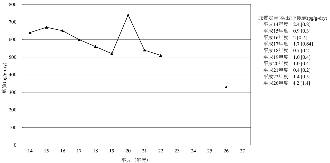
[6-3] p,p' -DDD
