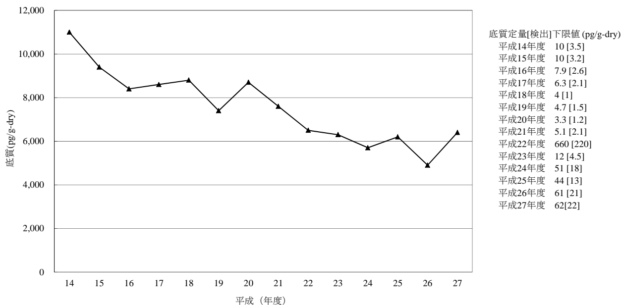
[1] 総PCB
