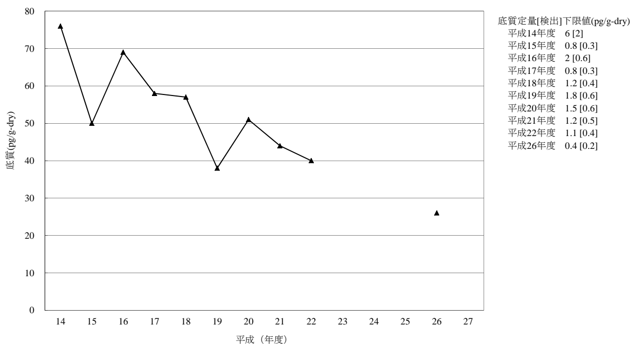
[6-4] o,p' -DDT
