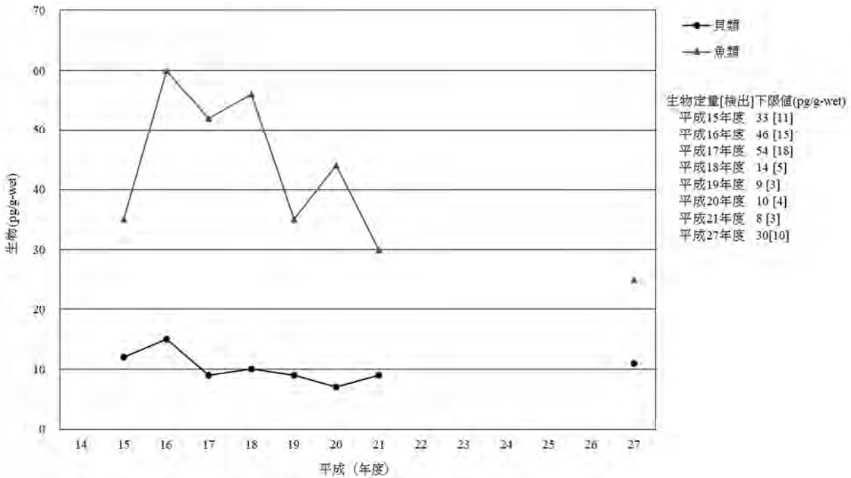
[9-2] Parlar-50
