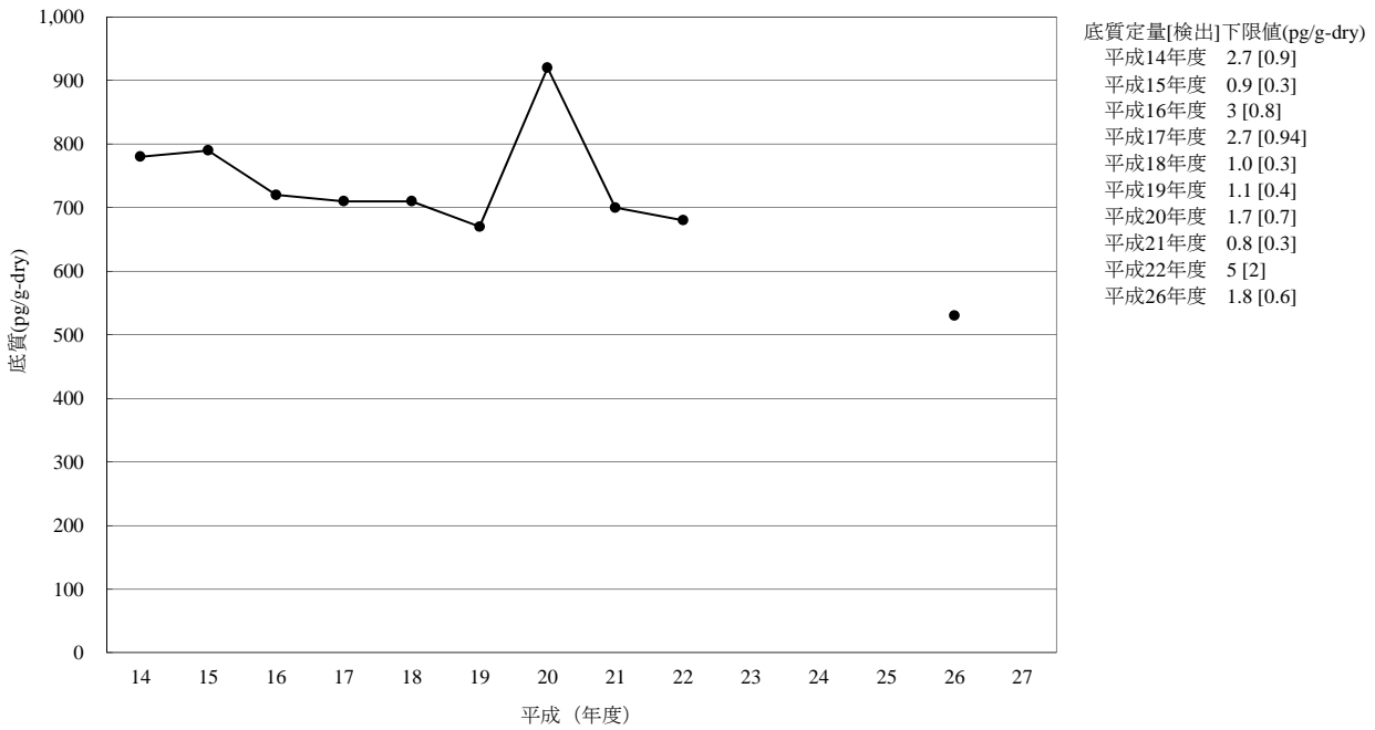
[6-2] p,p' -DDE
