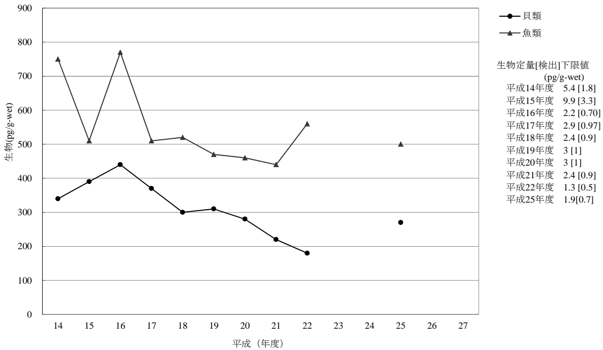
[6-3] p,p' -DDD
