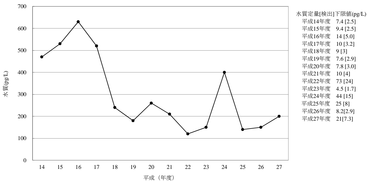
[1] 総PCB
