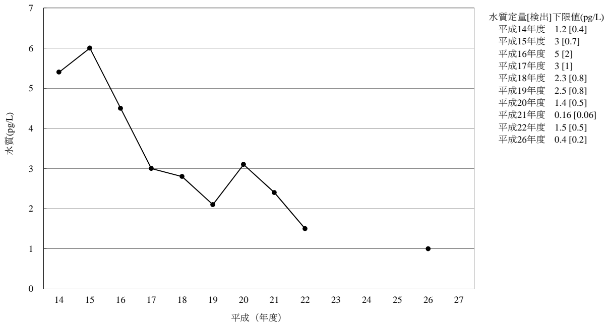
[6-4] o,p' -DDT
