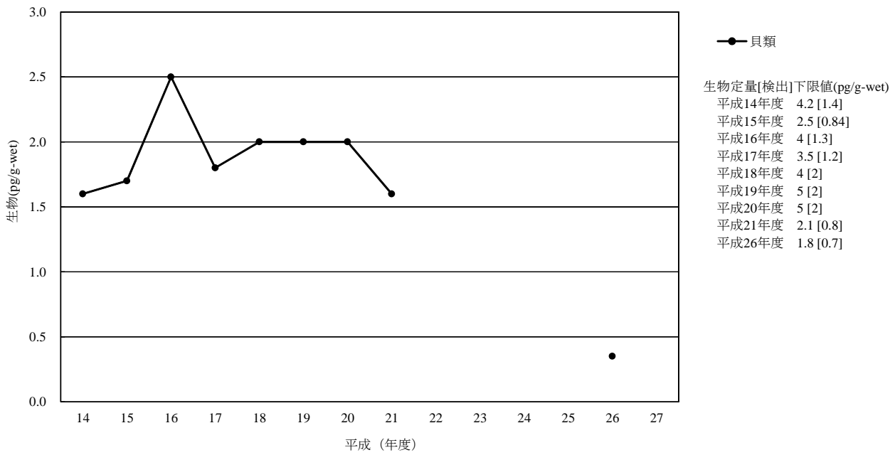
[3] アルドリノ
