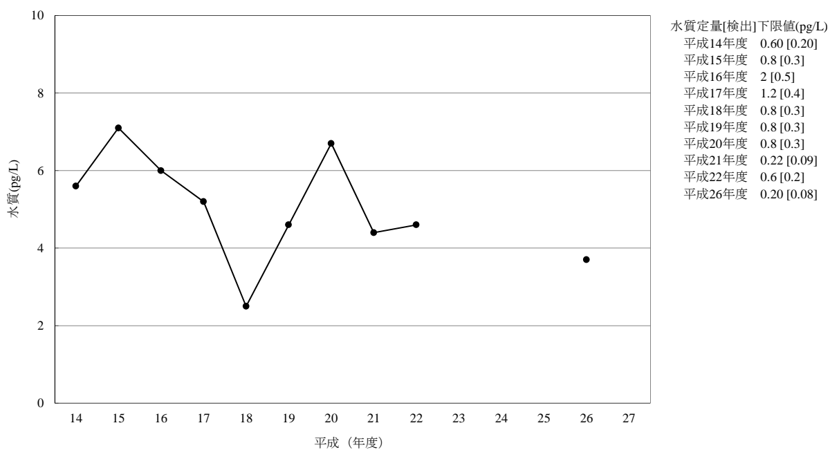
[6-6] o,p' -DDD
