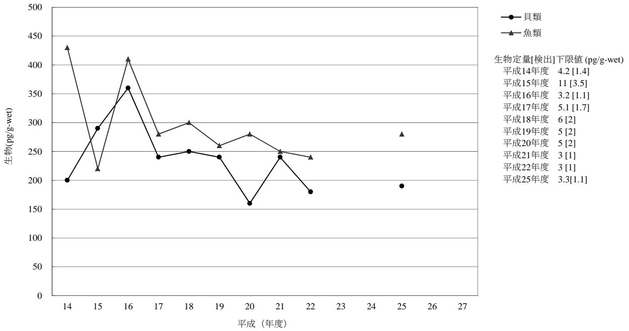
[6-1] p,p' -DDT
