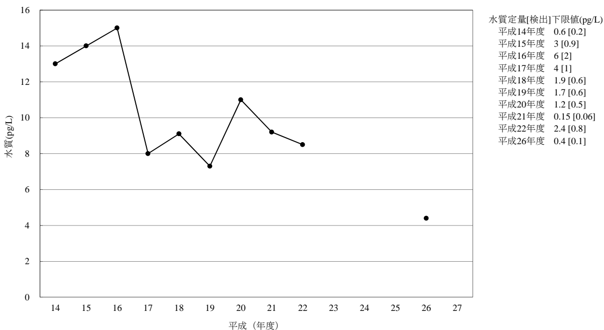
[6-1] p,p' -DDT
