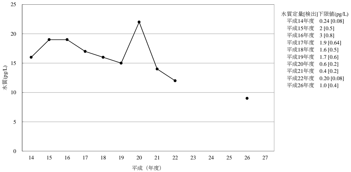
[6-3] p,p' -DDD
