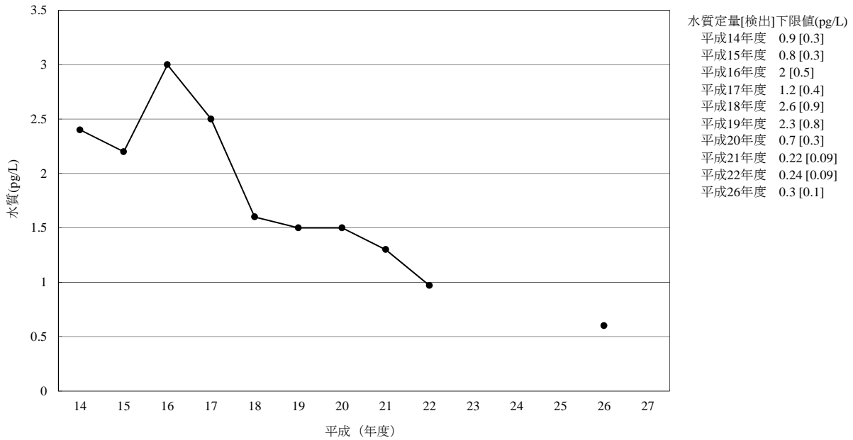
[6-5] o,p' -DDE
