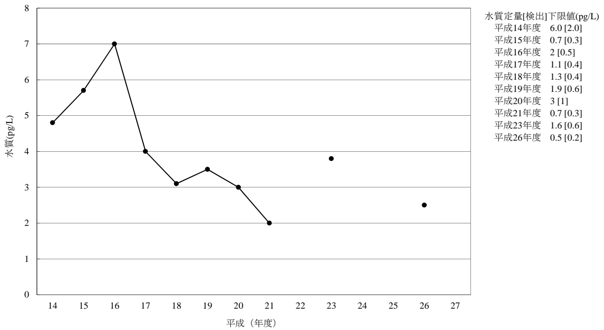
[5] エンドリン
