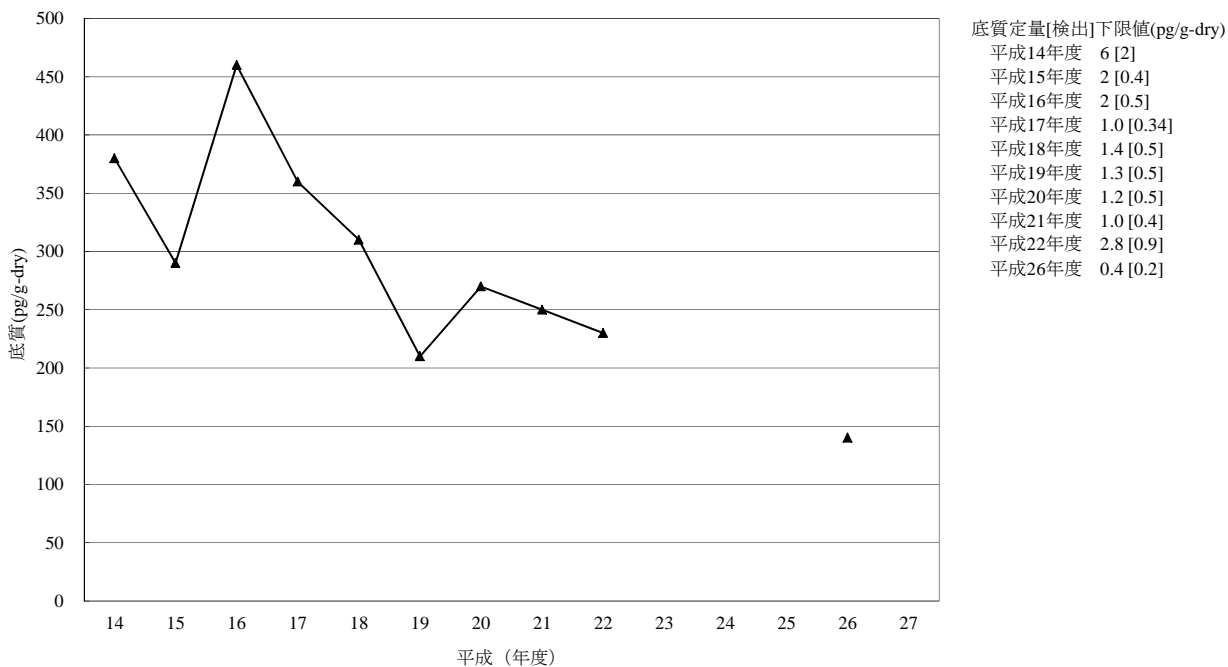
[6-1] p,p' -DDT
