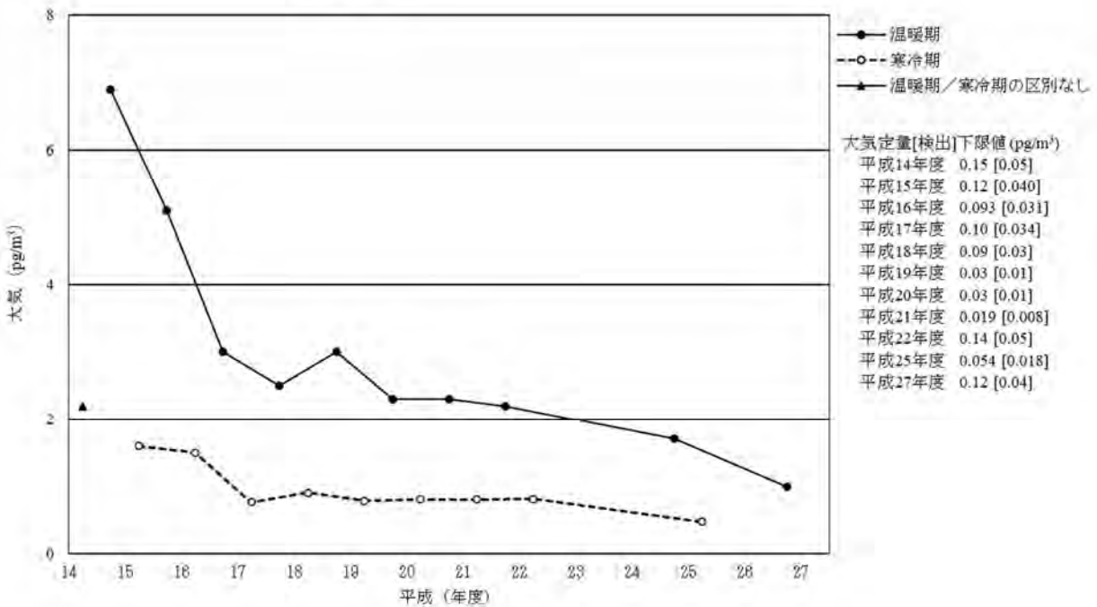
[6-4] o,p' -DDT
