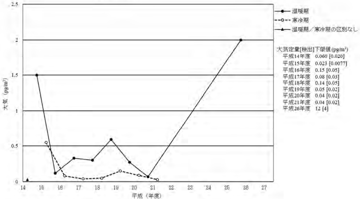
[3] アルドリノ
