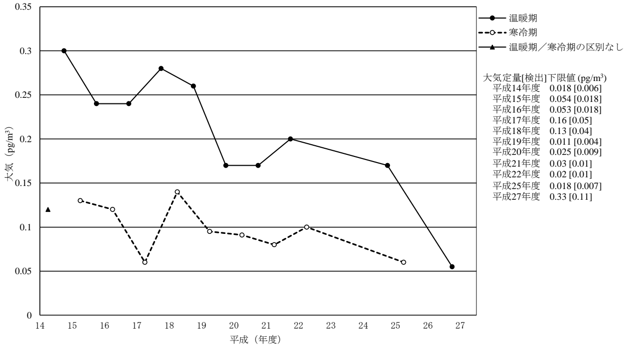
[6-3] p,p' -DDD
