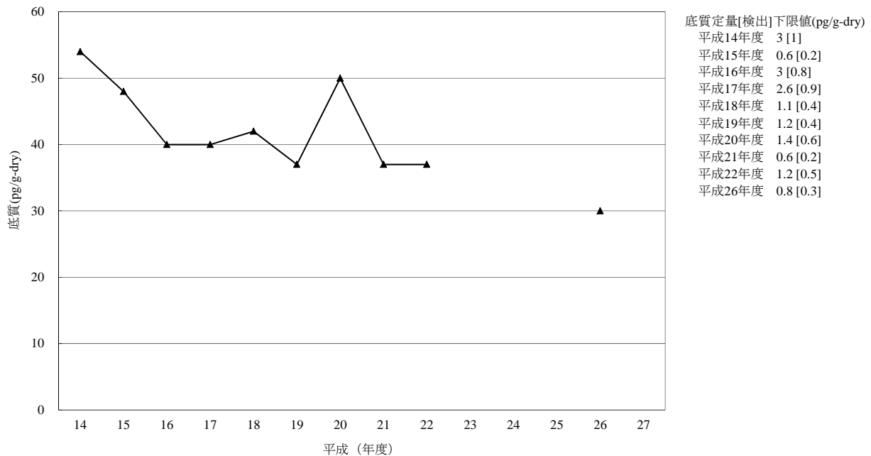
[6-5] o,p' -DDE
