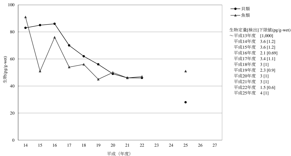
[6-5] o,p' -DDE
