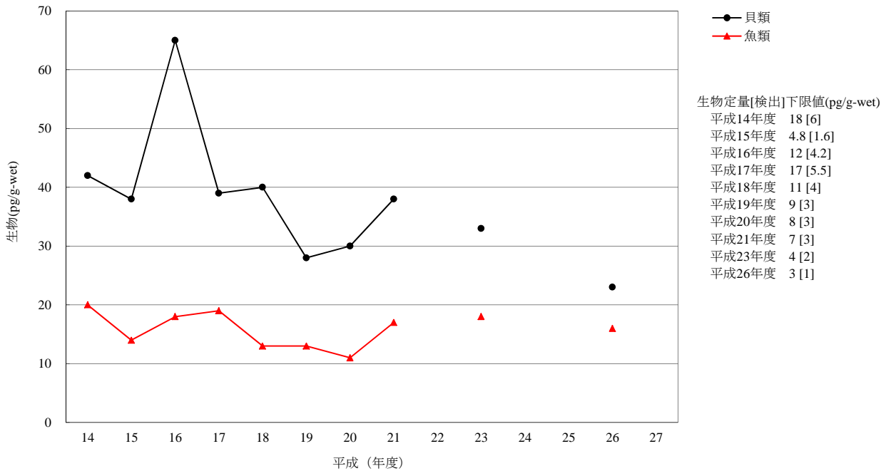
[5] エンドリン
