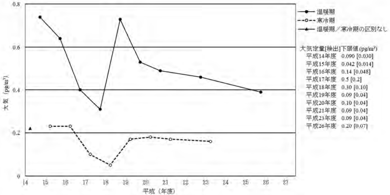
[5] エンドリン
