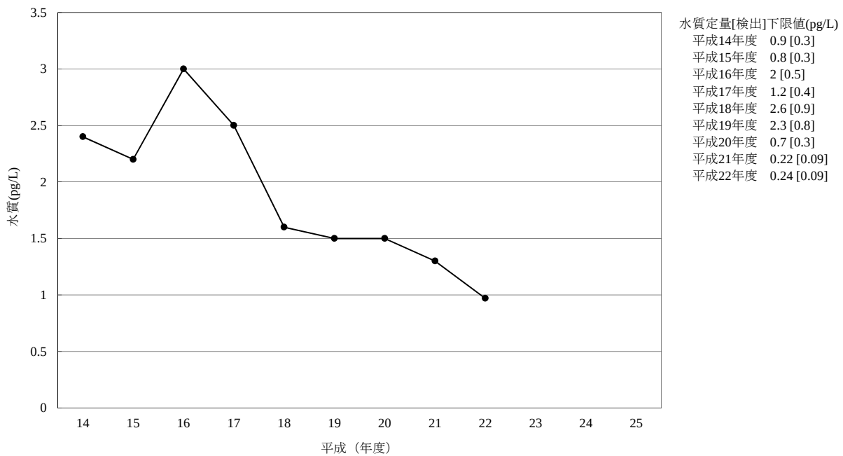
[6-5] o,p' -DDE
