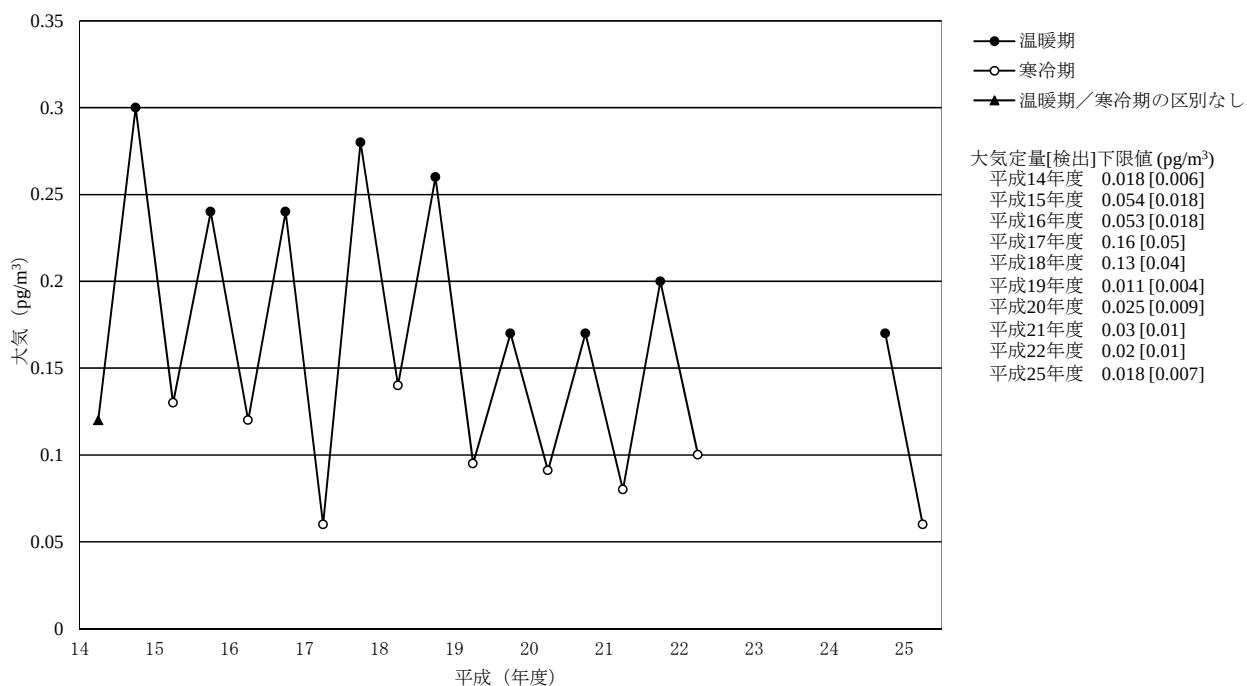
[6-3] p,p' -DDD
