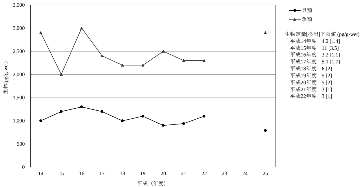
[6-2] p,p' -DDE
