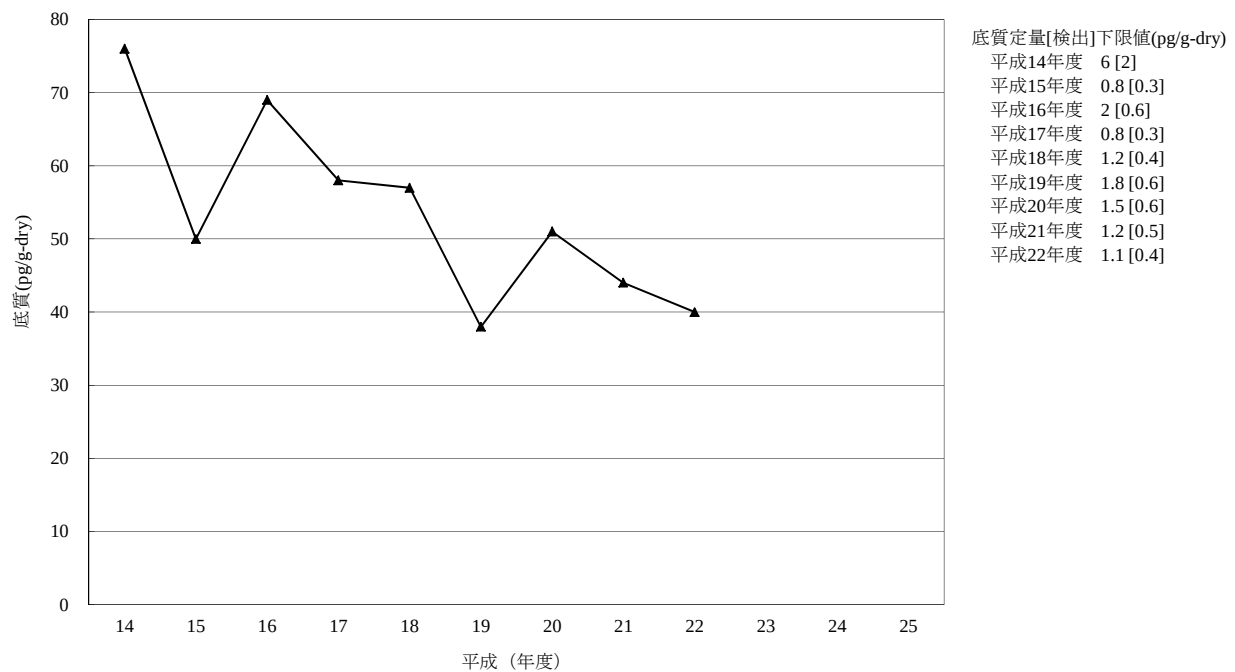
[6-4] o,p' -DDT
