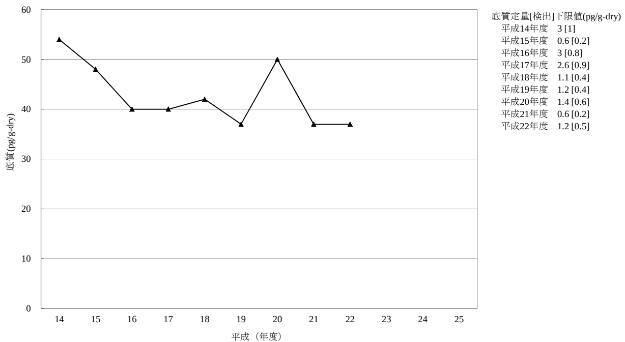
[6-5] o,p' -DDE
