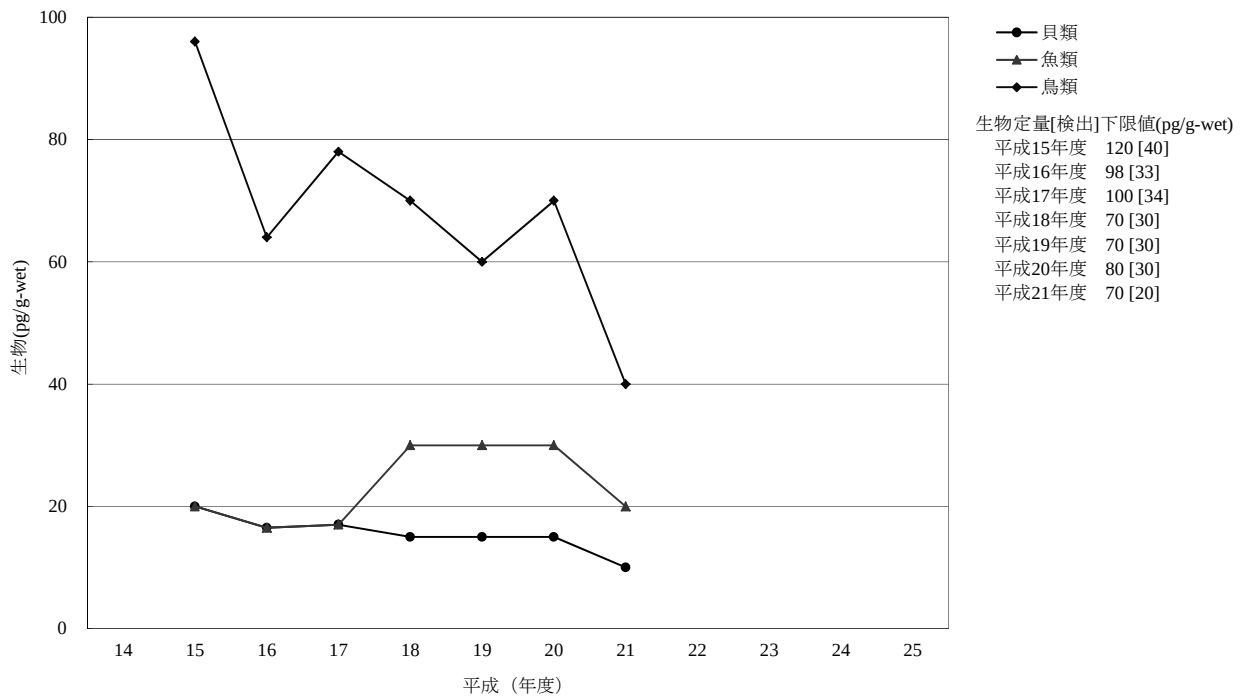
[9-3] Parlar-62
