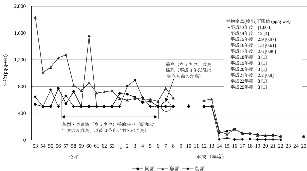
[6-4] o,p' -DDT
