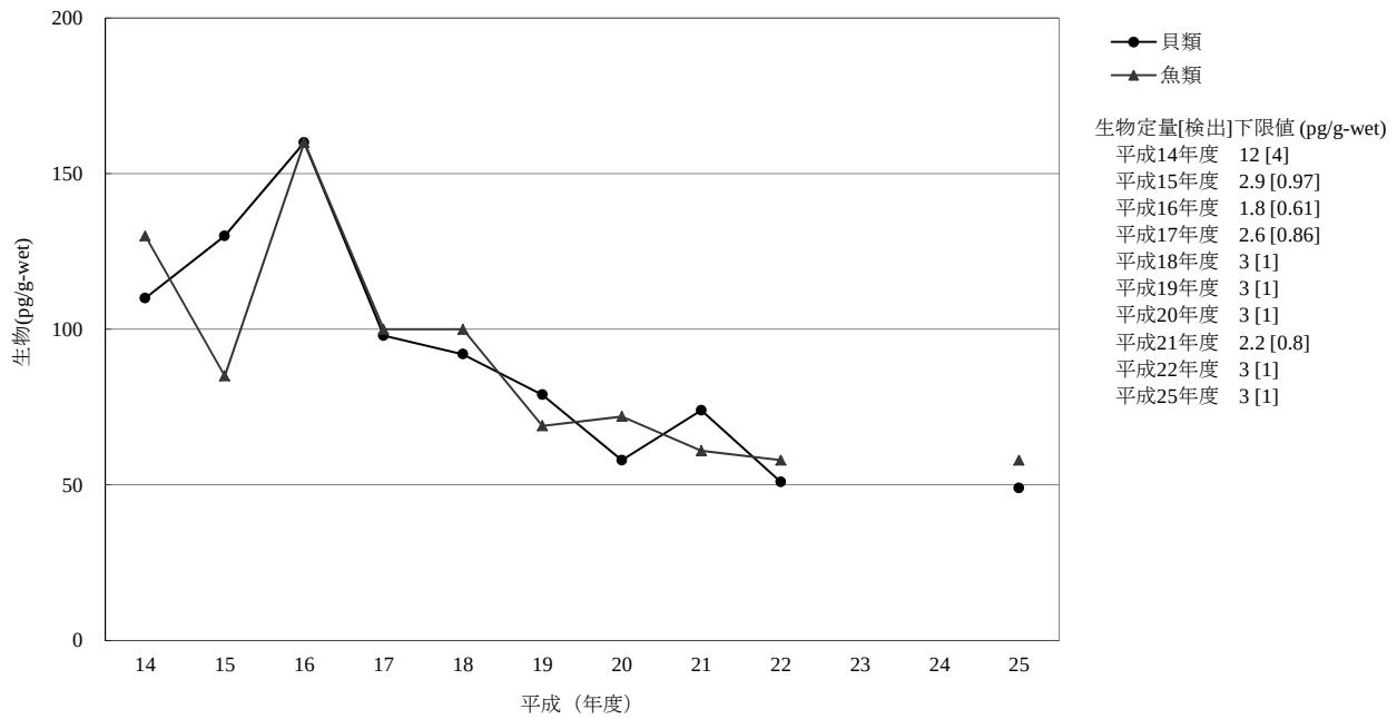
[6-4] o,p' -DDT
