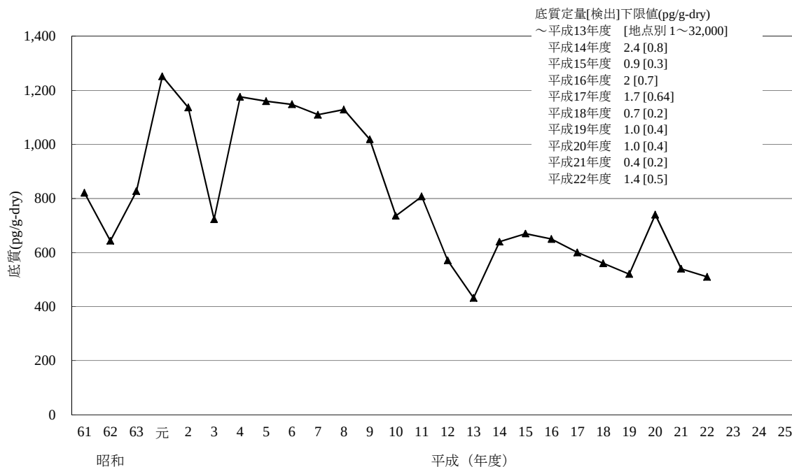
[6-3] p,p' -DDD
