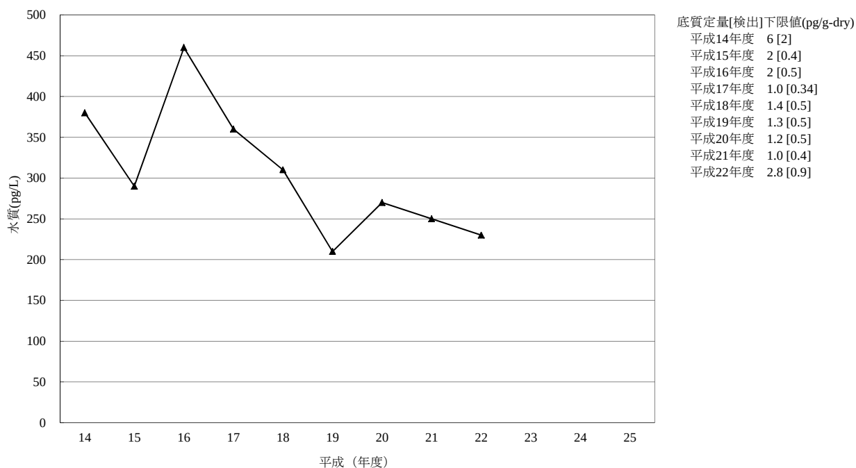
[6-1] p,p' -DDT
