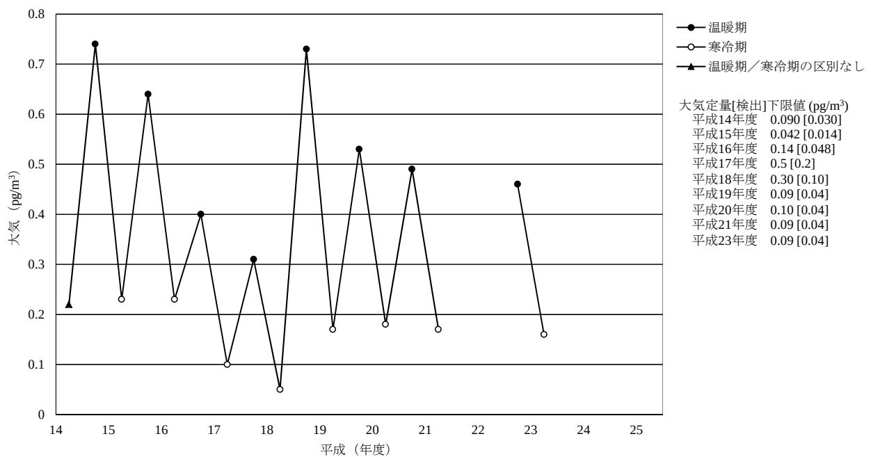
[5] エンドリン
