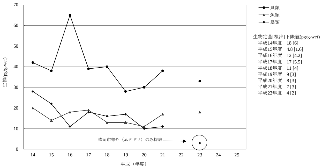
[5] エンドリン
