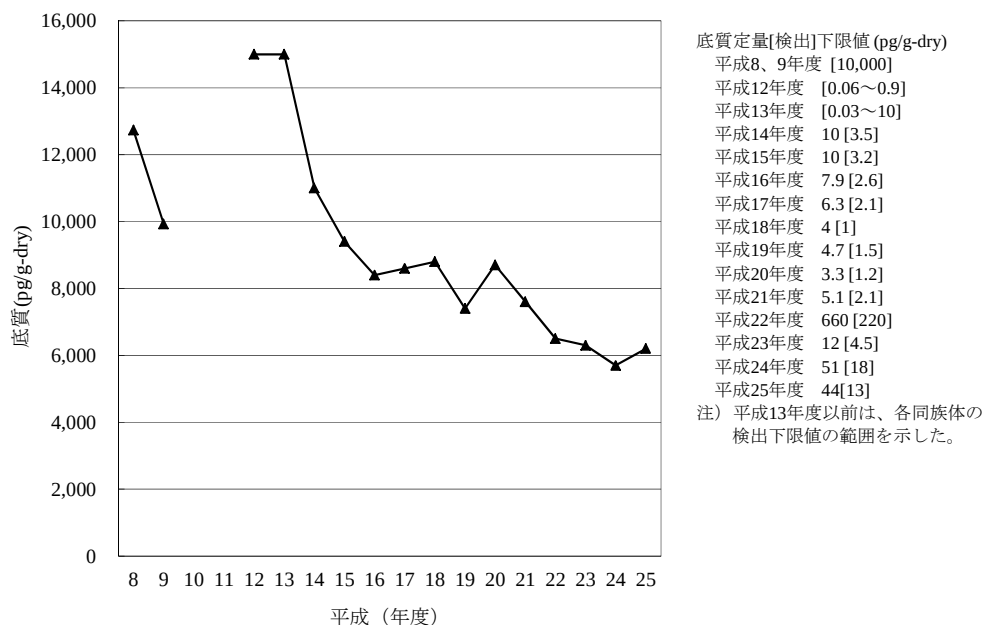
[1] 総PCB
