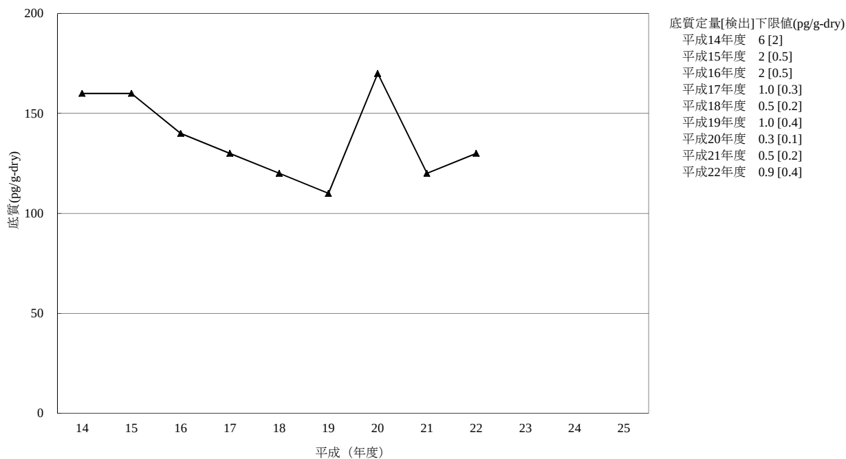
[6-6] o,p' -DDD
