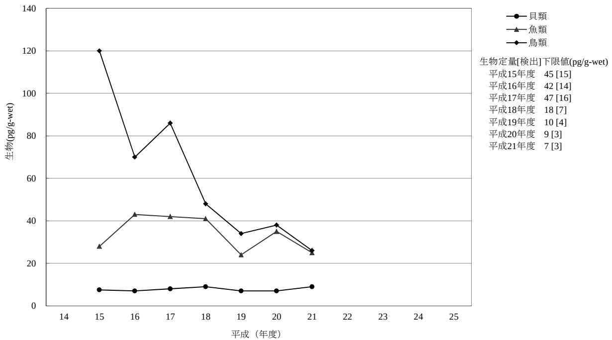
[9-1] Parlar-26
