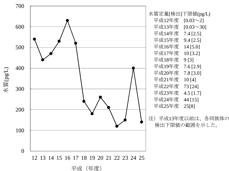
[1] 総PCB
