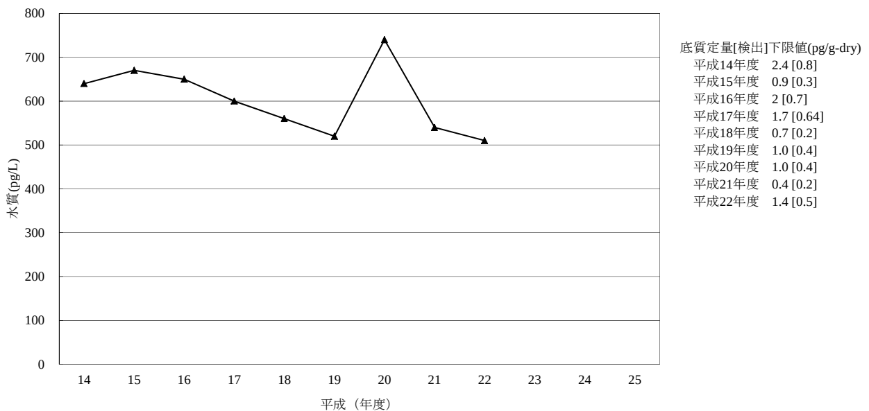
[6-3] p,p' -DDD
