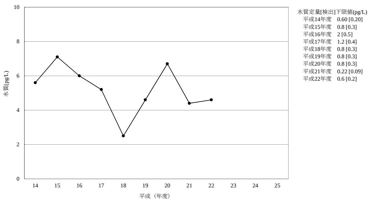
[6-6] o,p' -DDD
