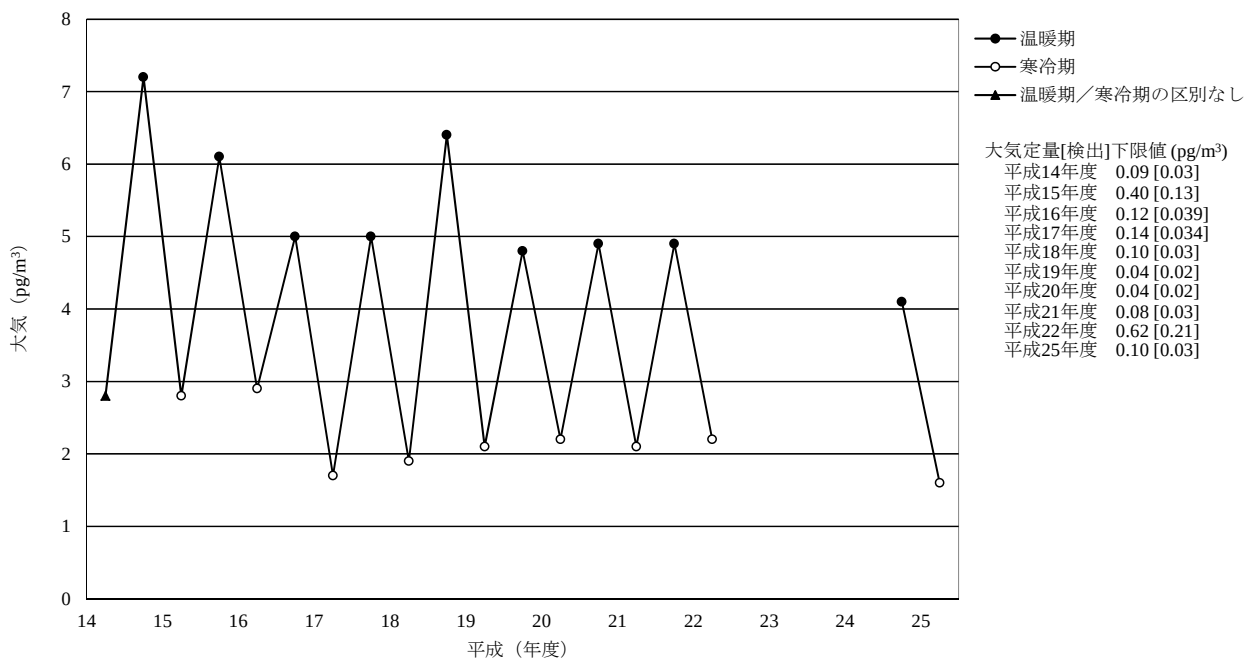
[6-2] p,p' -DDE
