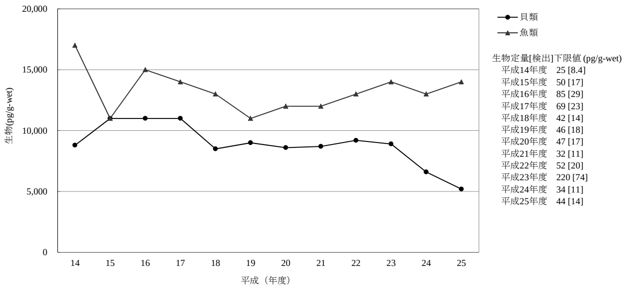
[1] 総PCB
