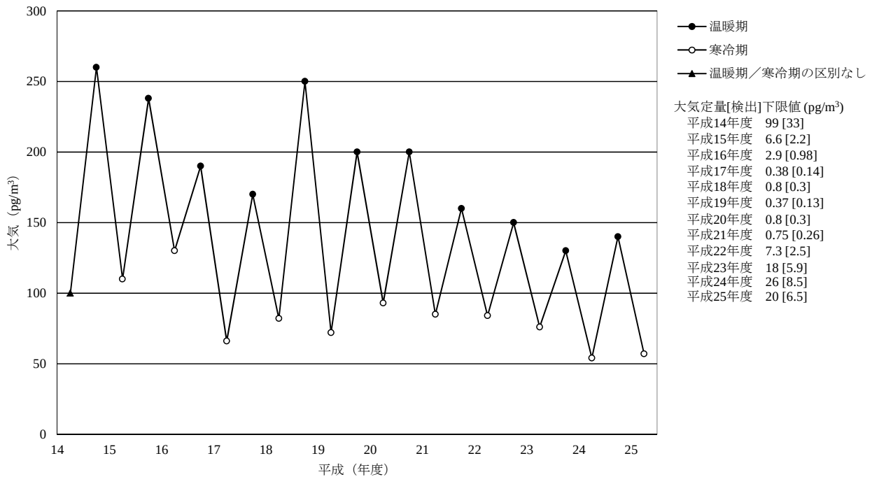
[1] 総PCB
