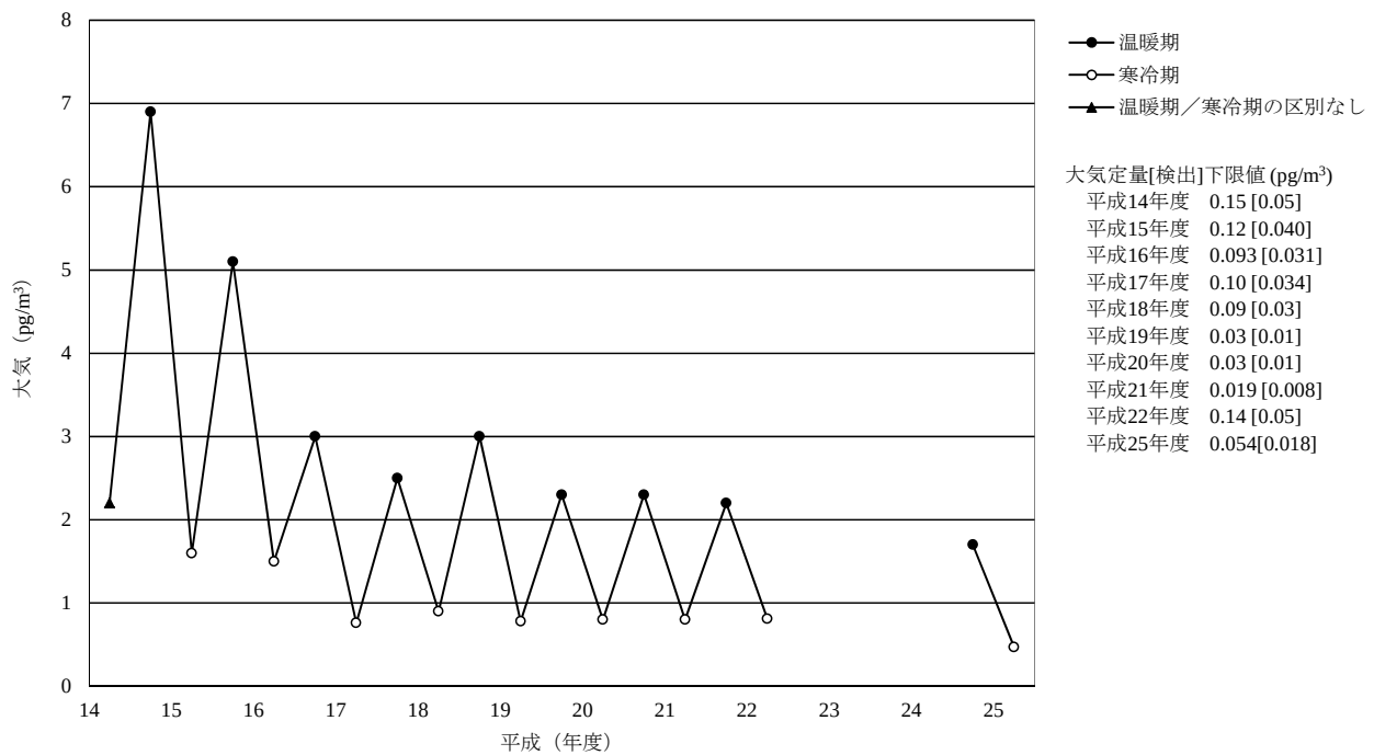
[6-4] o,p' -DDT
