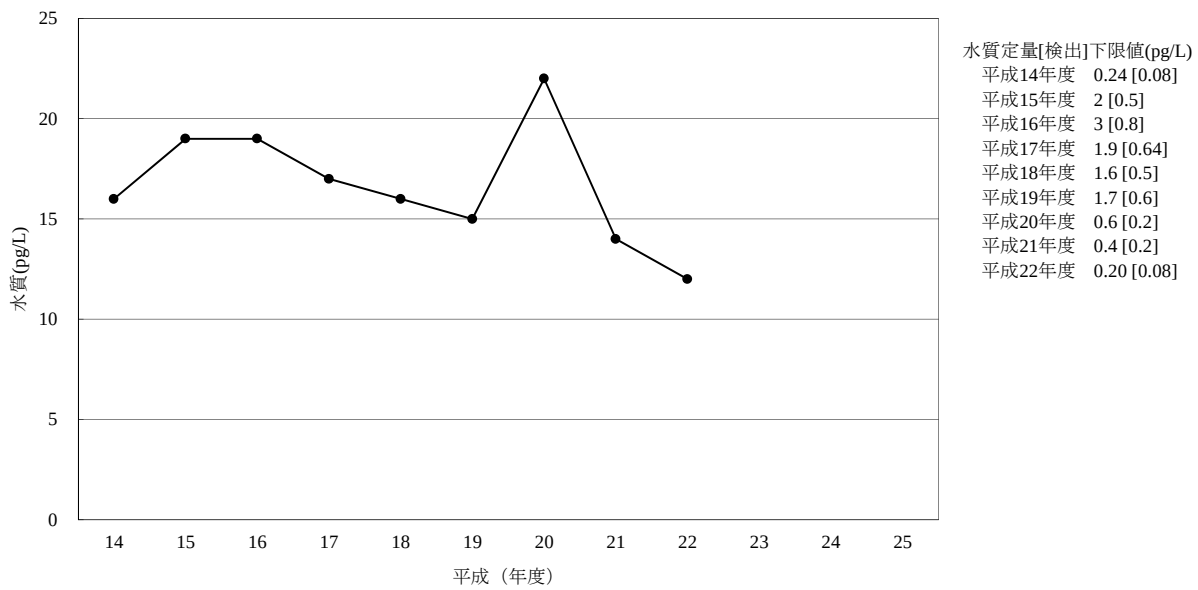
[6-3] p,p' -DDD
