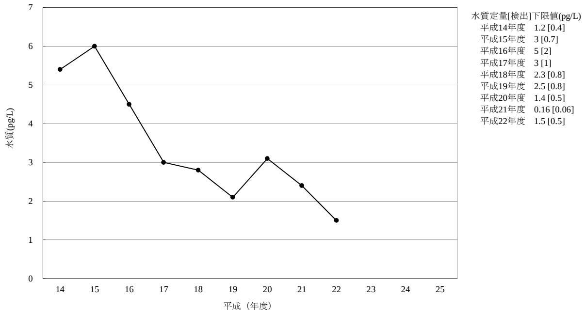
[6-4] o,p' -DDT
