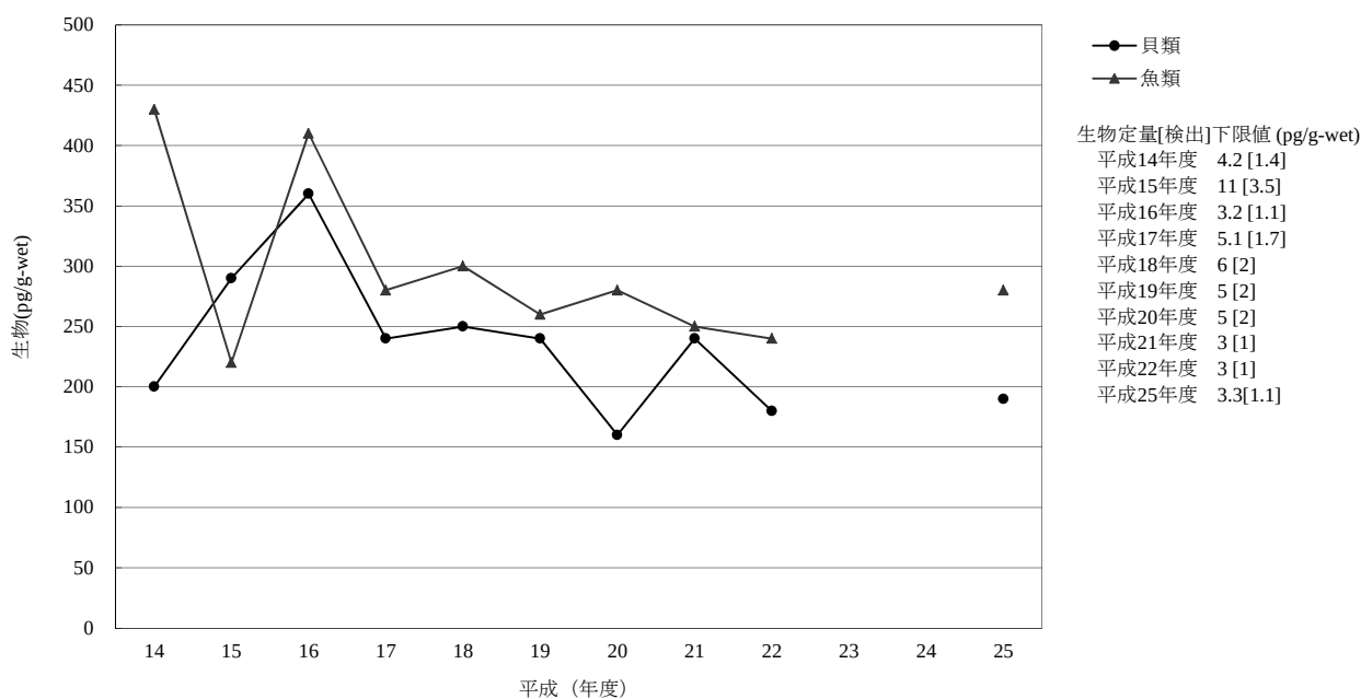
[6-1] p,p' -DDT
