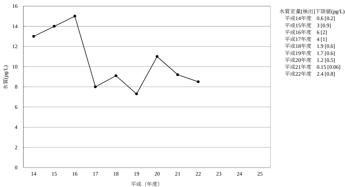
[6-1] p,p' -DDT
