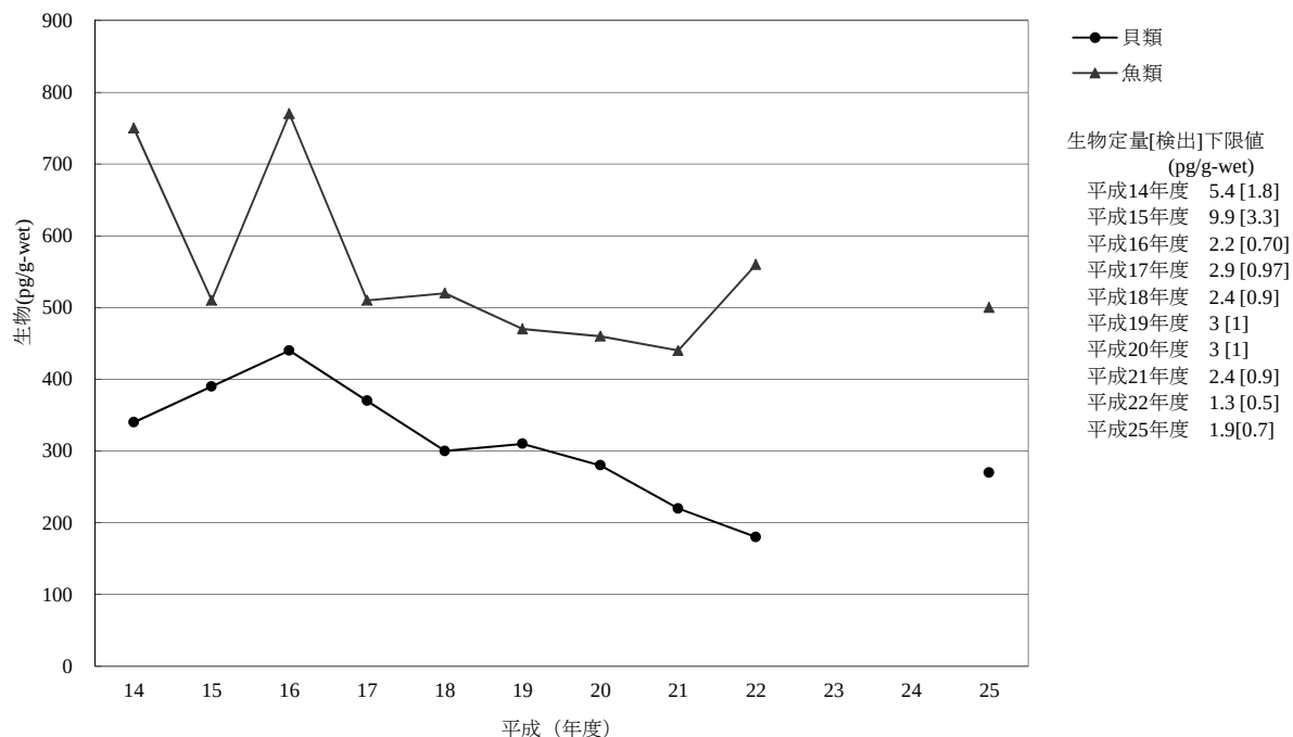
[6-3] p,p' -DDD
