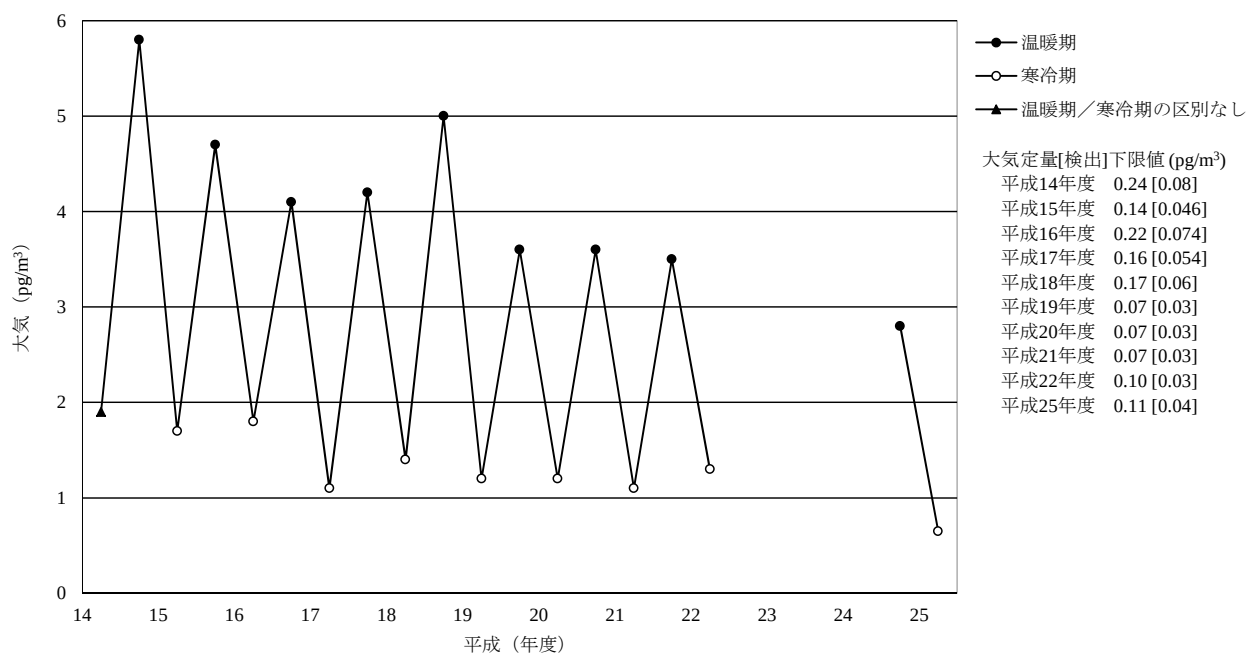
[6-1] p,p' -DDT
