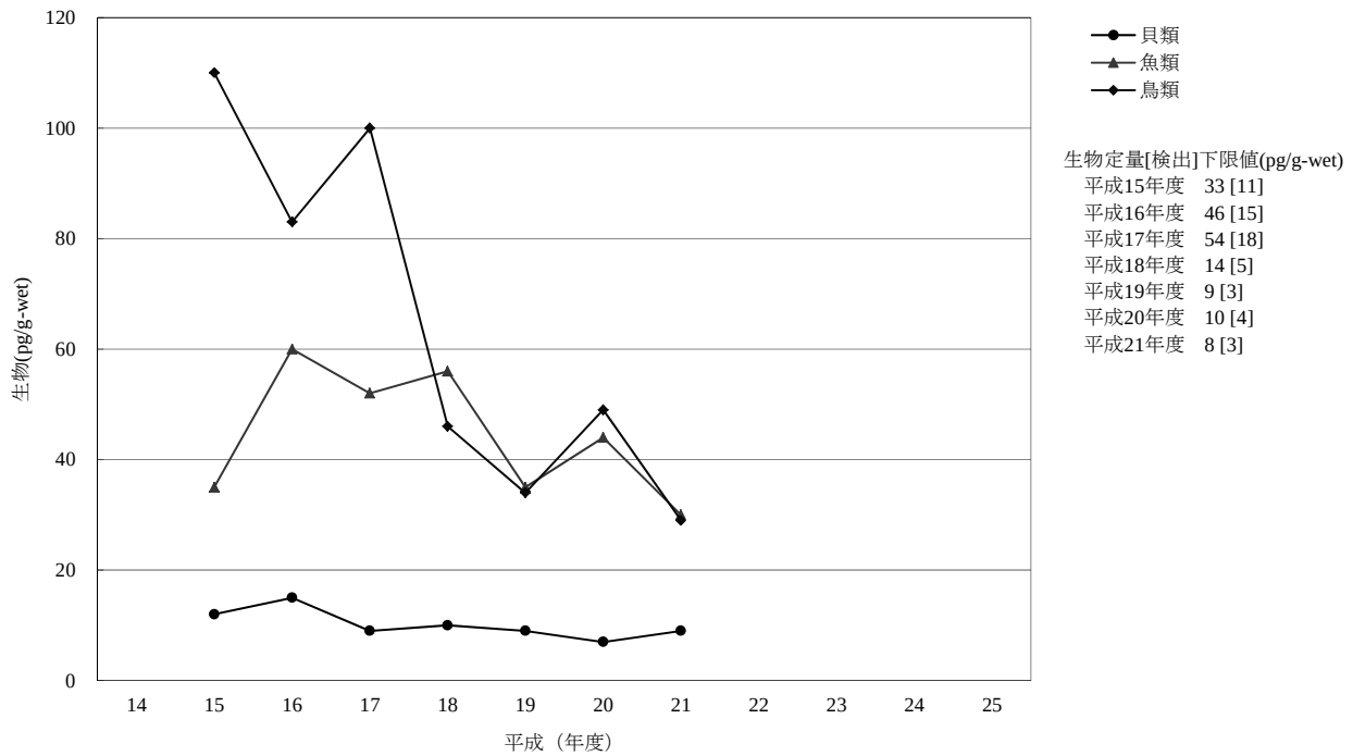
[9-2] Parlar-50
