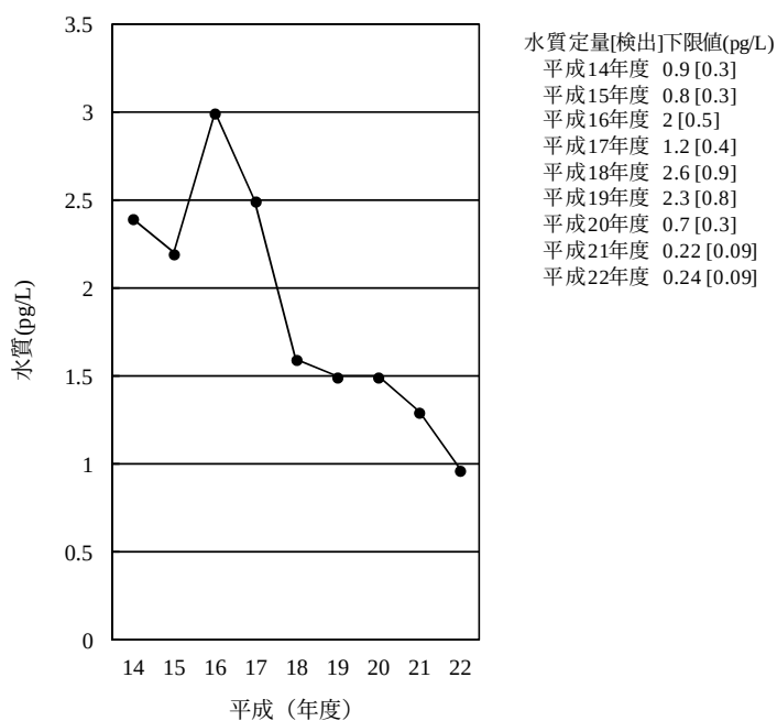
[6-5] o,p' -DDE
