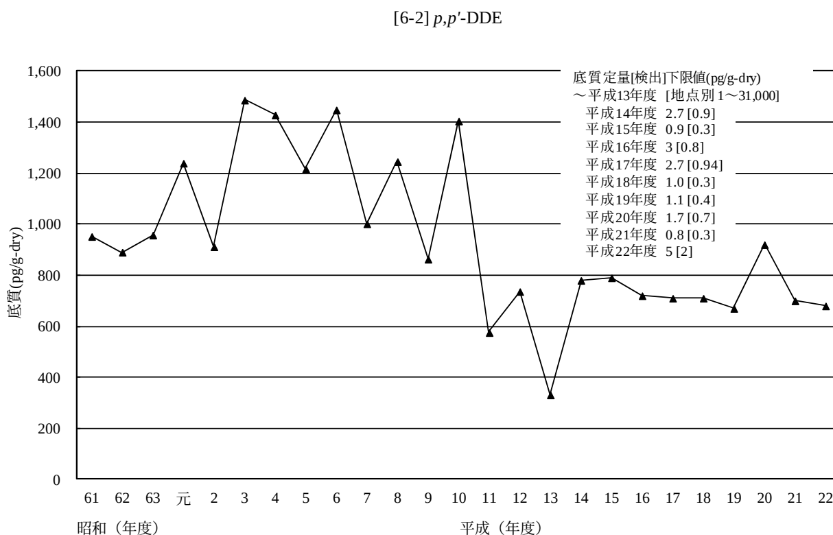
図 7-6-2-2 p,p' -DDE の底質の経年変化 (幾何平均値)
