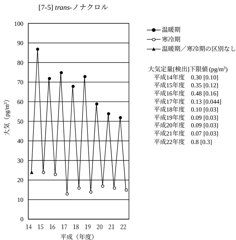
図 7-7-5-4 trans -ノナクロルの大気経年変化(幾何平均値)
