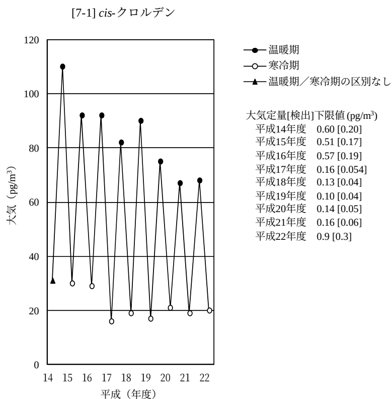
図 7-7-1-4 cis -クロルデンの大気経年変化(幾何平均値)
