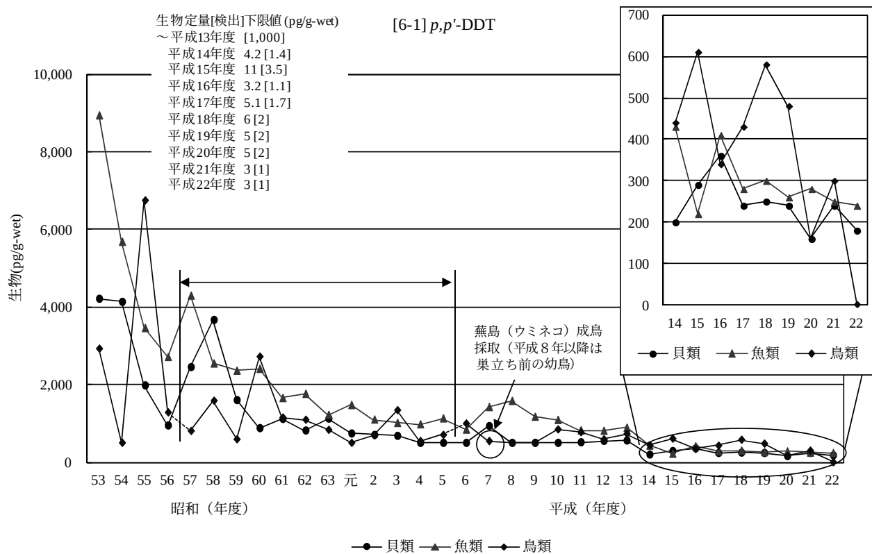
(注) 平成21年度以前は、各地点における算術平均値を求め、その算術平均値から全地点の幾何平均値を求めた。 図 7-6-1-3 p,p' -DDT の生物の経年変化 (幾何平均値)
