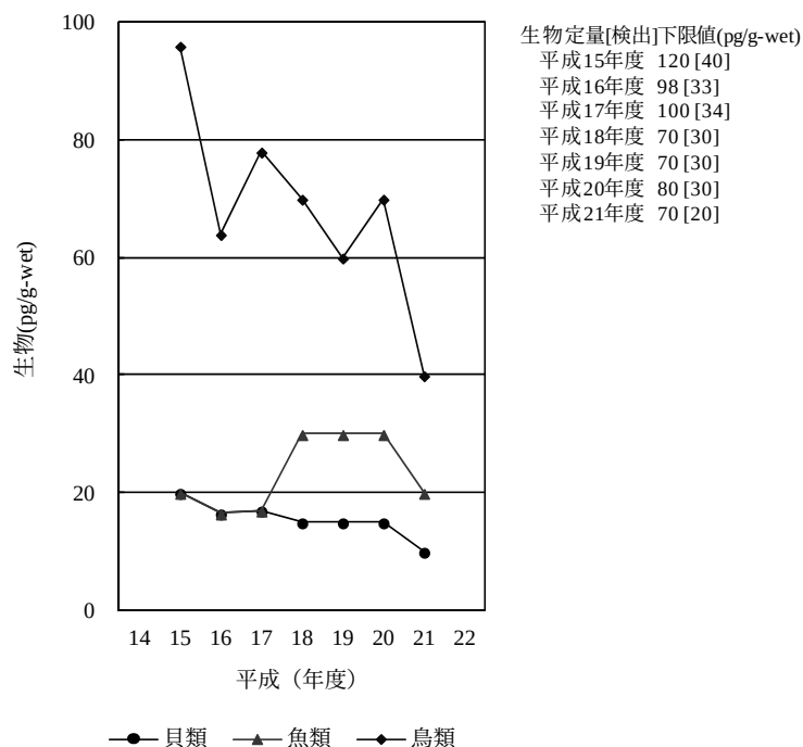
[9-3] Parlar-62
