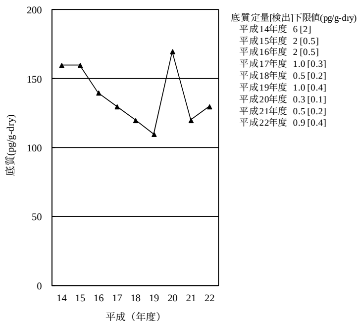
[6-6] o,p' -DDD
