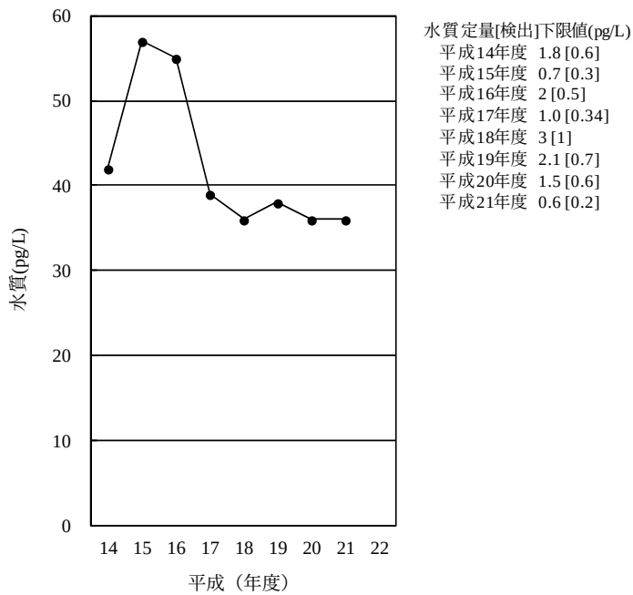
図 7-4-1 デイルドリンの水質の経年変化 (幾何平均値)
