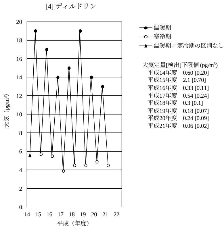
図 7-4-4 ディルドリンの大気経年変化（幾何平均値）
