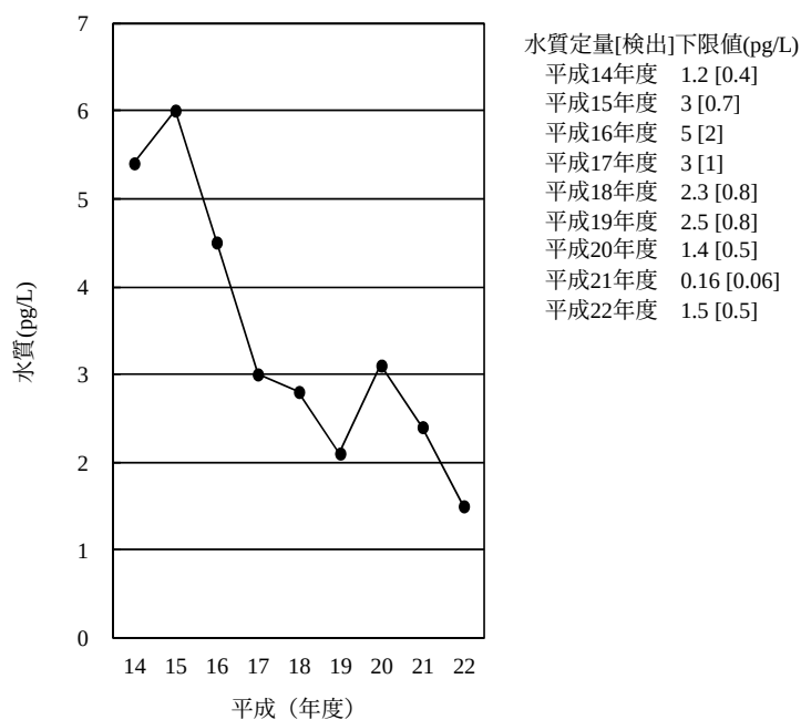
[6-4] o,p' -DDT
