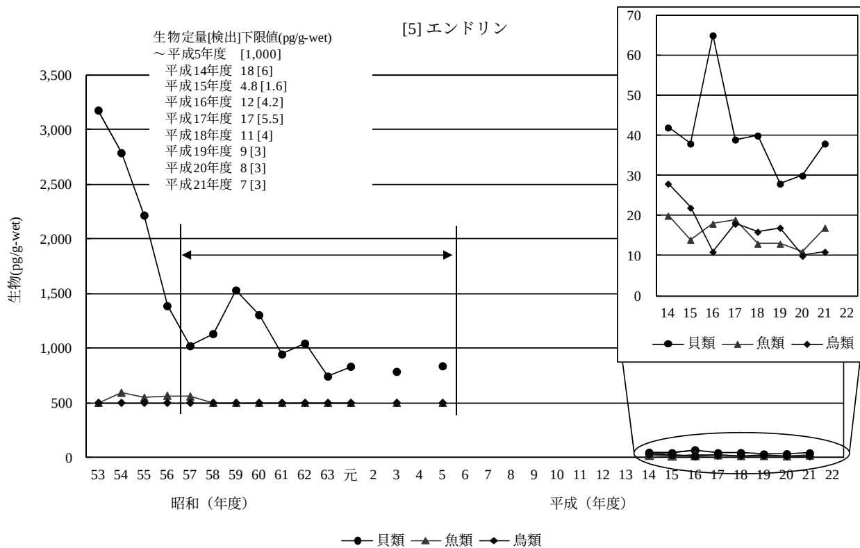
(注) 平成 21 年度以前は、各地点における算術平均値を求め、その算術平均値から全地点の幾何平均値を求めた。 図 7-5-3 エンドリンの生物の経年変化 (幾何平均値)
