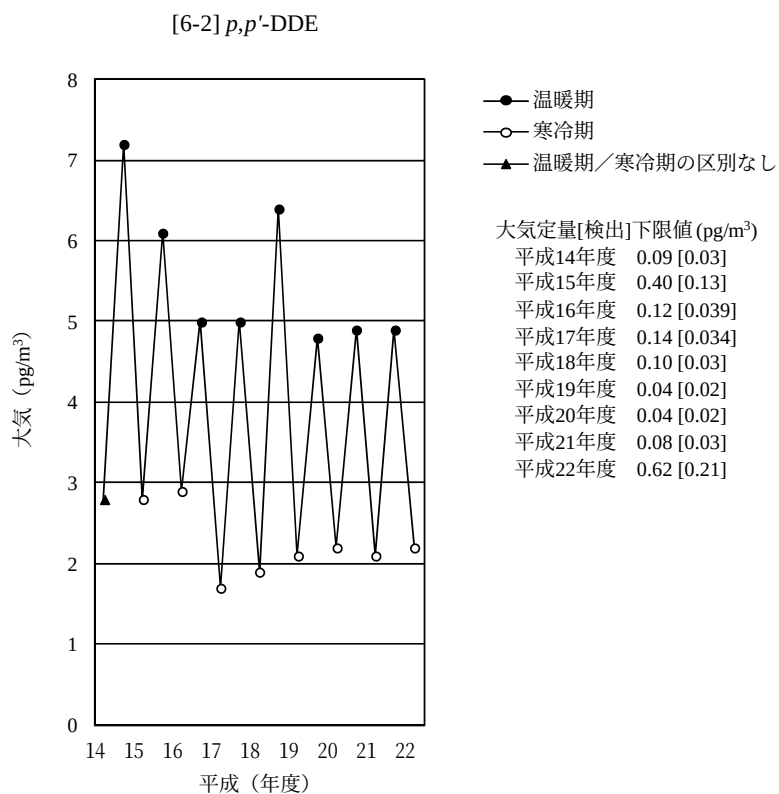
図 7-6-2-4 p,p' -DDE の大気の経年変化（幾何平均値）
