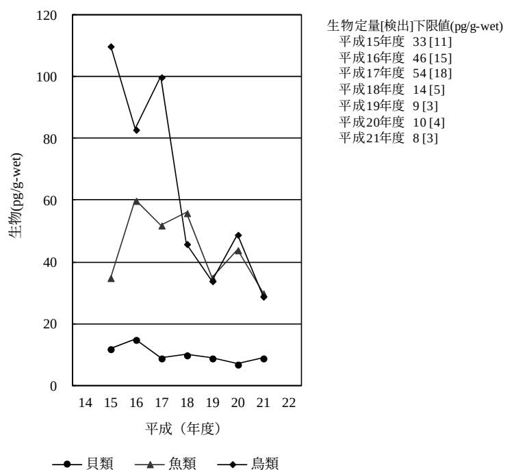
[9-2] Parlar-50
