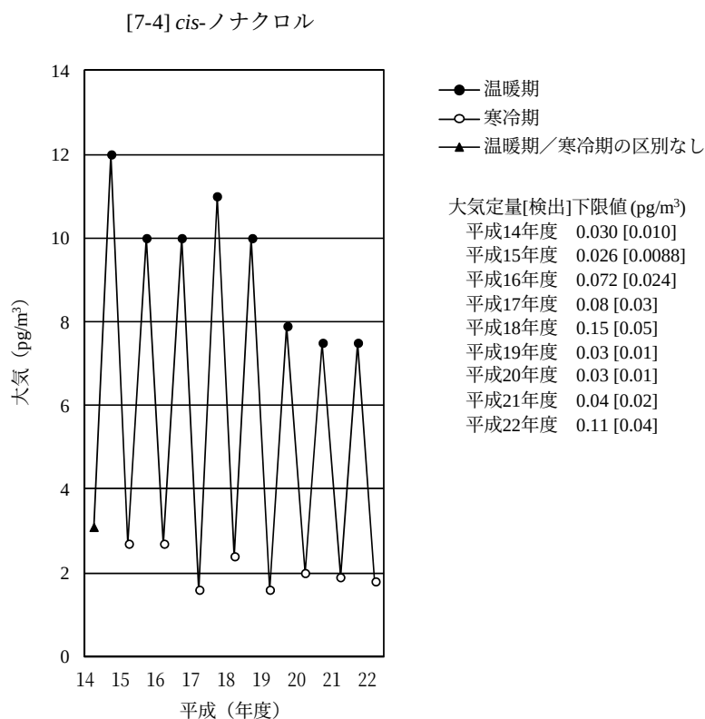
図 7-7-4-4 cis-ノナクロルの大気の経年変化(幾何平均値)
