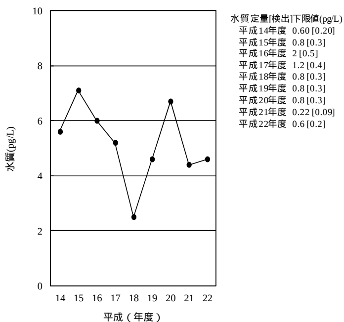
[6-6] o,p' -DDD
