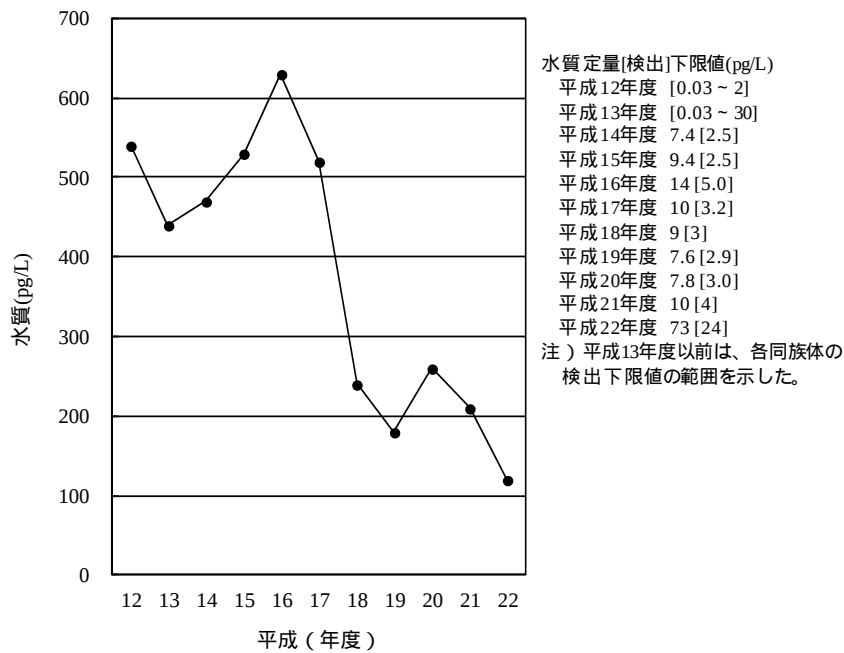
[1] PCB類
