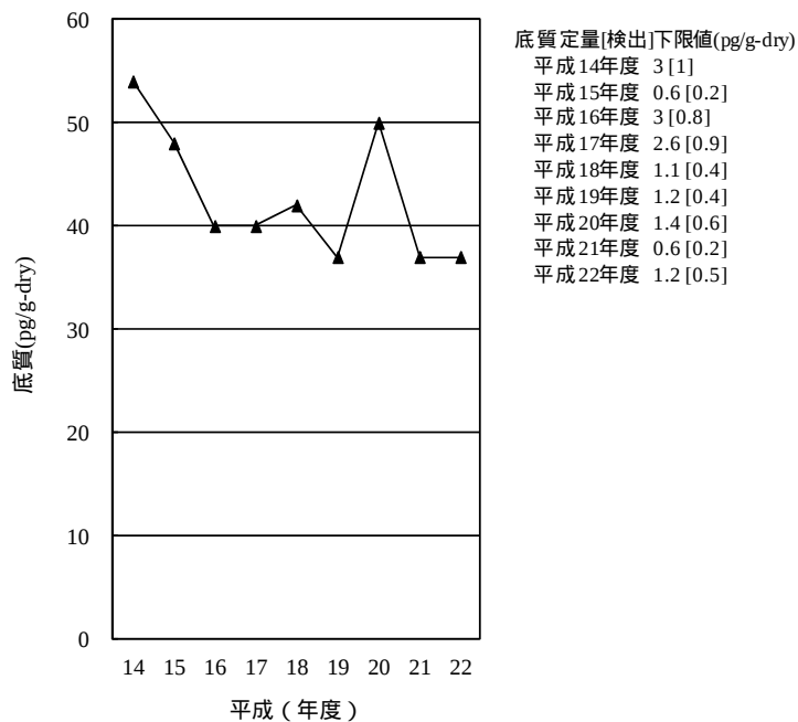
[6-5] o,p' -DDE
