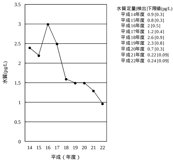
[6-5] o,p' -DDE
