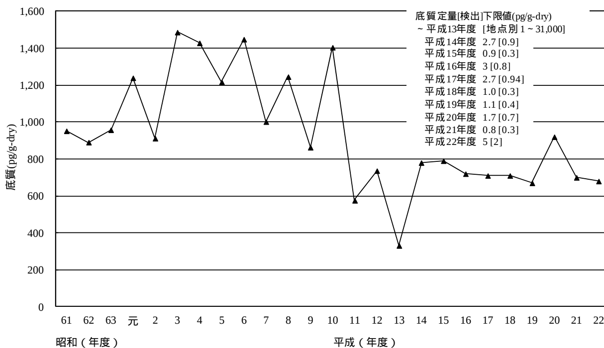
[6-2] p,p' -DDE
