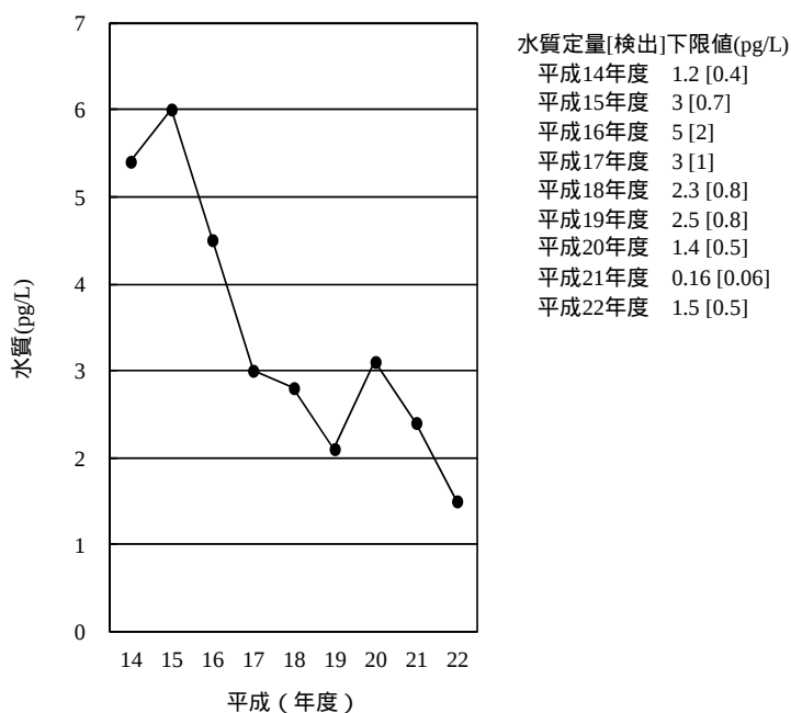
[6-4] o,p' -DDT
