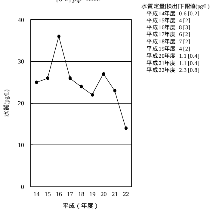
[6-2] p,p' -DDE
