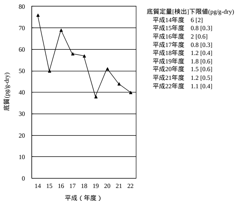
[6-4] o,p' -DDT
