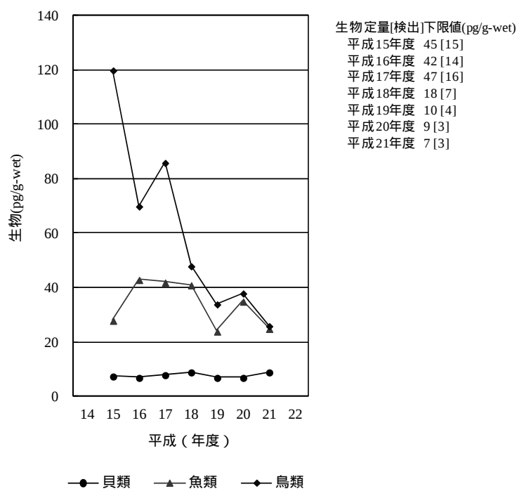
[9-1] Parlar-26
