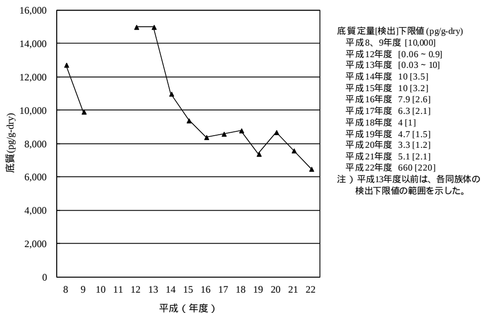
[1] PCB類
