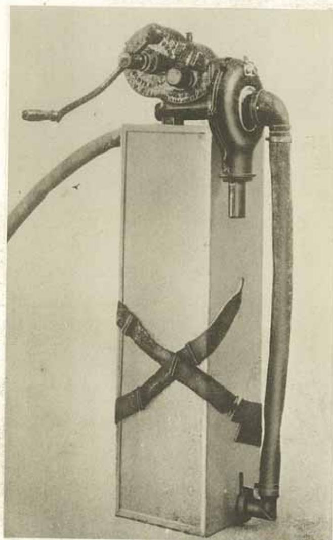
米軍用濾函 (C. W.)
