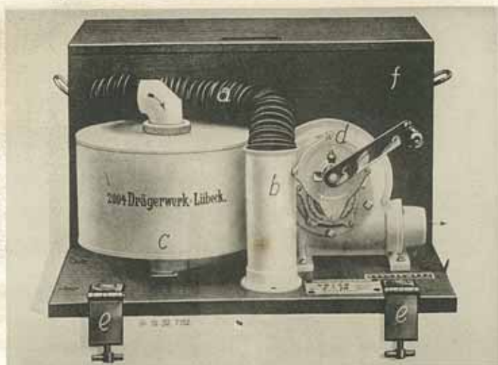
「ドレーガー」社手動濾函 (D. H. 1933)
