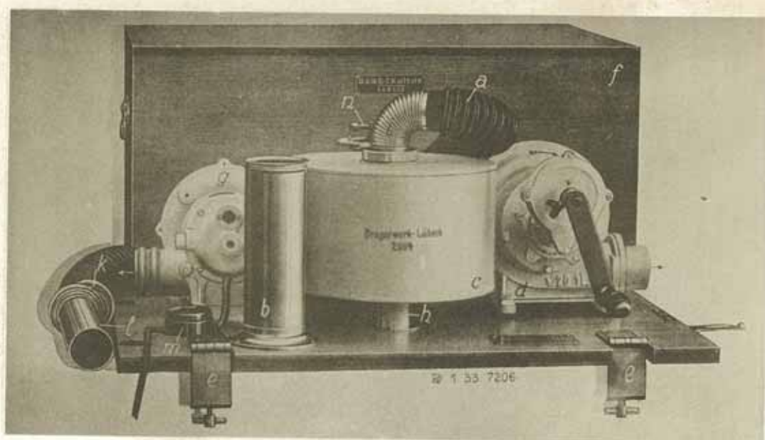
ドレーガー社手電動式濾函 (D. H. 1933)
