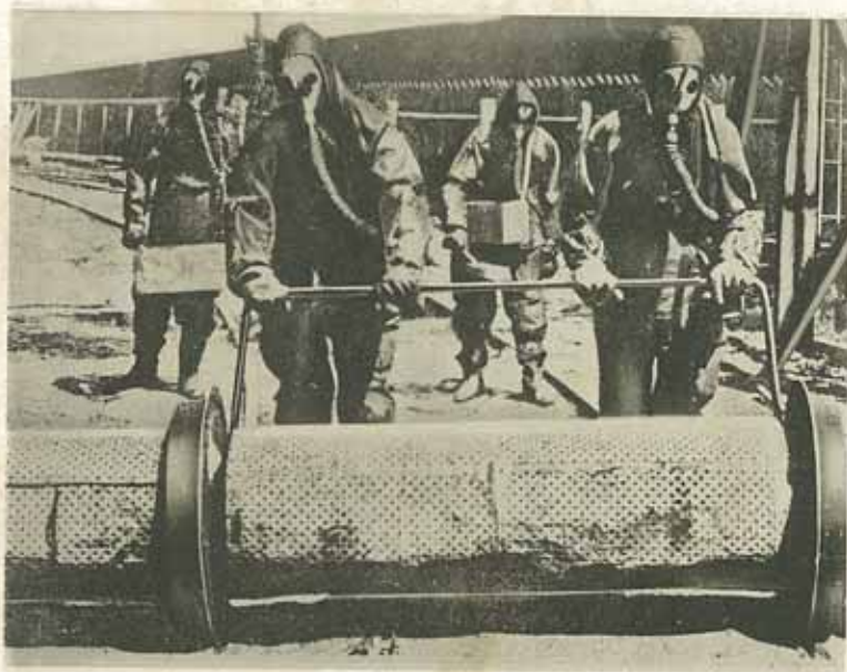
鼓胴型晒粉撒布車に依て糜爛劑の消毒の状況(蘇邦)
