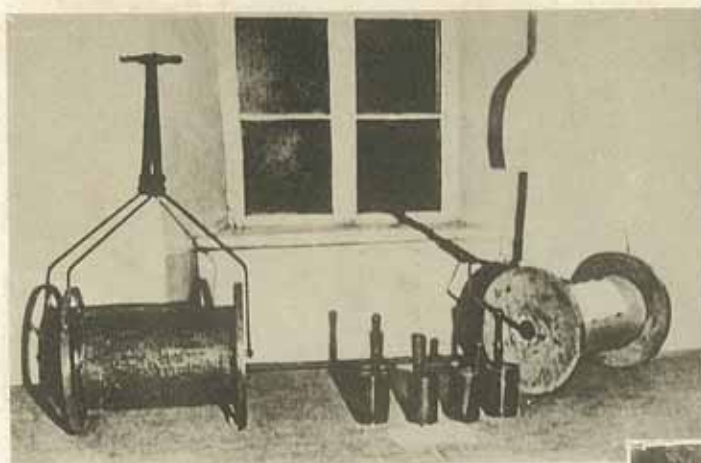
「エストニア」防空演習に際し「タリン」に於て 観覧に供せる鼓胴消毒器と手持型消毒器なり (R. I. C. R.)
