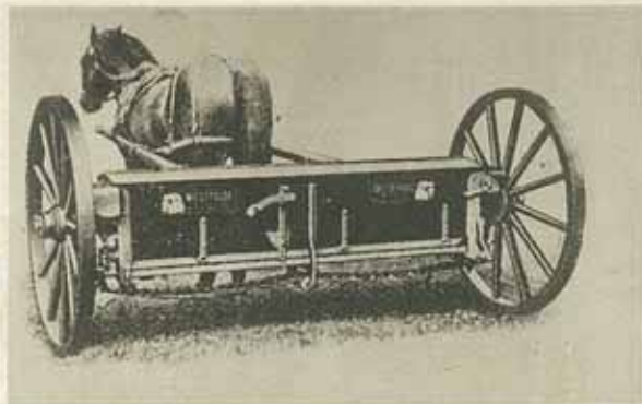
獨逸の繋駕 晒粉撒布用消毒車(撒肥車を利用す) (G. L. 1932)
