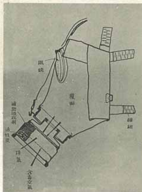
獨軍一九一八年型直結式防毒面断面圖 (H. T.)
