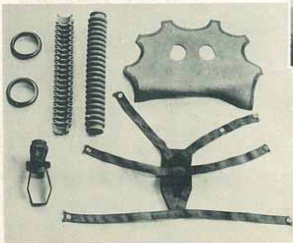
隔離式工業用防毒面の覆面の部分品
