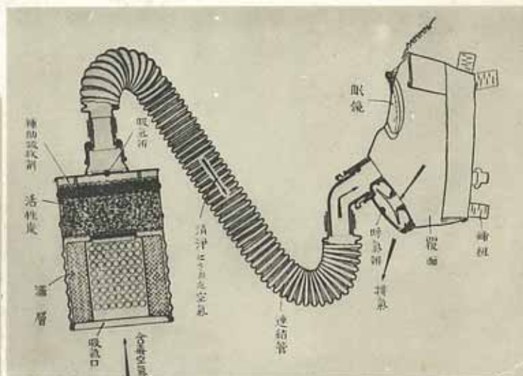
獨逸二四年型軍用隔離式防毒面の構造要圖 (H. T.)
