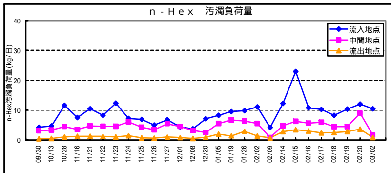
図5-7 実証試験施設における負荷量及び除去率の結果(1)
