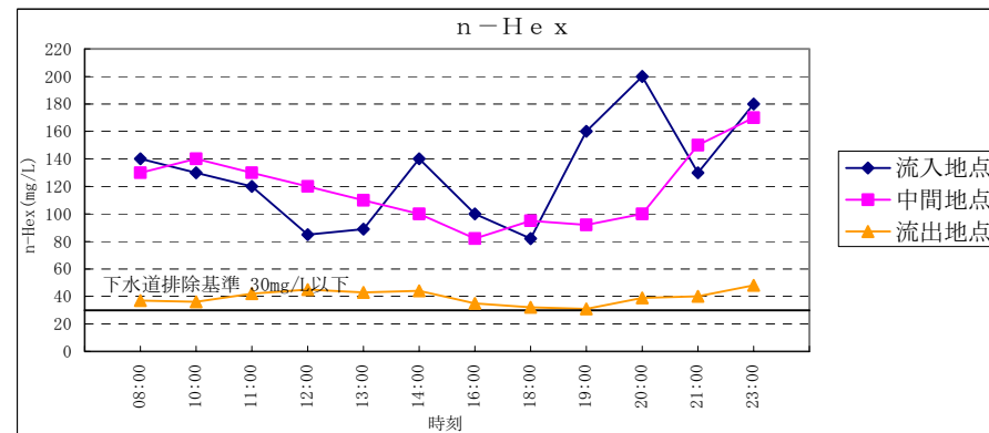
図5-1 日間変動調査(1) 第1回目(平成16年11月16日)
