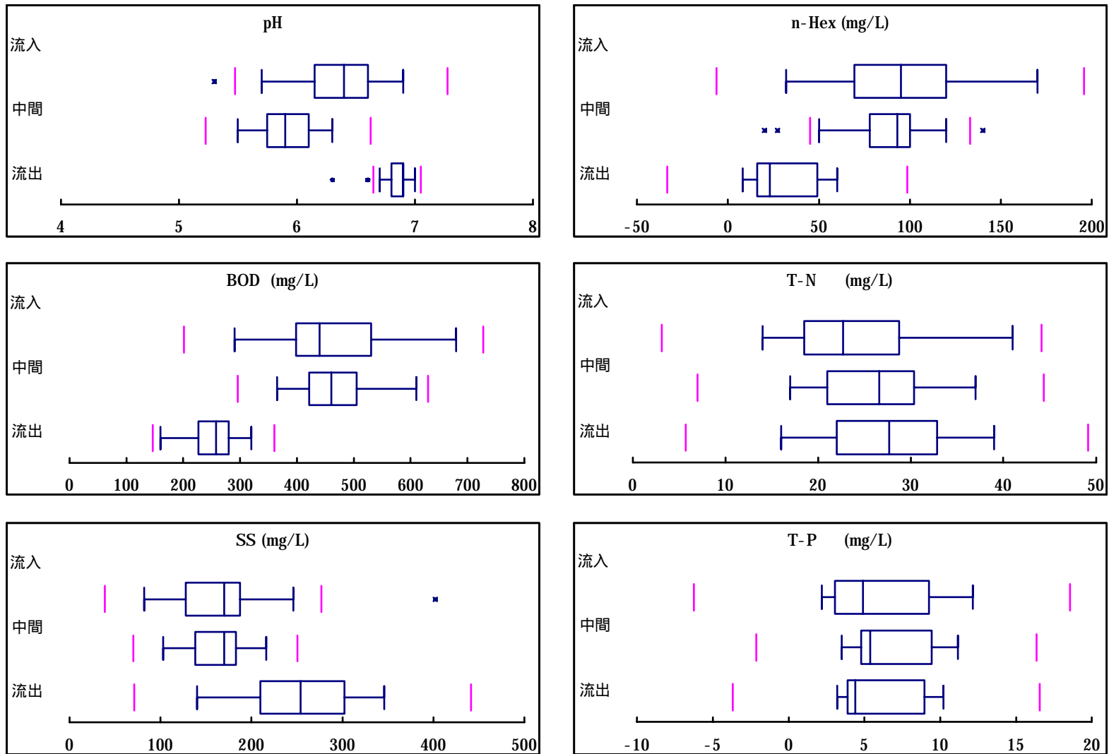
図 5- 5 水質分析結果の箱型図
