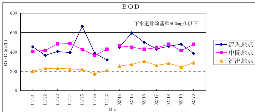
図 5 - 2 週間変動調査
