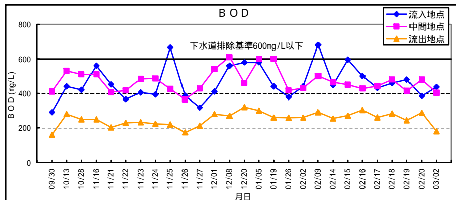
図5 - 4 水質分析結果の経日変化
