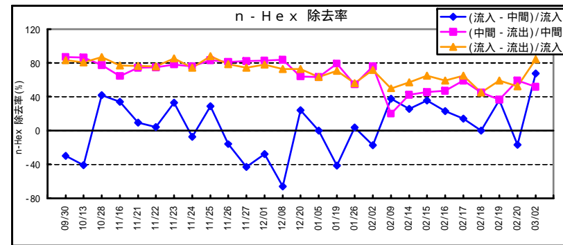
図5-7 実証試験施設における負荷量及び除去率の結果(1)
