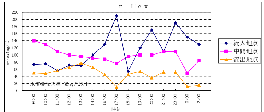
図5-1 日間変動調査(2) 第2回目(平成17年1月26日)
