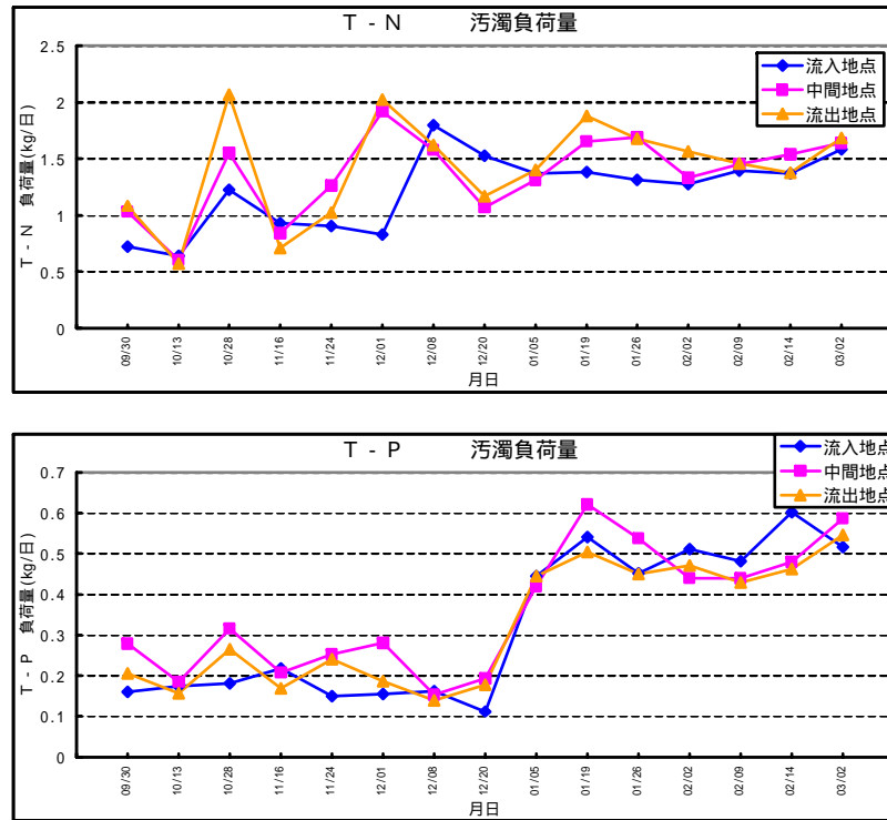
図5 - 7 実証試験施設における負荷量及び除去率の結果(2) 印: 参考項目
