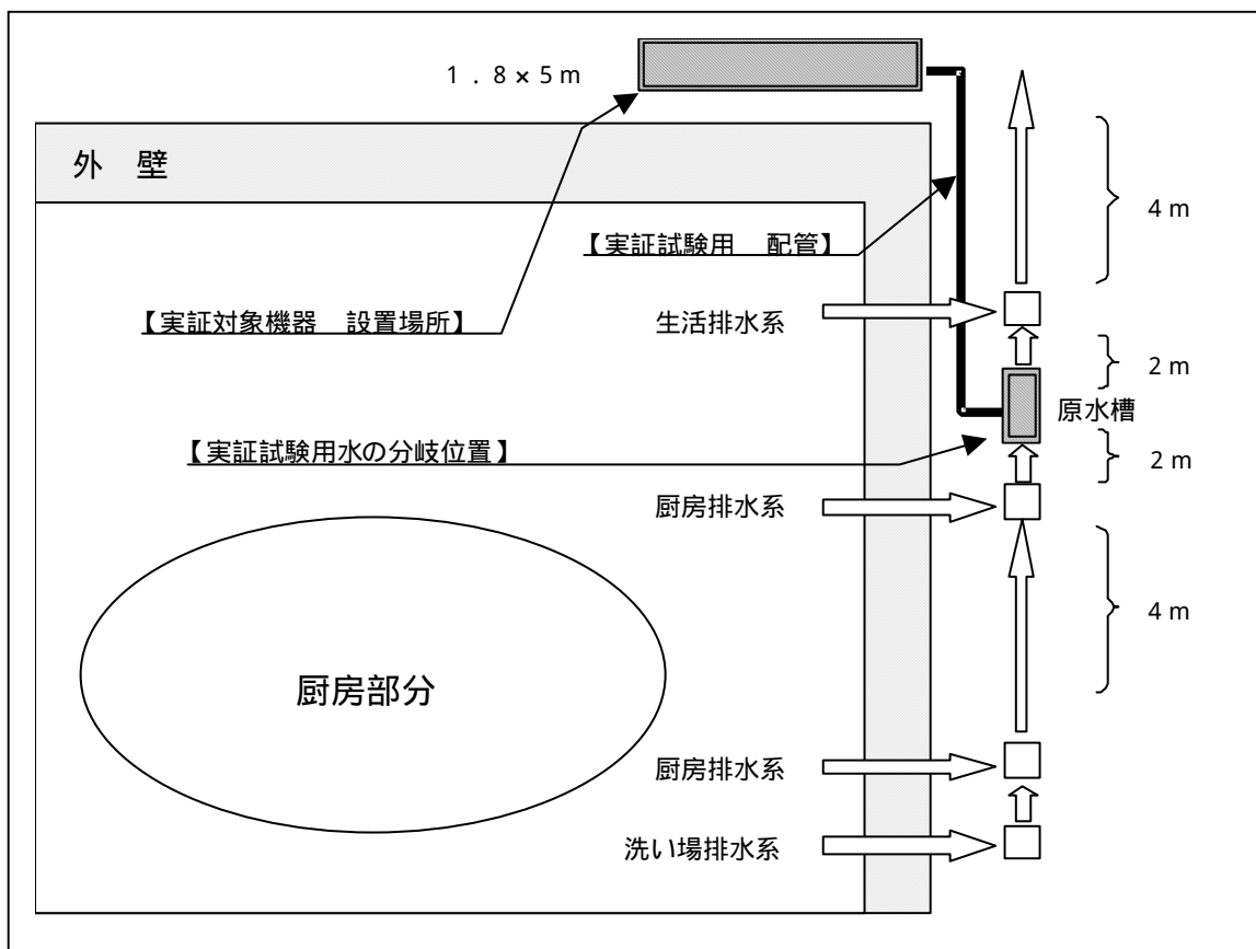
図3-1 排水系統図
