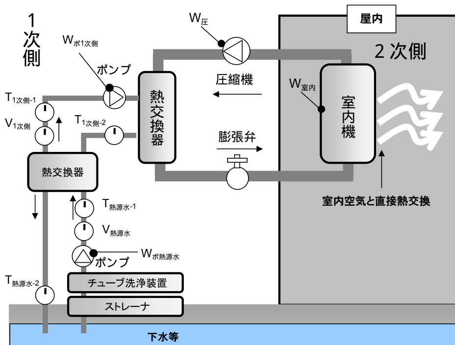
図7 システム全体の実証における測定箇所(下水等熱源の場合)
