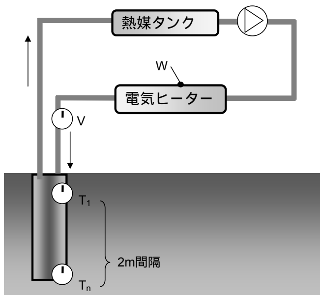
図 10-10 地中熱交換部の実証における測定点
