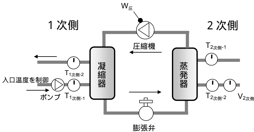
図 887 ヒートポンプのみの実証における測定点
