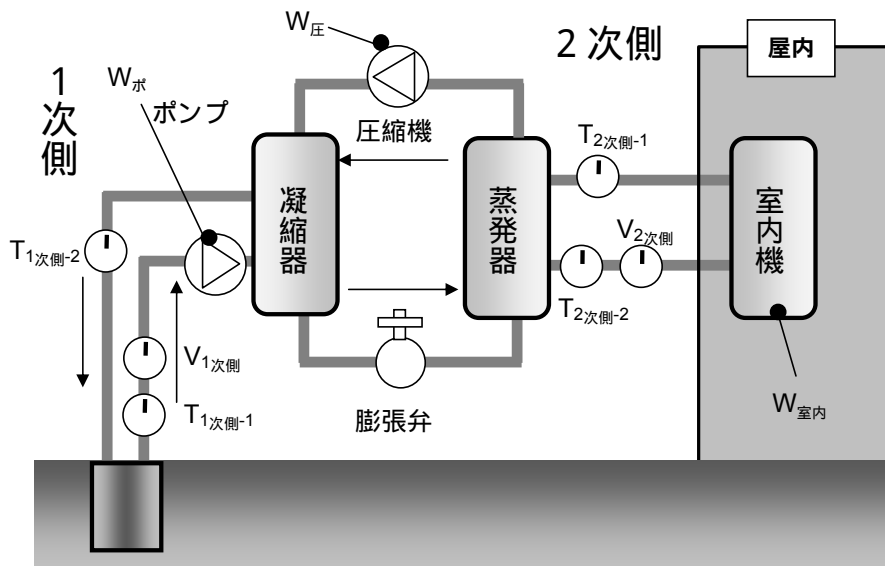
図 4 システム全体の検証における測定箇所 (間接式の場合)
