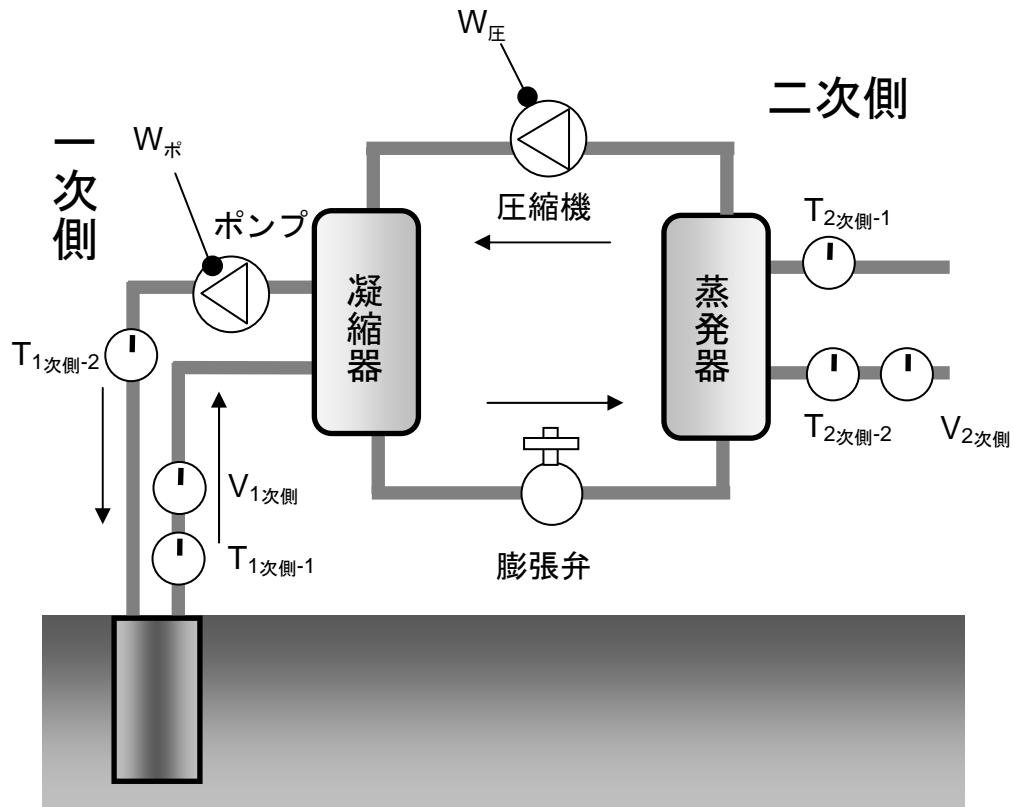
図5 システム全体の実証における測定箇所（間接方式の場合）
