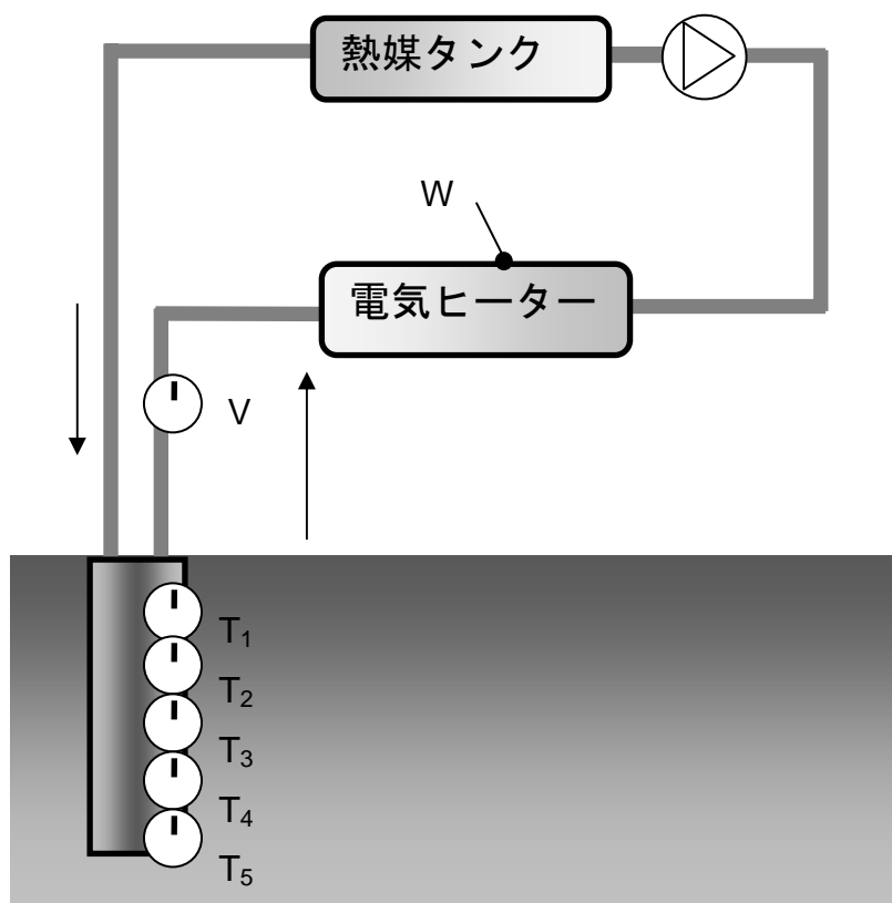
図 10 地中熱交換部の実証における測定点
