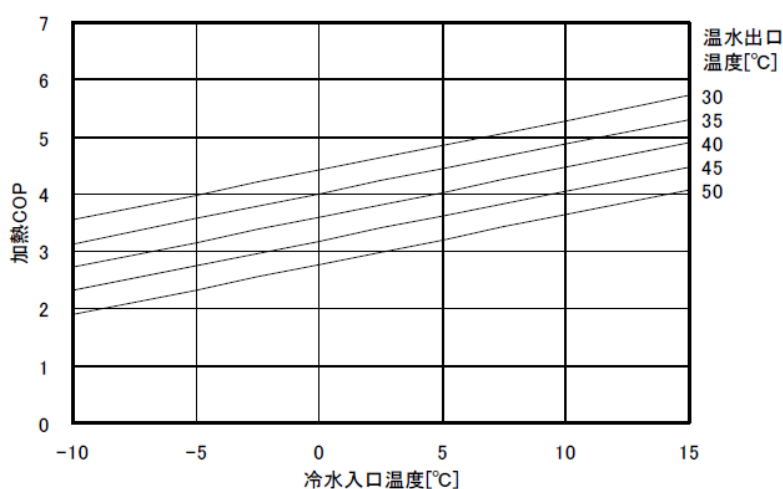
図 7 COP 特性グラフの例 (暖房時)
