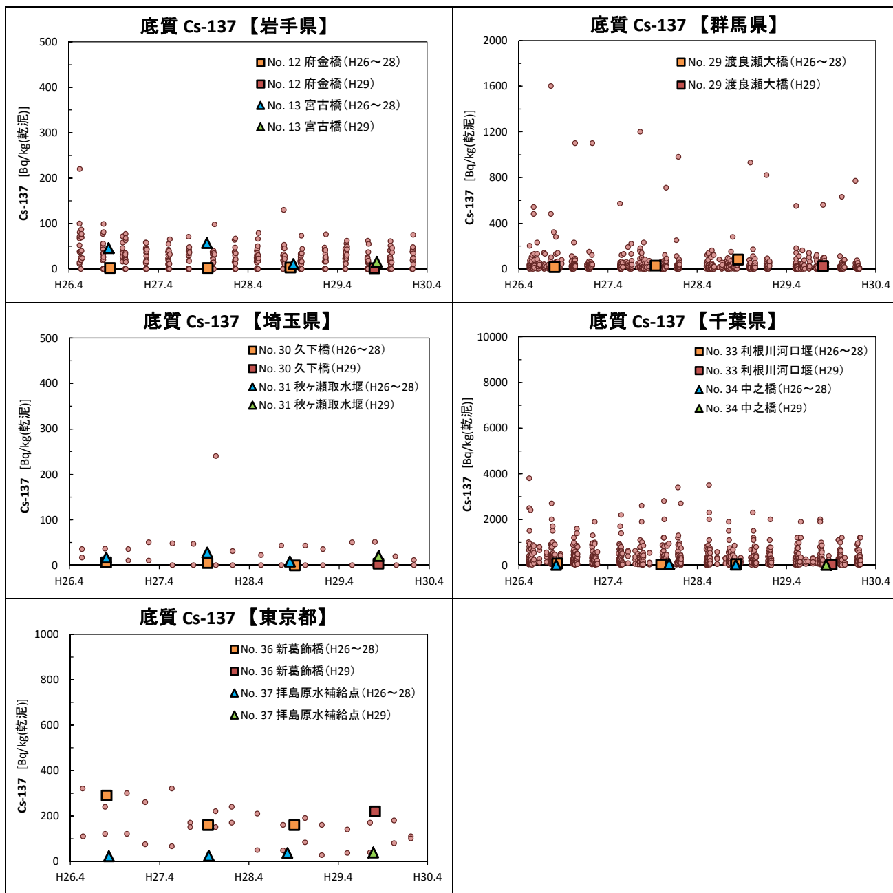
図 3. 2-9 (2) ①震災対応モニタリングの同一都県での調査結果との比較【Cs-137】
