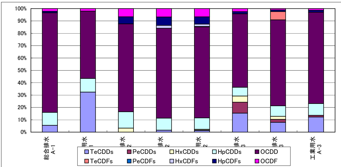
図-14 排水水 PCDDs/DFs同族体組成
