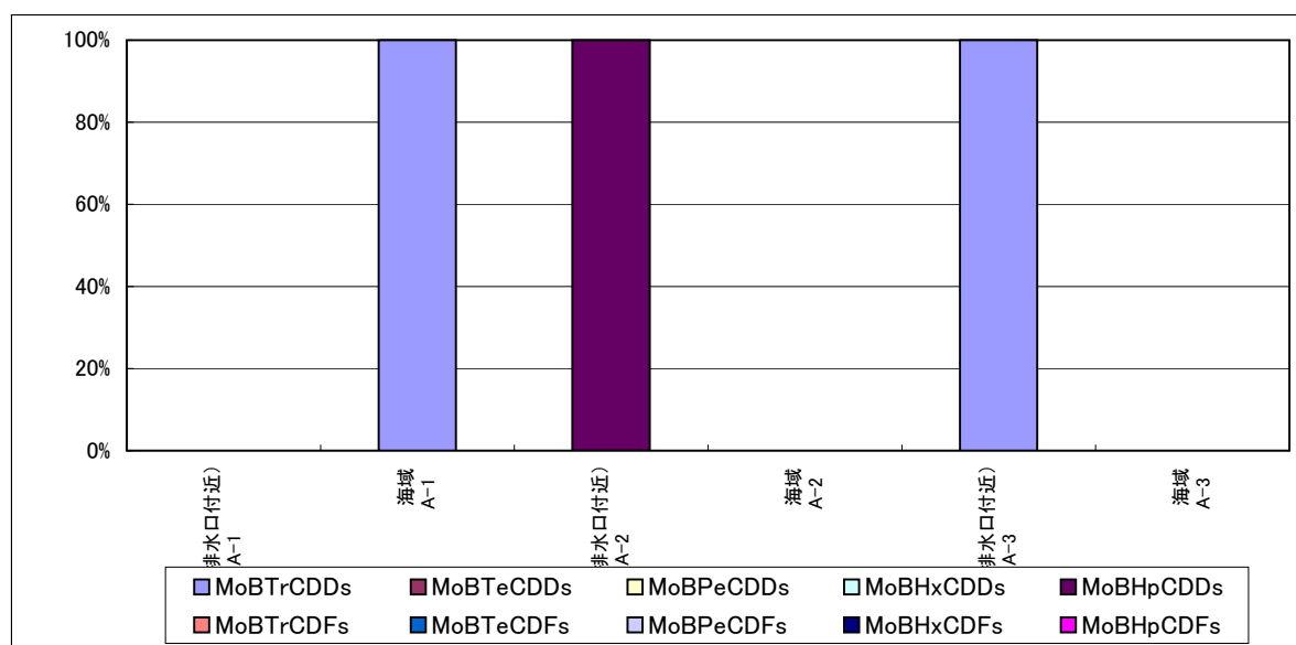
図-11 公共用水域水質 MoBPCDDs/DFs同族体組成
