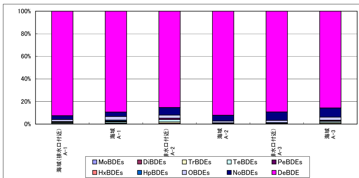
図-23 公共用水域水質 PBDEs同族体組成
