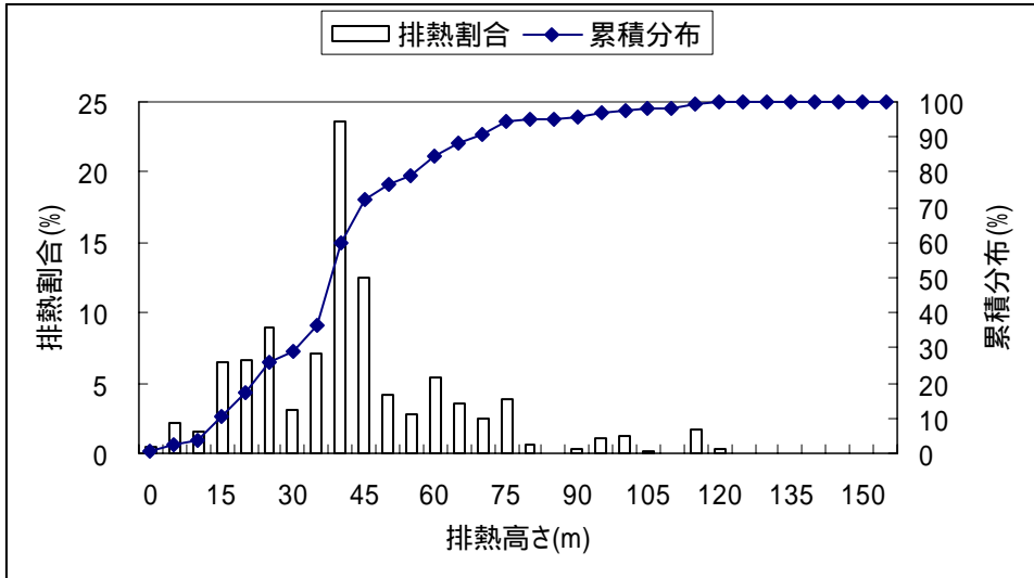
図 10 空冷ヒートポンプ排熱の排出高さ
