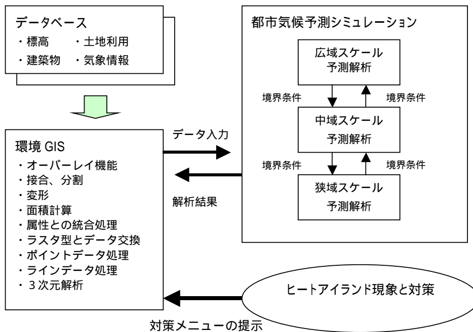
図5 - 2 U C S Sモデルの概要
