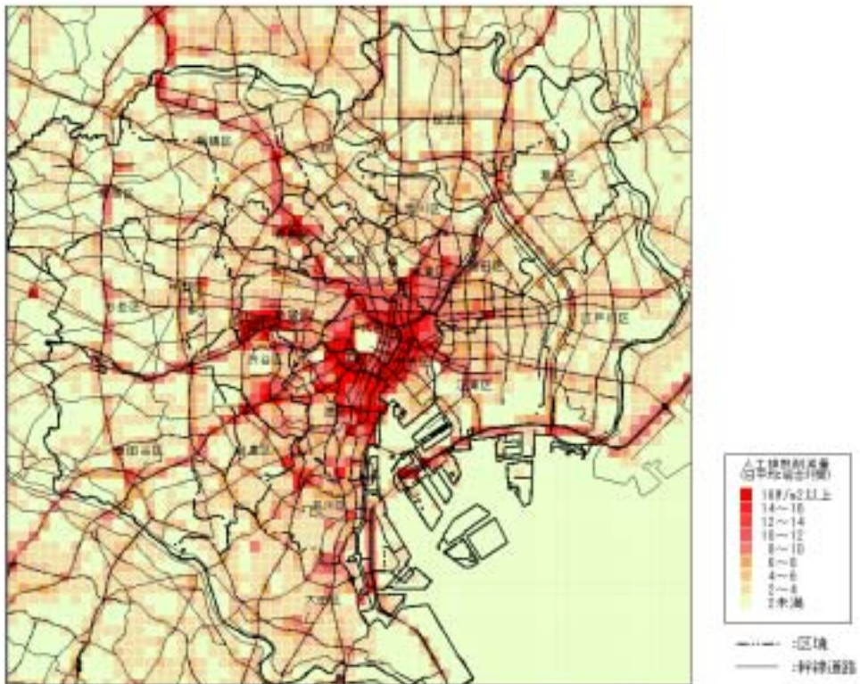
図5 - 7 総合対策による人工排熱削減量（日平均）分布：東京23区
