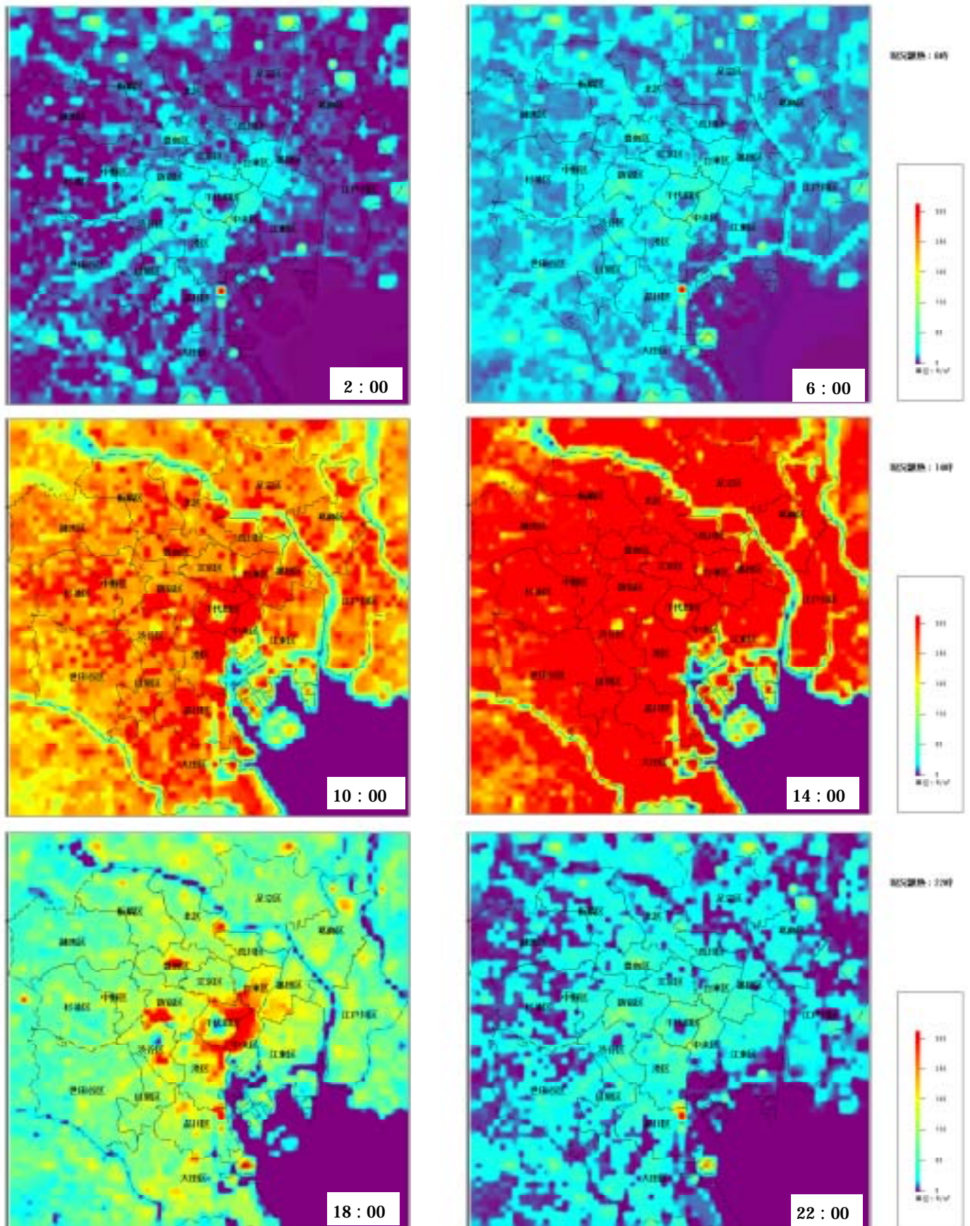
図3.5 顕熱分布の時間変化(23区現況)
