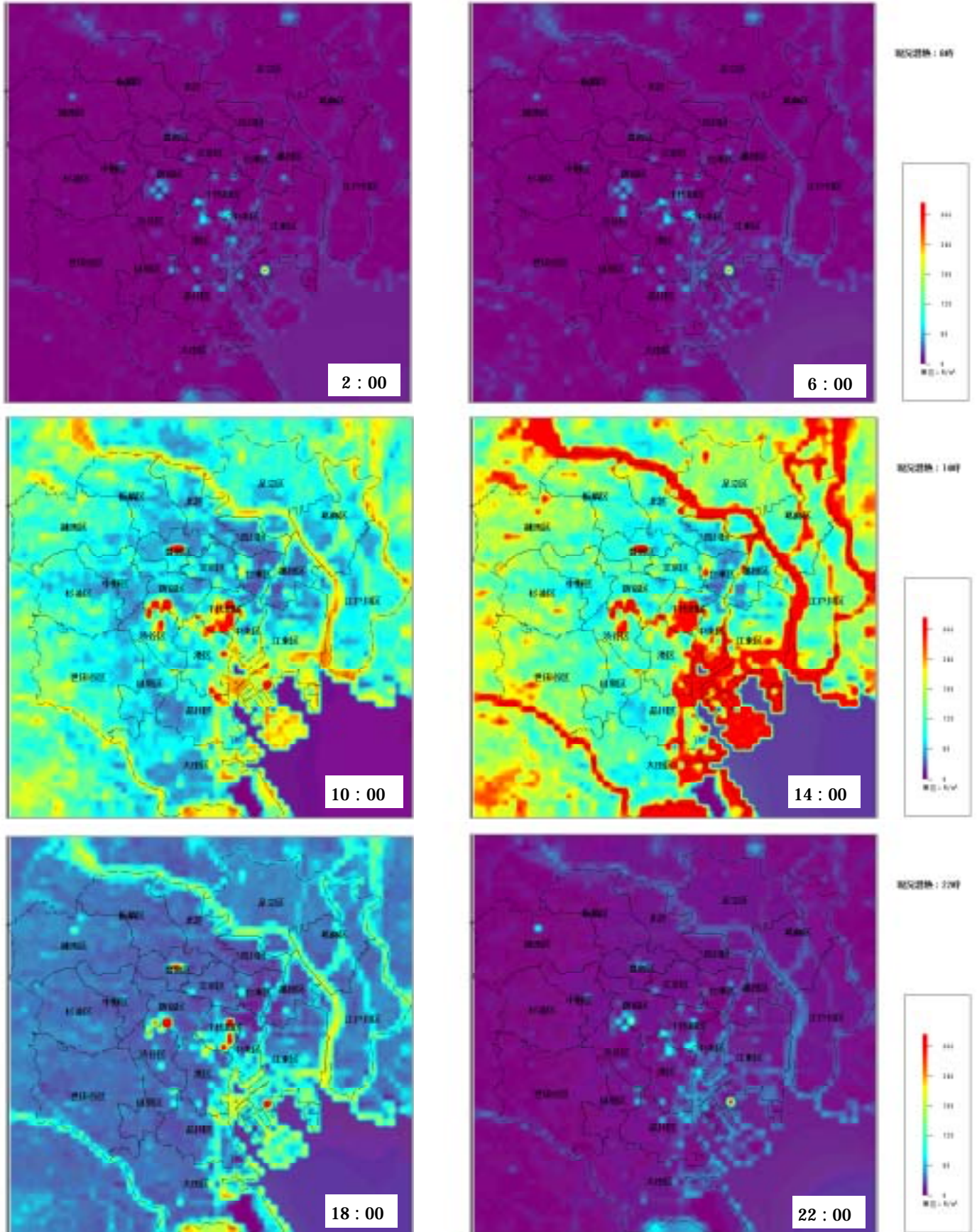
図3.6 潜熱分布の時間変化(23区現況)
