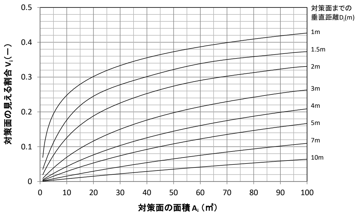
図4 対策面の面積、対策面までの垂直距離と対策面に見える割合（縦横比 R_{H/W}=1 の場合）
