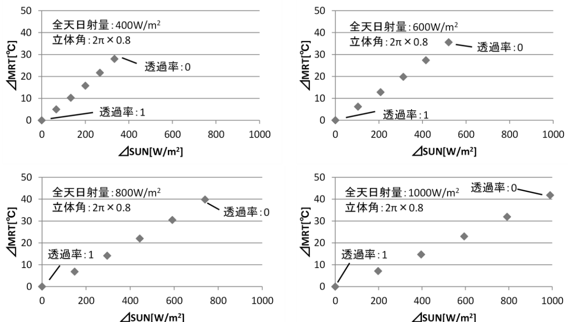
図 2 \angle \text{SUN} と \angle \text{MRT} との関係
