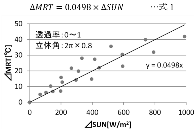
図 5 \angle SUN と \angle MRT との関係
