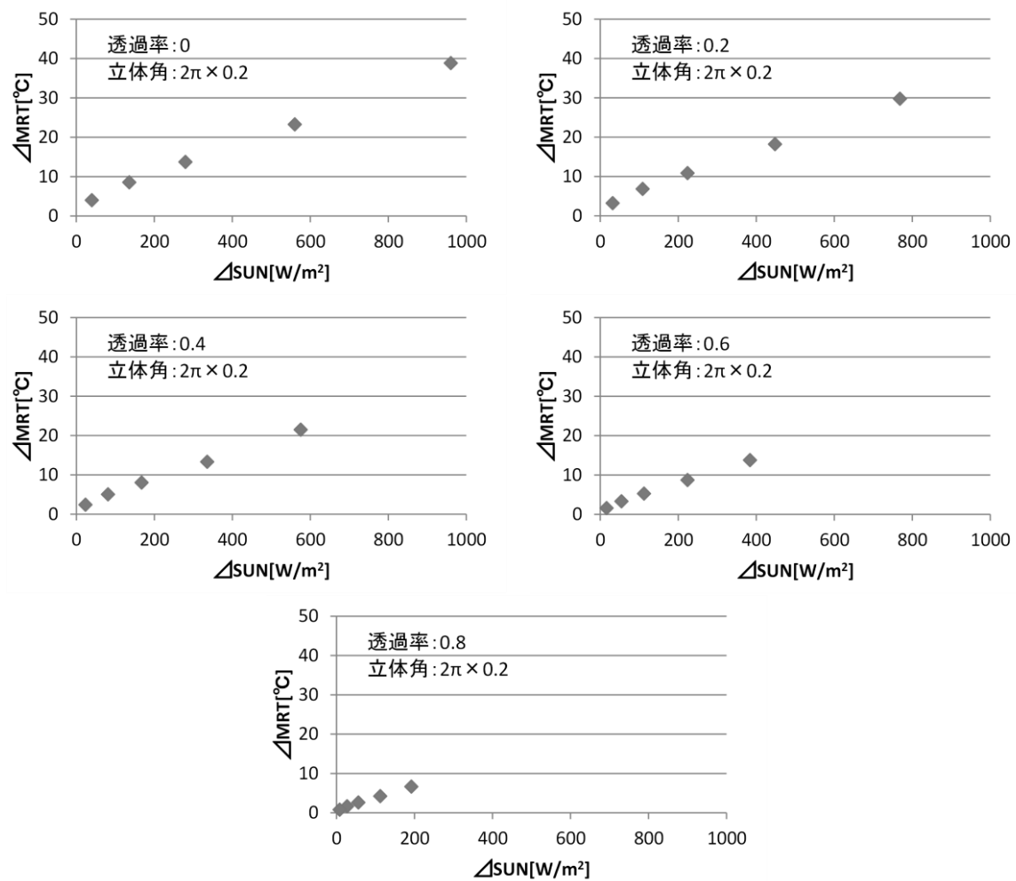
図 8 \Delta \text{SUN} と \Delta \text{MRT} との関係
