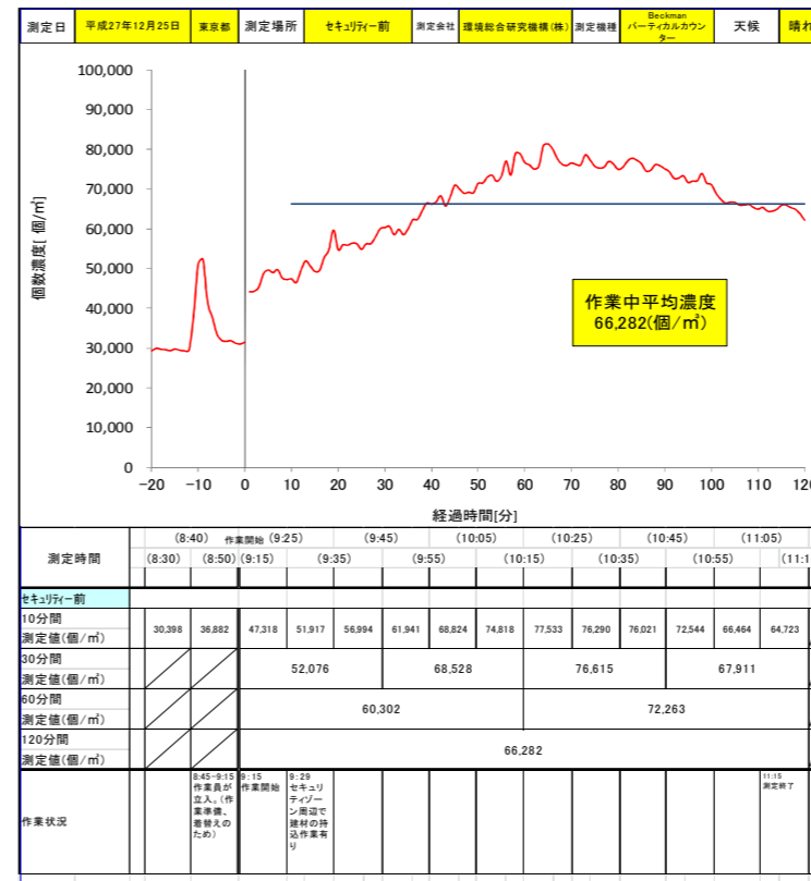
パーティクルカウンター(0.5 μm)
