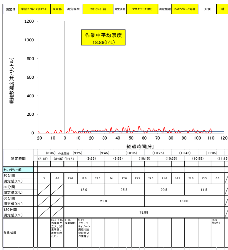
リアルタイムファイバーモニター
