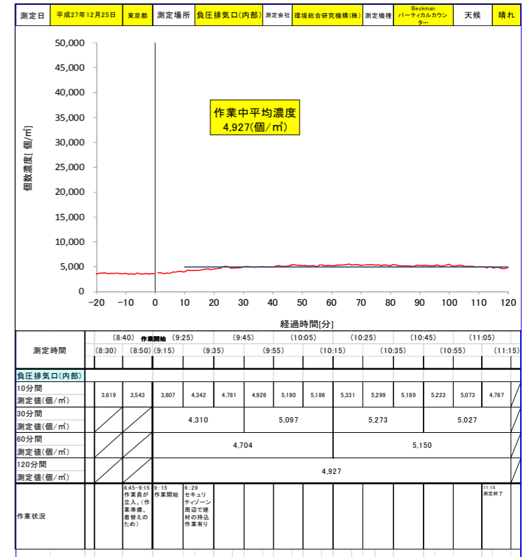
パーティクルカウンター(0.3 μm)
