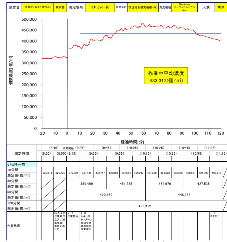
パーティクルカウンター(0.3 μm)
