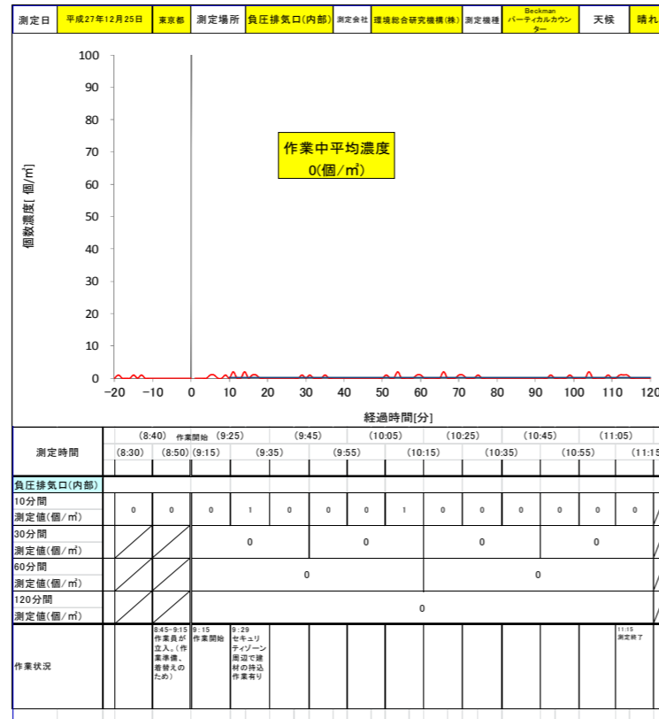
パーティクルカウンター(5.0 μm)
