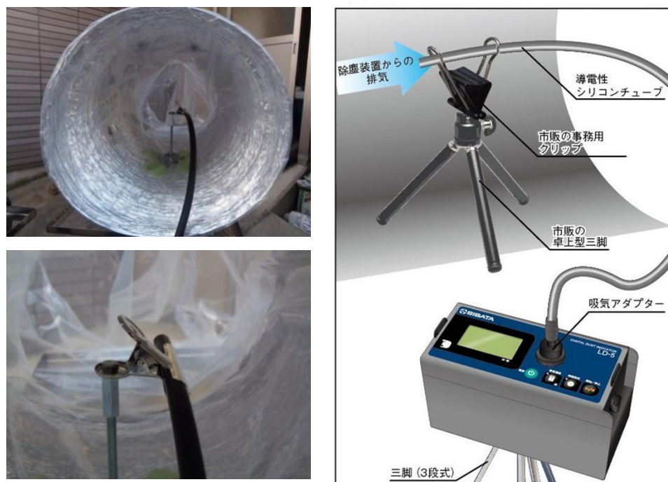
図4.14.15 チューブ配管を使用した場合の排気ダクトの測定例
