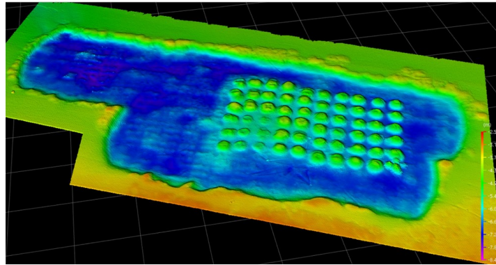
図 5-9. 細井沖浚渫窪地の深浅図 2 (2022 年 10 月, (株)ウエスコ測量) (国土地理院写真を利用).
