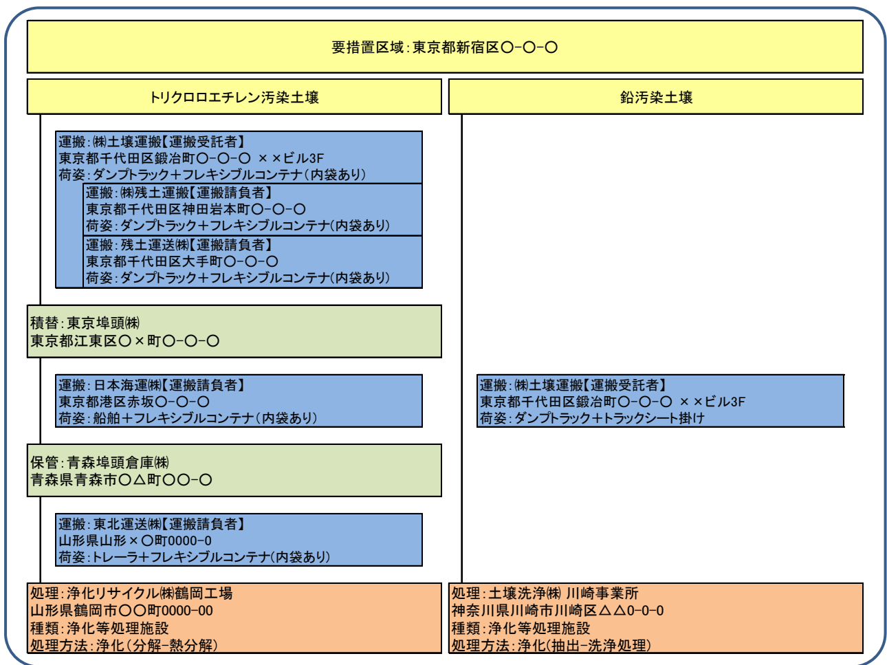
図 2.1.1-2 運搬フロー図の記載例
