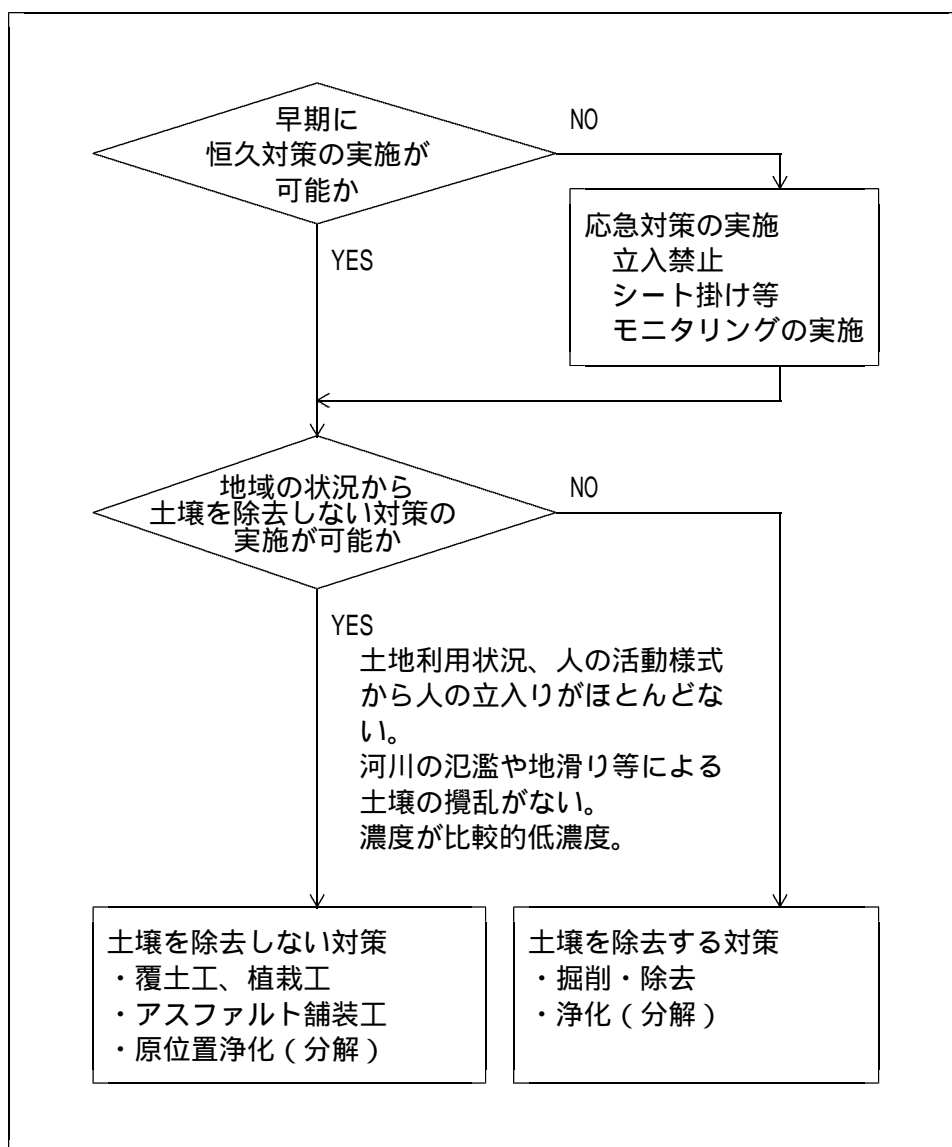
図6 ダイオキシン類汚染土壌対策手法選定に係るフロー
