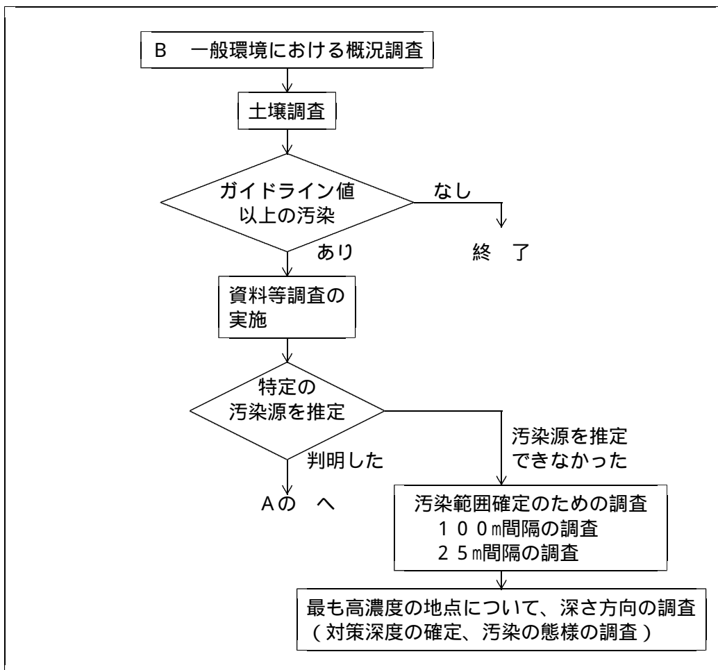
図5 ダイオキシン類汚染土壌調査に係るフロー
