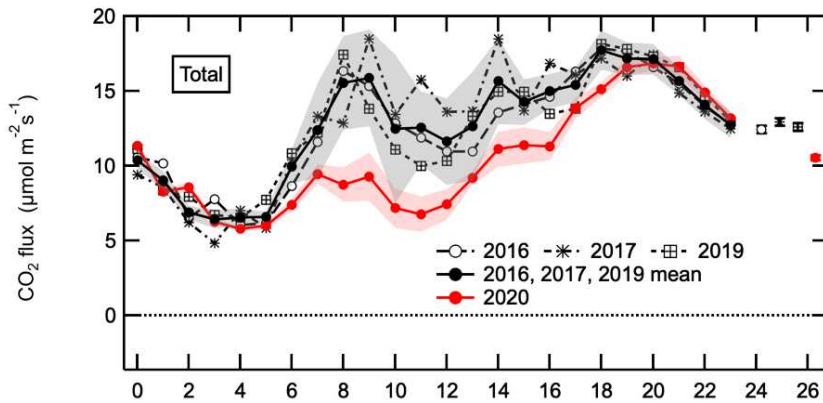
図 1-2 東京代々木街区における各年の CO 2 排出量の日変動。2020 年コロナ禍の期間を赤色で示す。
