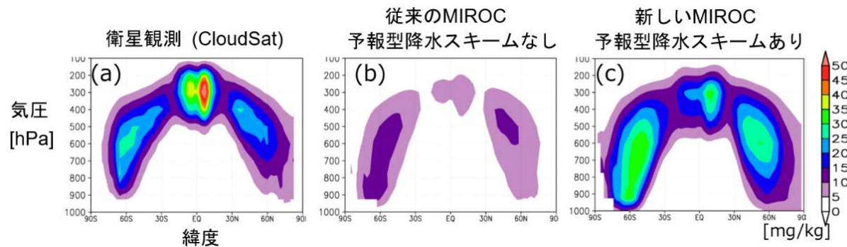
図 1-3 新スキームを導入した際の MIROC 気候モデルにおける降水粒子の分布。新スキームの導入により衛星観測をよく再現していることがわかる。
