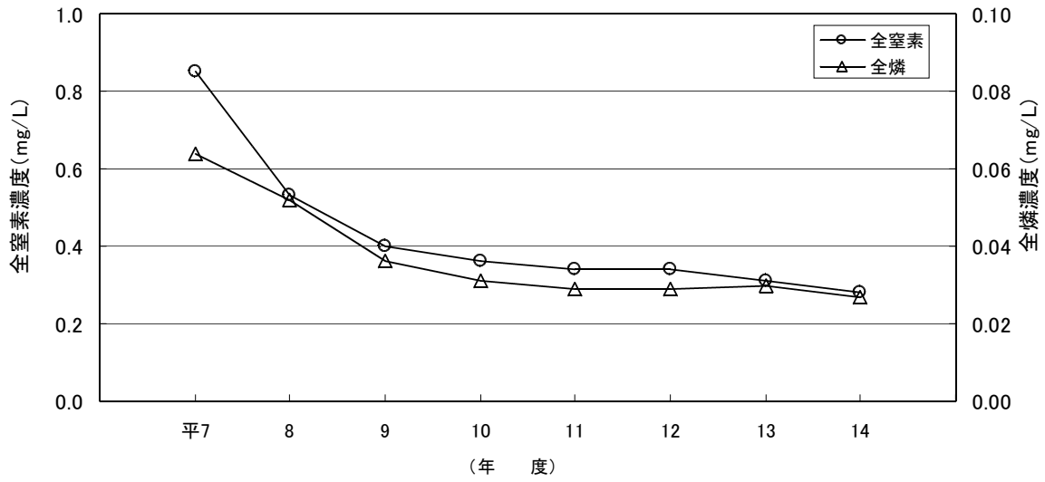
海域における全窒素及び全磷の濃度推移
