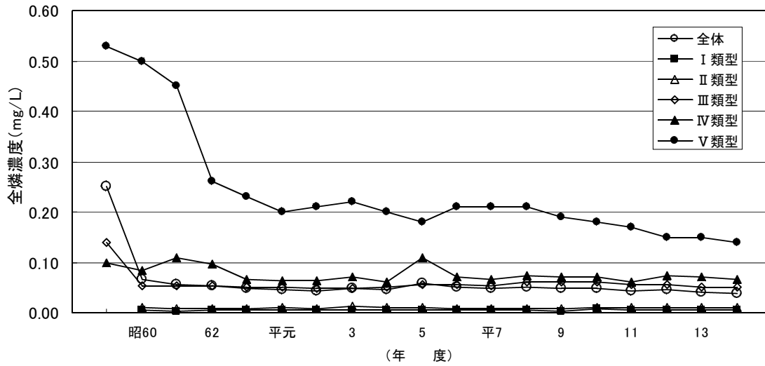
湖沼における類型別全磷濃度推移
