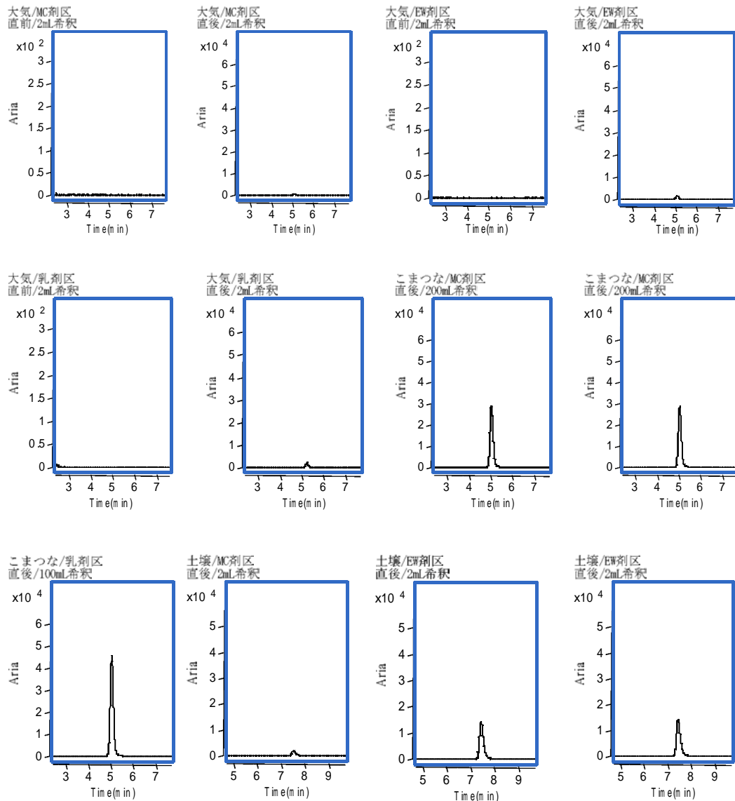
図 処理区試料のクロマトグラム
