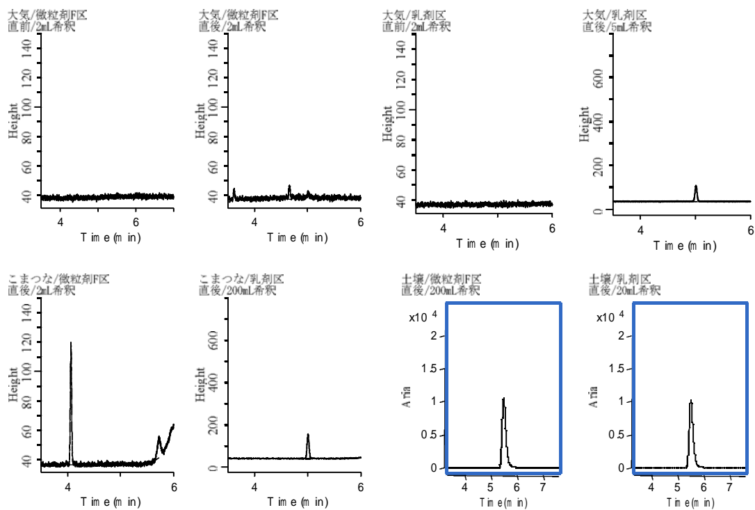
図 処理区試料のクロマトグラム
