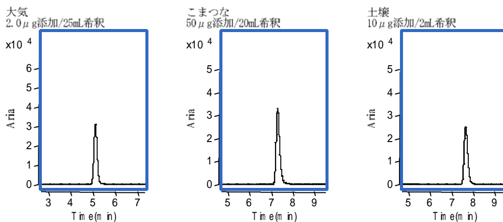
図 添加回収試験のクロマトグラム
