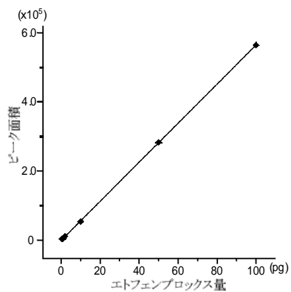
図 検量線の一例
