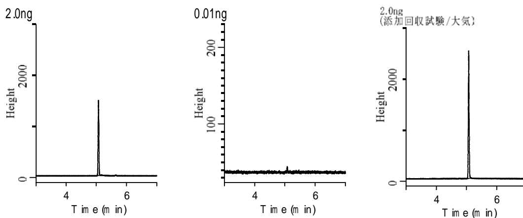
図 標準品のクロマトグラム
