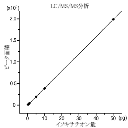
図 検量線の一例
