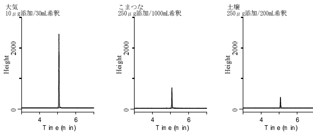
図 添加回収試験のクロマトグラム
