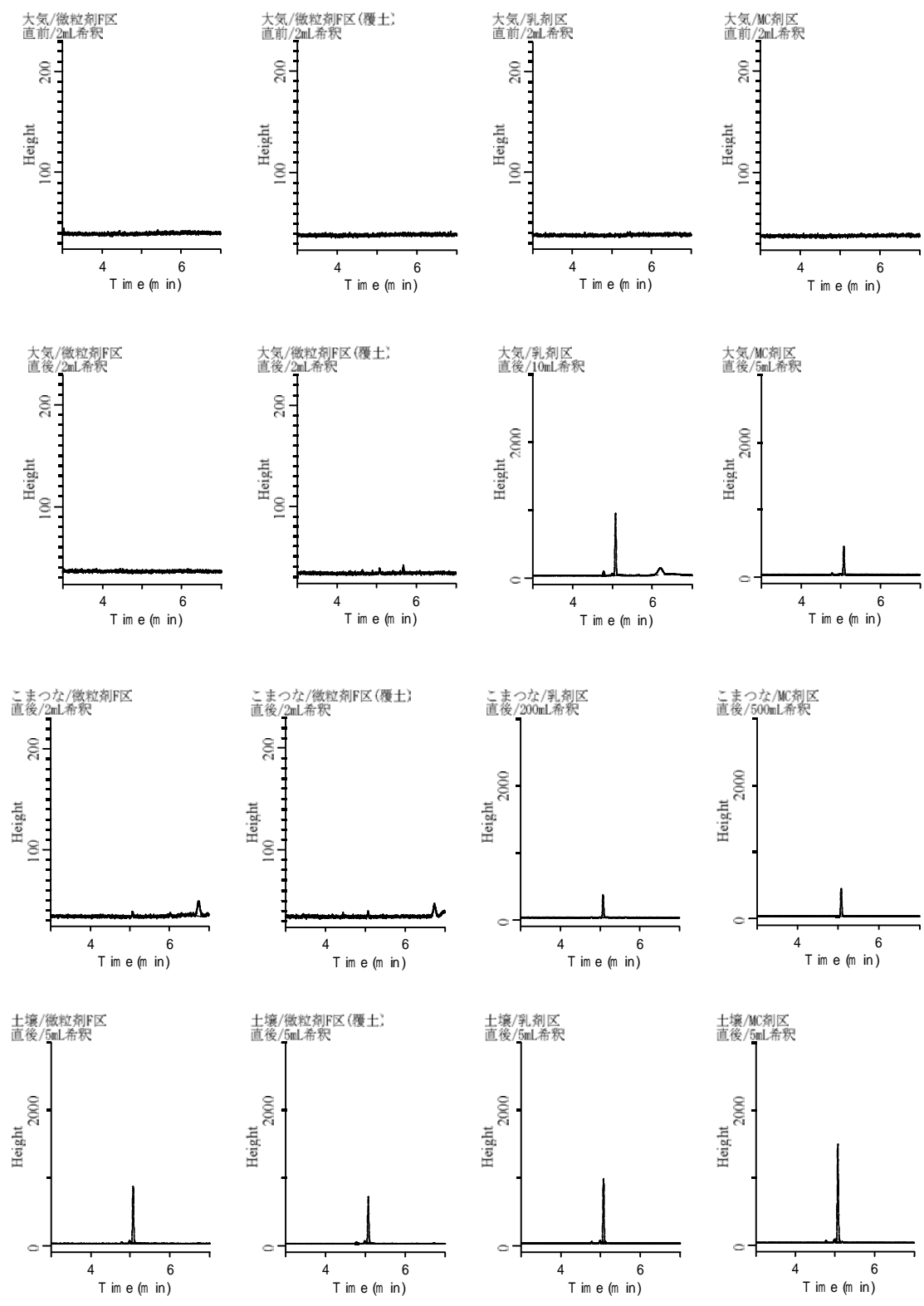
図 処理区試料のクロマトグラム
