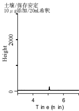
図 保存安定性試験のクロマトグラム (土壌)
