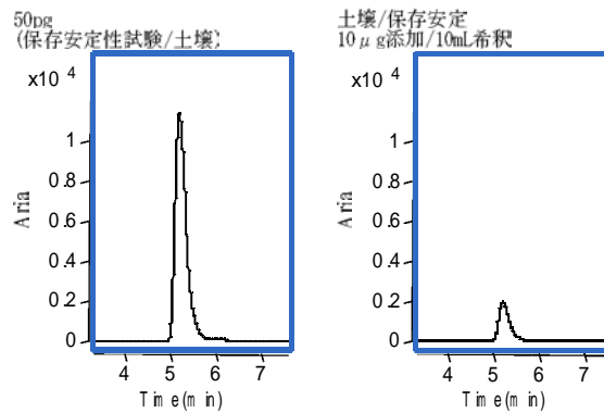
図 保存安定性試験のクロマトグラム(土壌)
