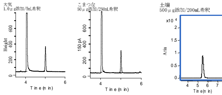
図 添加回収試験のクロマトグラム
