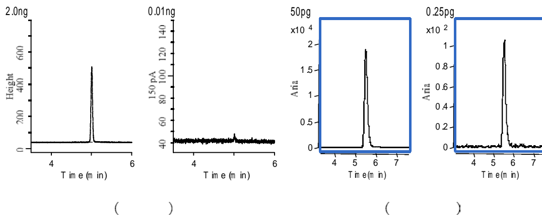
図 検量線の一例
