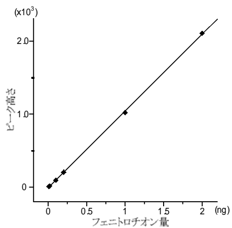
図 検量線の一例
