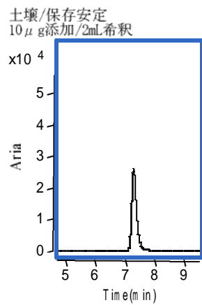
図 保存安定性試験のクロマトグラム(土壌)
