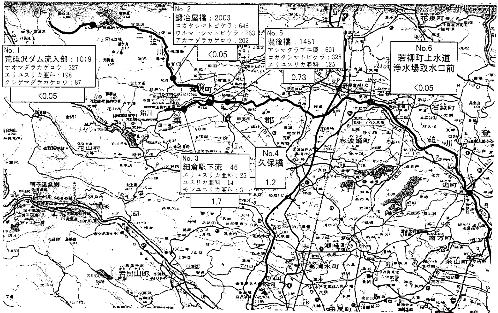
図7 調査地点ごとの底生動物の総個体数、主要出現種の個体数および亜鉛濃度 (mg/L)
