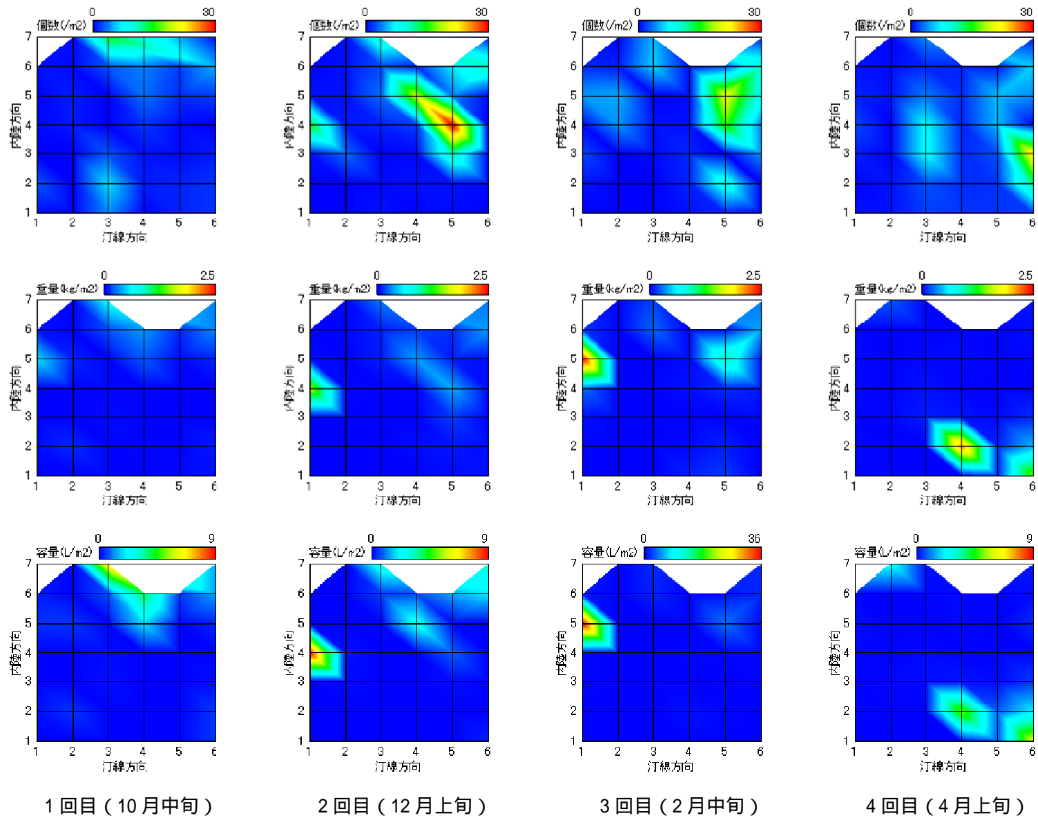
図 10 漂着ゴミの水平分布図 (石垣)
