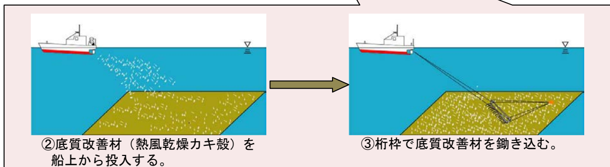
図 1 方策の実施手順 (例)
