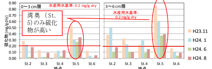
局所的な底質の悪化 (全硫化物の現地調査結果)
