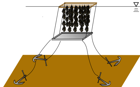
人工中層海底の設置（イメージ）
