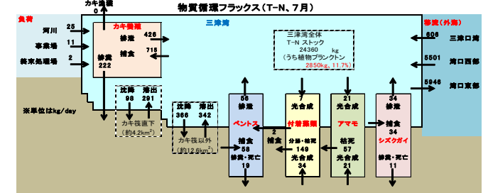
シミュレーションによる三津湾の再現結果
