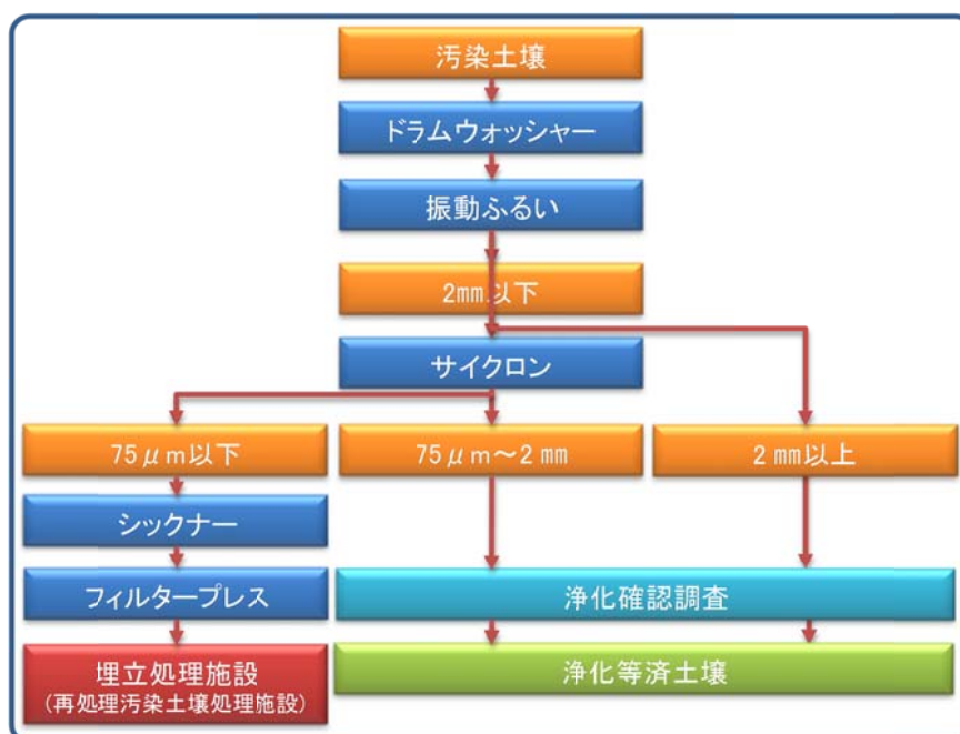
図 2.1.3-4 洗浄処理における処理工程図の例
