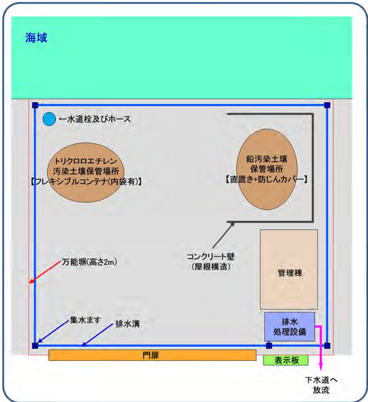
図 2.1.2-3 保管施設の配置図の例
