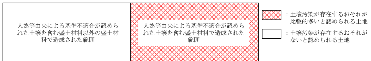
図 2.4.1-6 土壤汚染のおそれの区分の判断ケース⑥ (土壤汚染状況調査の対象地の盛土部分の土壤に人為等由来のみによる基準不適合が認められた場合)
