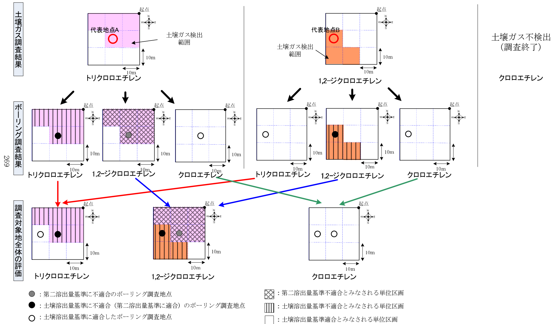
図 2.7.3-3(1) 親物質と分解生成物が土壌ガス調査で検出され、ボーリング調査を実施した結果の評価方法
