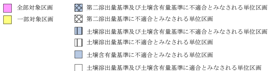
(d) 30m格子内の汚染範囲確定のための個別試料採取をいくつかの30m格子において省略した例(左)とその時の土壌汚染の状態の評価(右)
