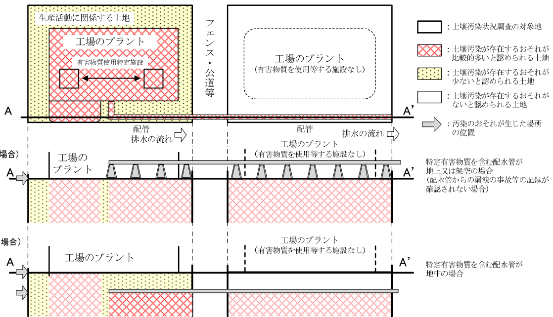
図 2.4.1-2 土壤汚染のおそれの区分の判断ケース②（工場又は事業場、その2）
