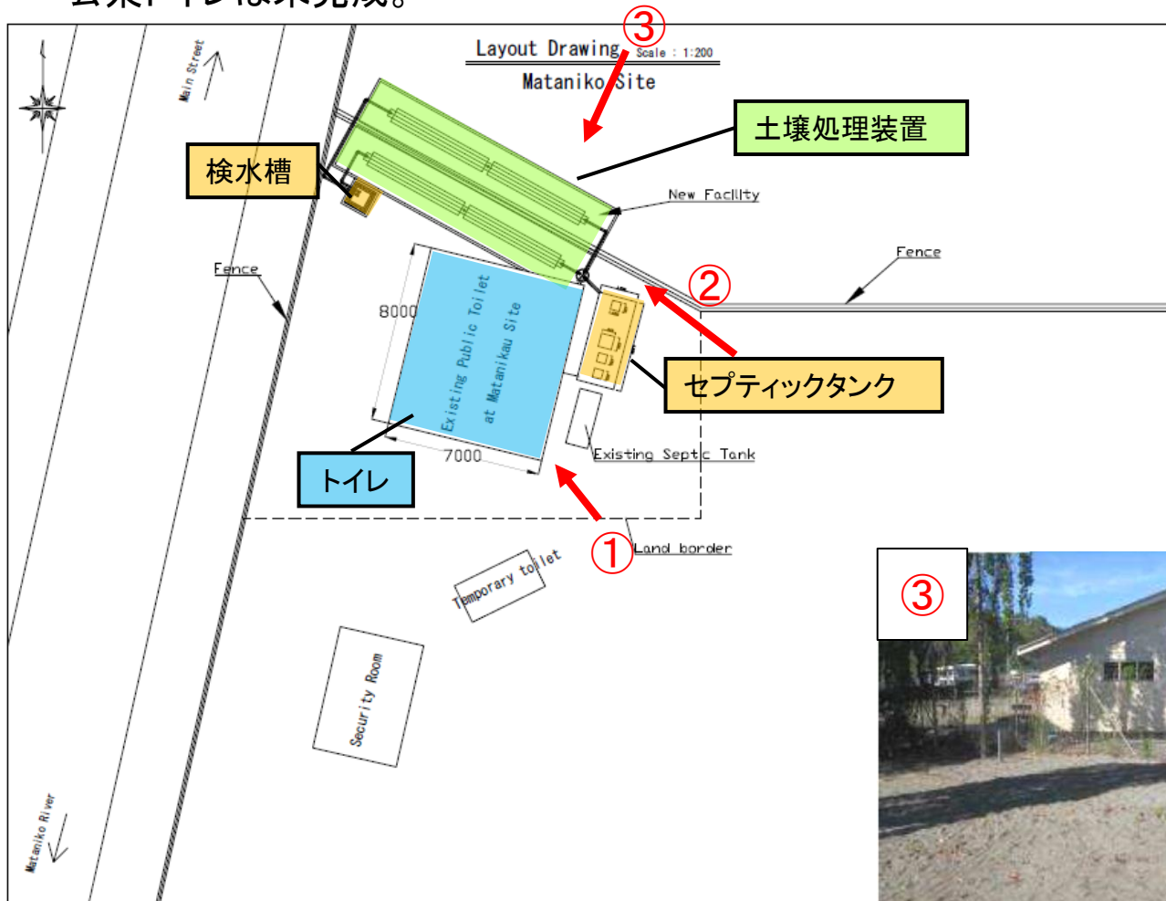
【図7:TSS平面概要】
