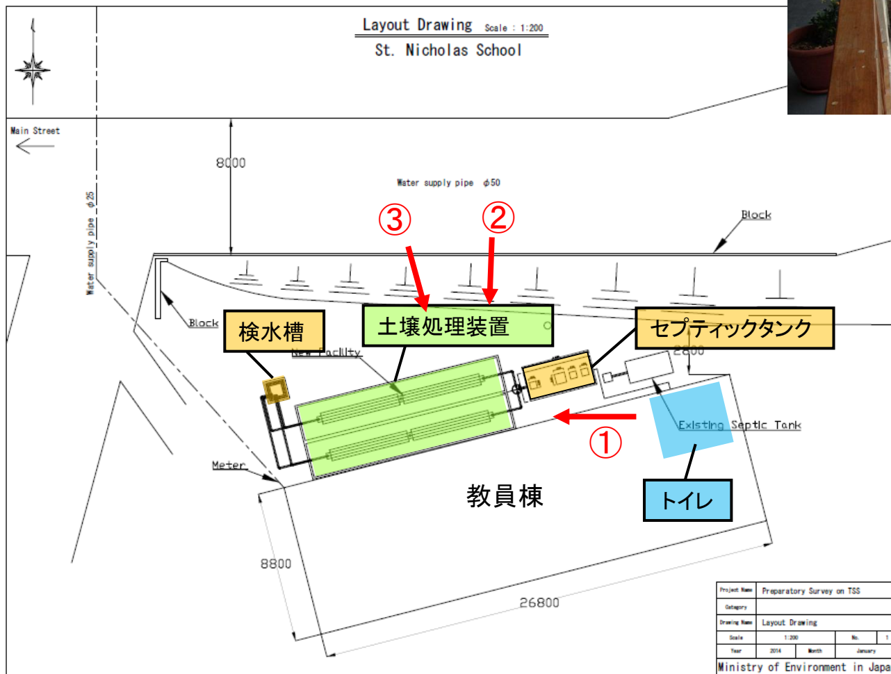
【図6: TSS平面概要】
