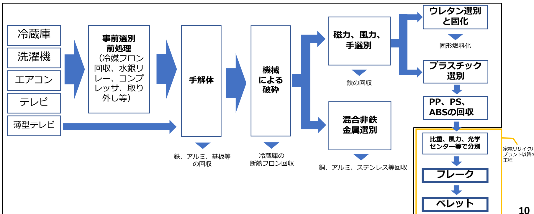
＜家電リサイクルプラントにおける廃家電処理とプラスチック選別の流れの例＞
