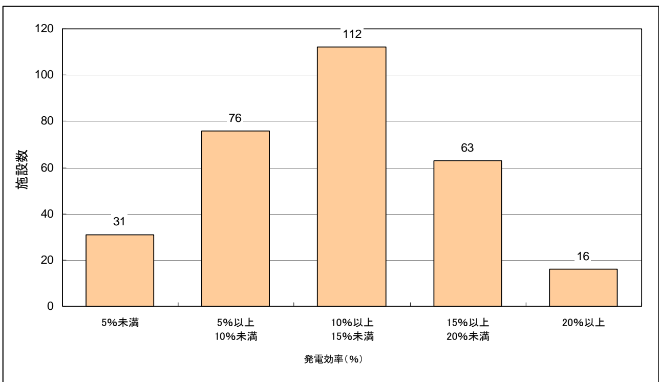
図－１４ ごみ焼却施設の発電効率別の施設数
