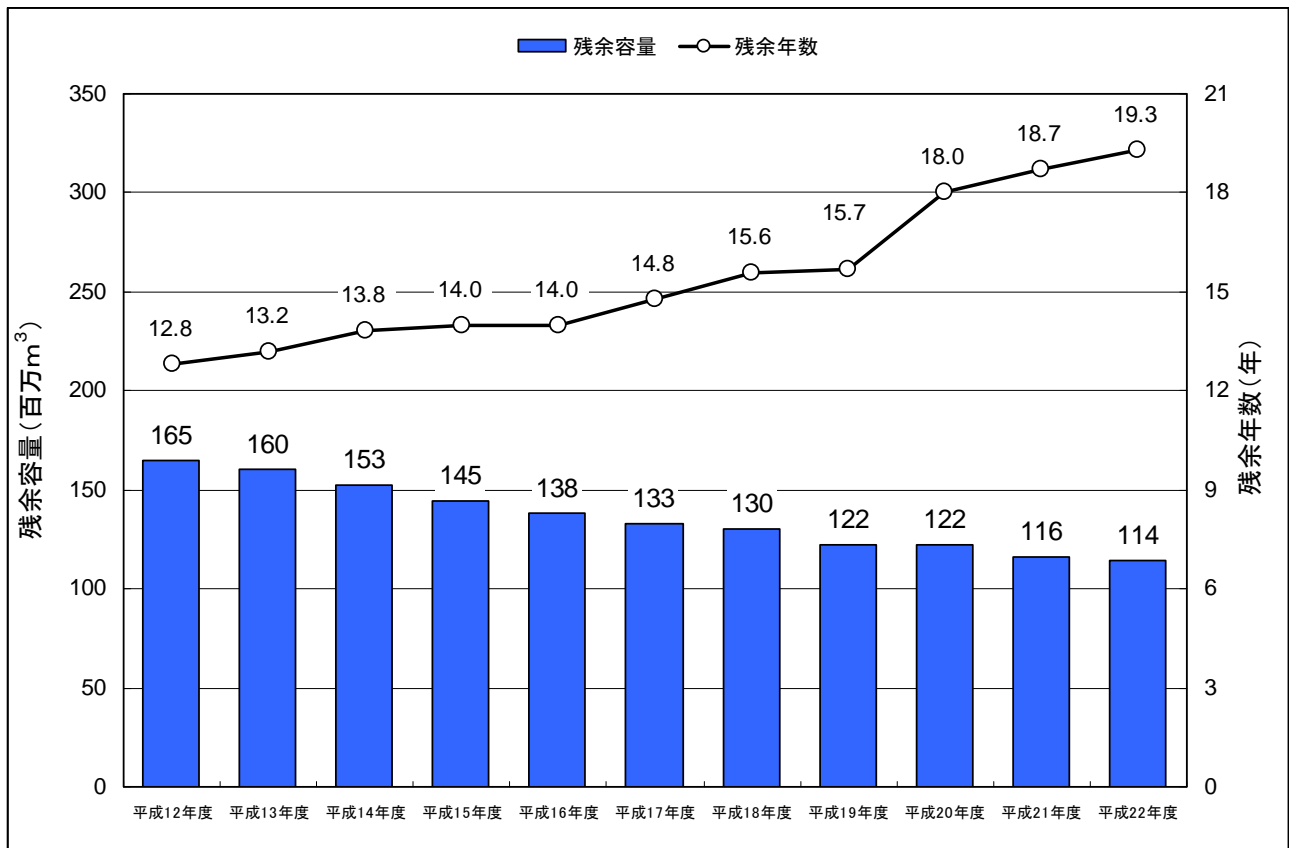
図－18 一般廃棄物最終処分場の残余容量と残余年数の推移 (注13)
