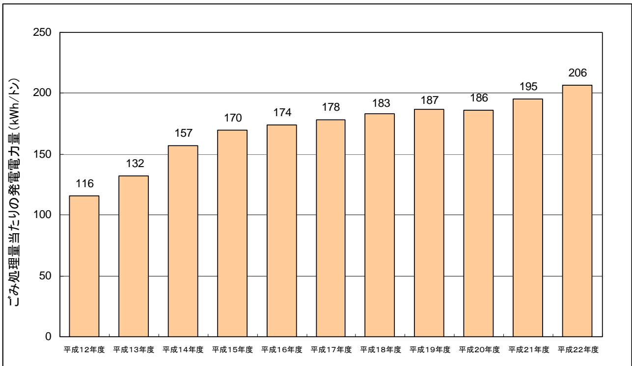
図－１３ ごみ処理量当たりの発電電力量（注9）
