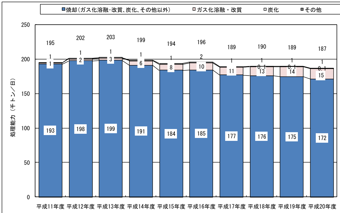
図-10 ごみ焼却施設の種別処理能力の推移
