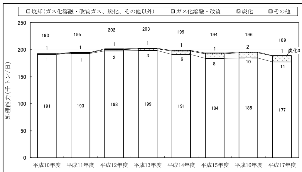
図-11 ごみ焼却施設の種類別処理能力の推移
