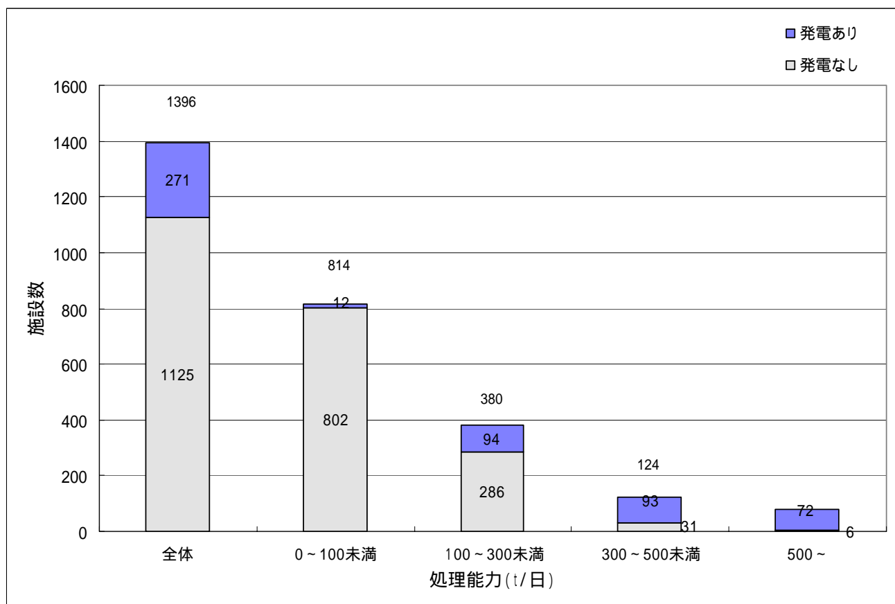
図 - 1 3 処理能力別発電状況
