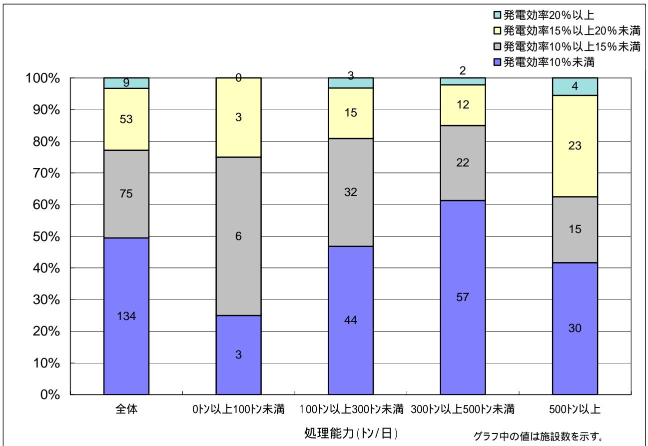
図 - 1 4 処理能力別発電効率状況
