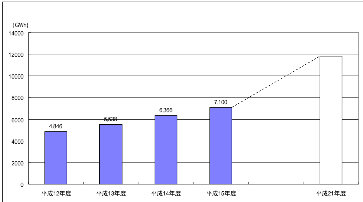
P9のグラフ「図 - 15 総発電電力量の推移」
