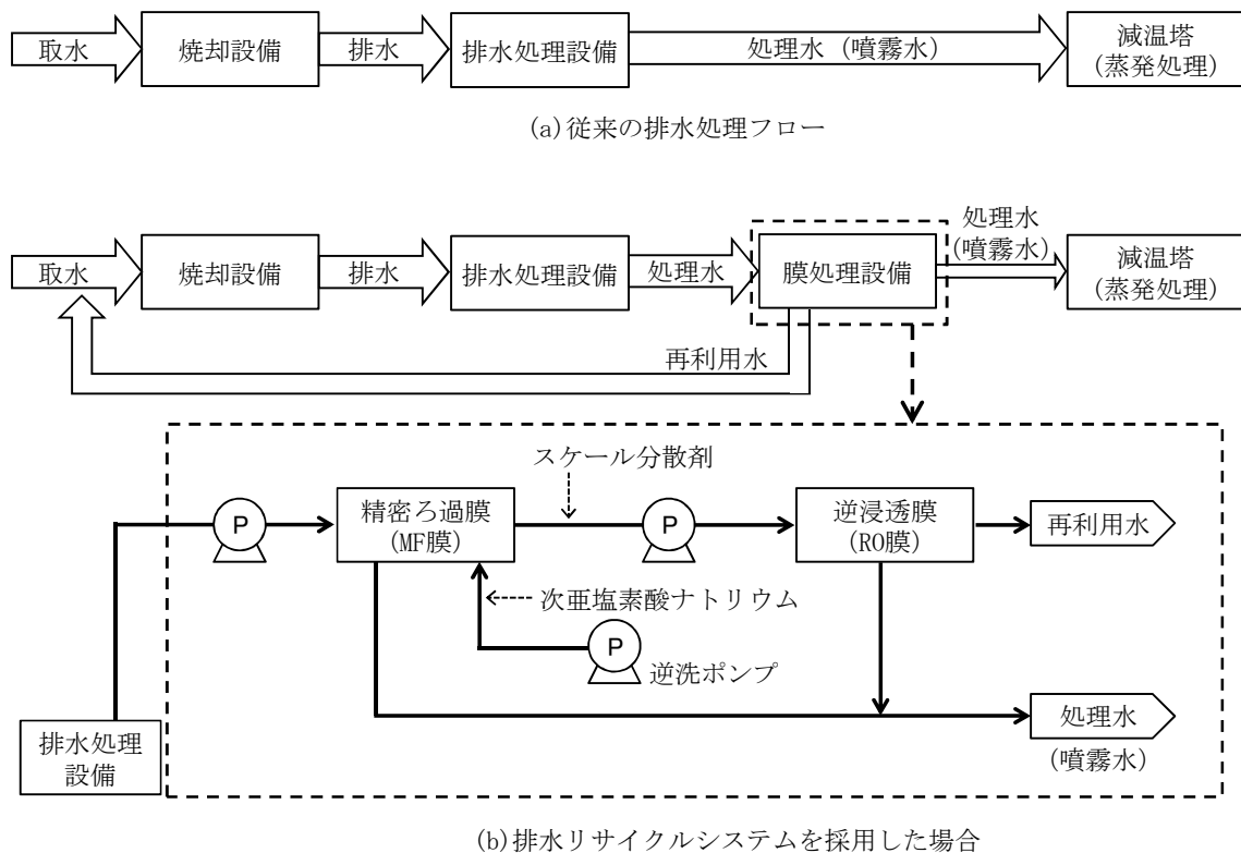
図 I.3.12 焼却設備における排水処理フロー（例）
