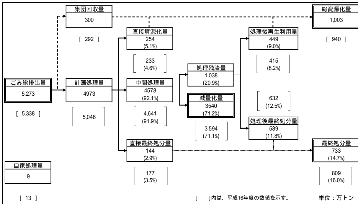
図 - 3 全国のごみ処理のフロー
