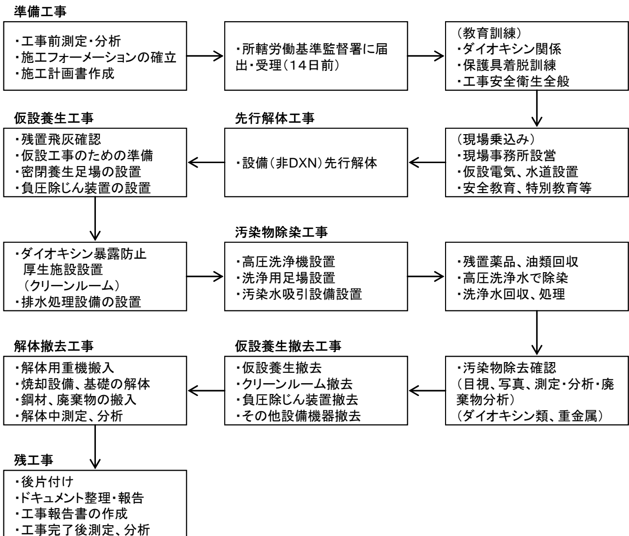
仮設焼却炉の解体・撤去工事フロー（例）
