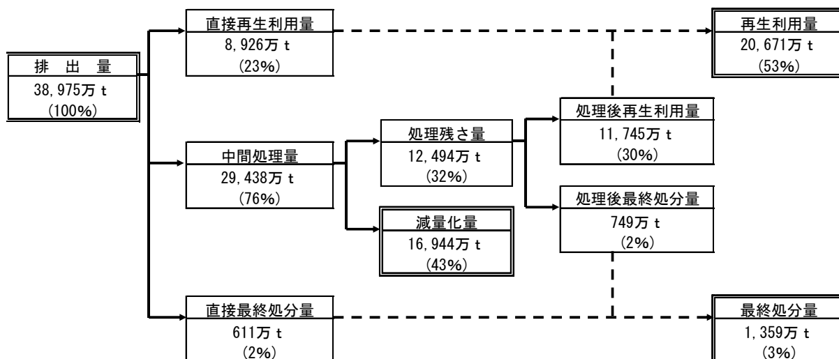
図 3-1-1 産業廃棄物の処理・再資源化の流れ（平成 21 年度）
