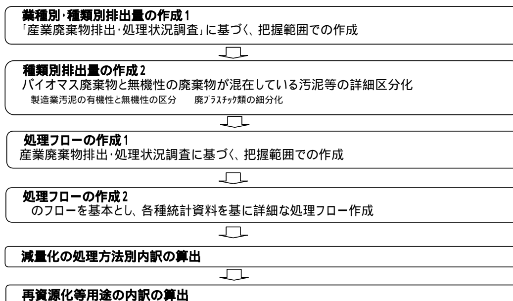
図 3-1-2 産業廃棄物の循環的利用量の推計作業フロー
