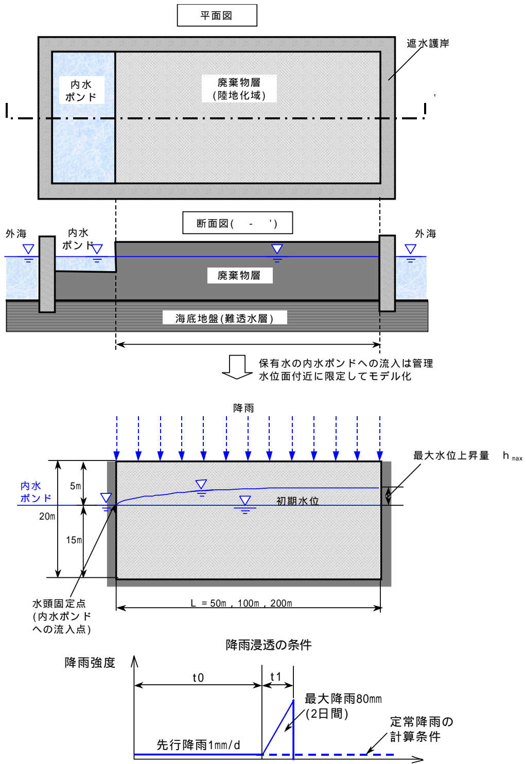
図 - 5.2.1 解析モデルb (浸透流解析) の概要
