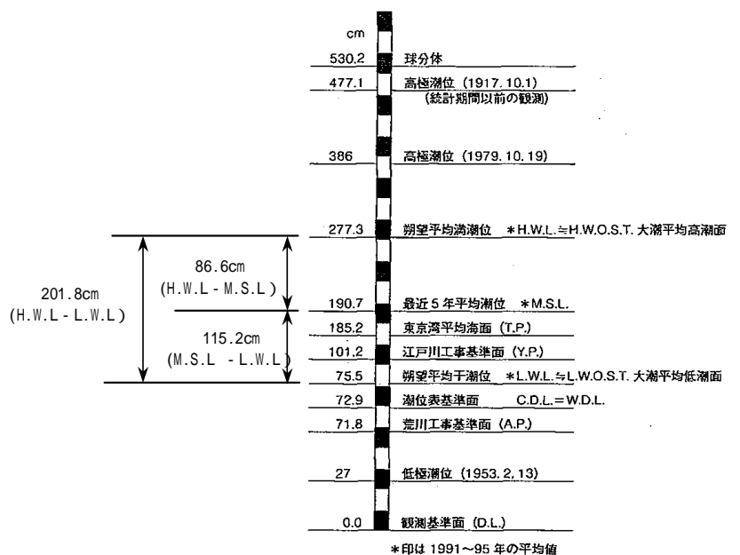
参・図 - 4.1 東京(晴海)検潮所の潮位実況図
