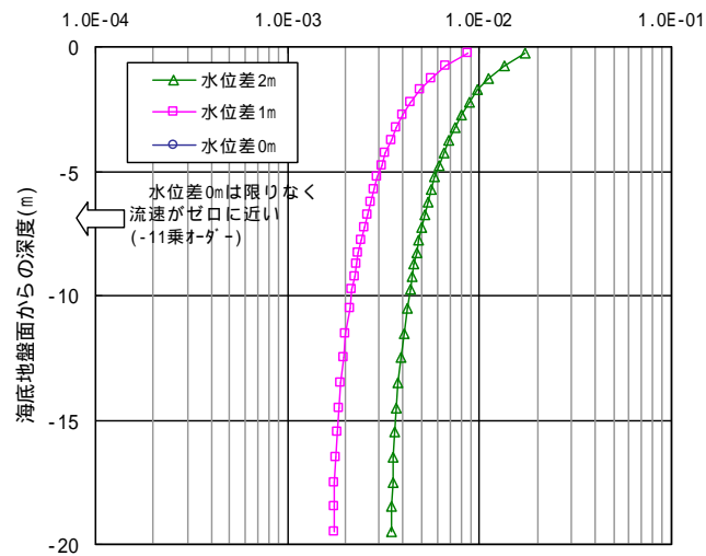
図 - 4.3.3 平均ダルシー流速の深度分布
