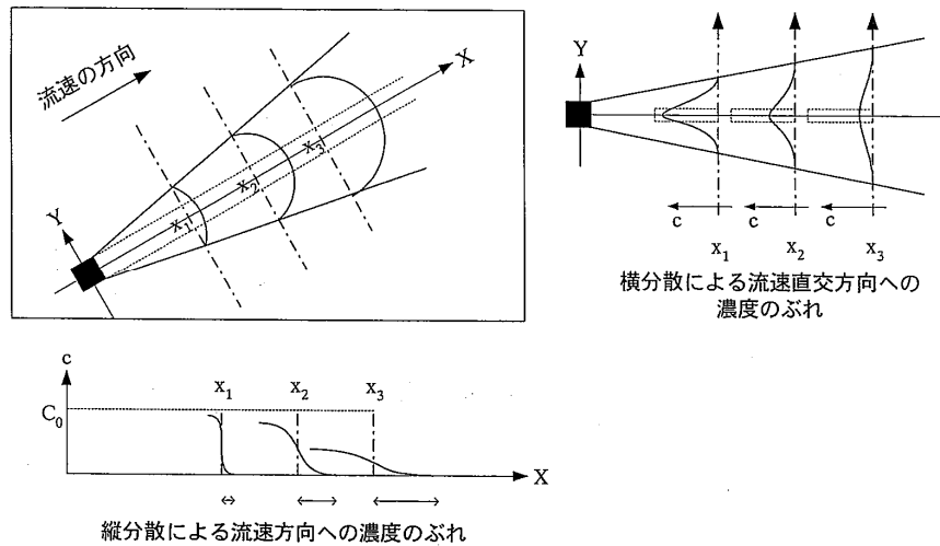
図 - 3.2.5 縦分散, 横分散の概念
