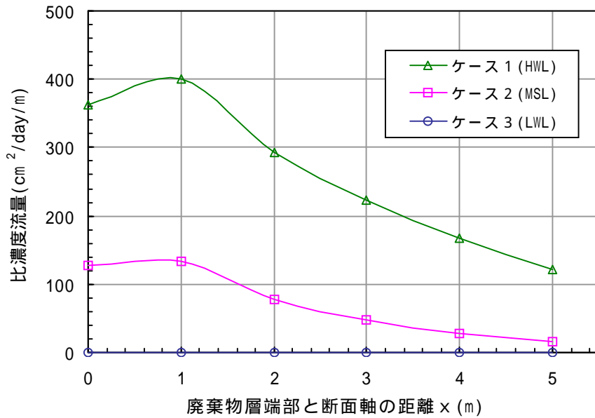
図 - 4.3.5 水平距離 x と比濃度流量の関係（経過年数 50 年を対象）
