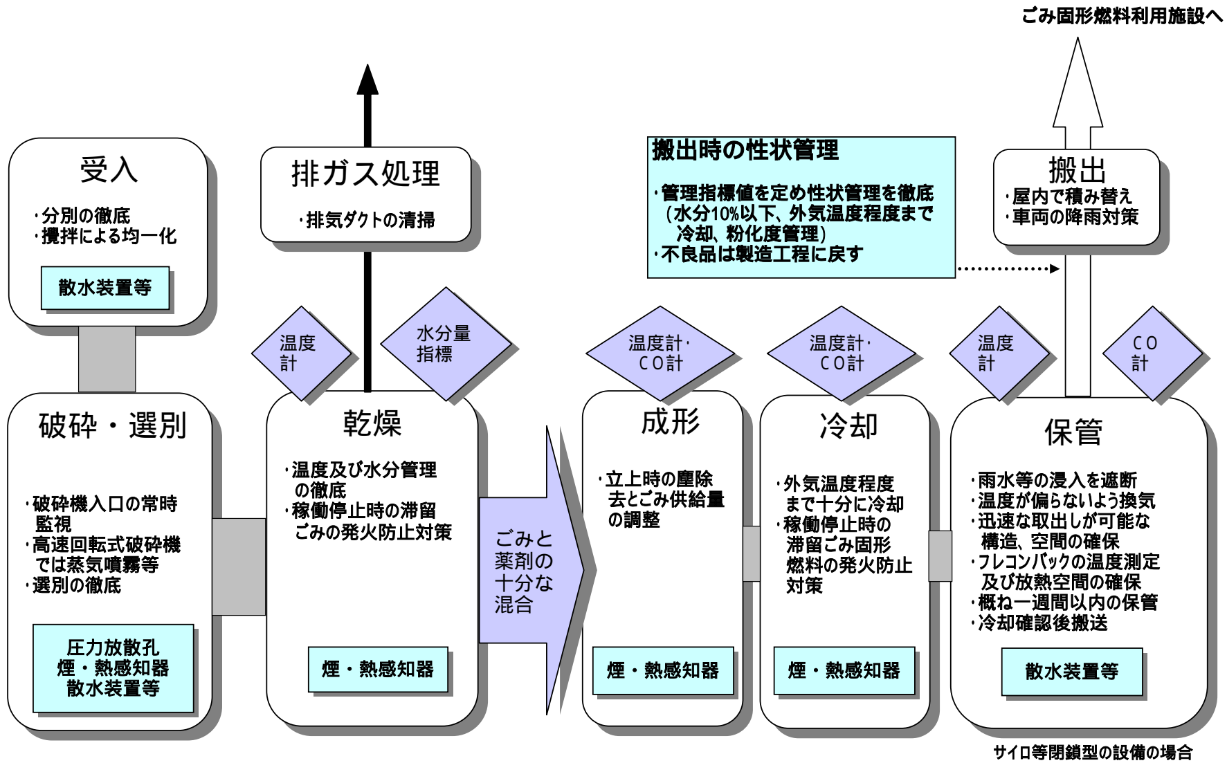
図6-1 ごみ固形燃料化施設における対策のイメージ
