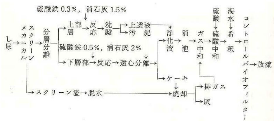
図2.3-5 相生市の施設の処理工程 16)
