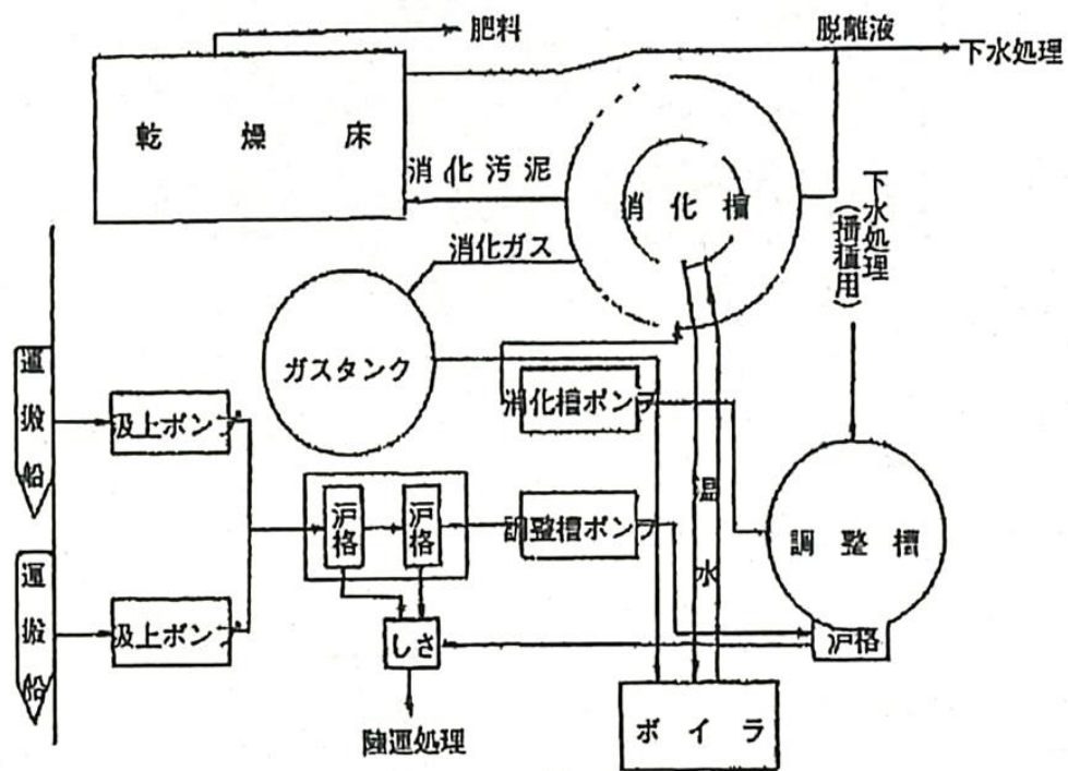
図 2.2-3 砂町し尿消化槽施設平面図 23)
