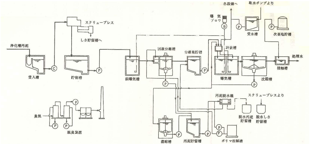
図 2.6-8 前ばっ気方式のフローシート 14)
