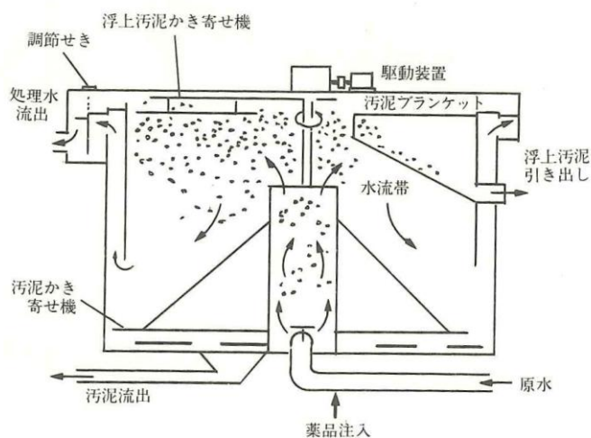
図 2.6-13 固液分離装置 [浮上分離式] の例 18)
