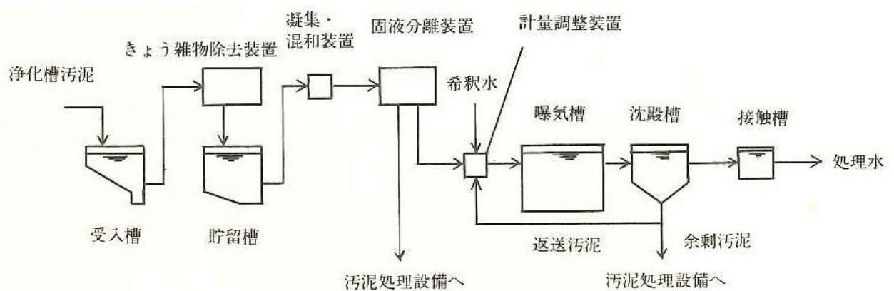
図 2.6-9 前ばっ気を行わない方式のフローシート 15)
