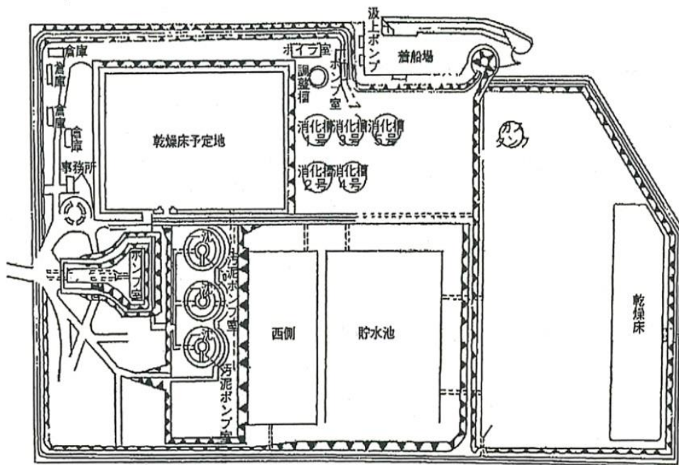
図 2.2-3 砂町し尿消化槽施設平面図 23)
