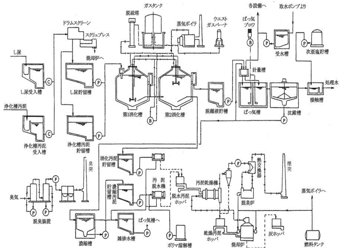
図 2.2-25 嫌気性消化・活性汚泥法処理方式のフローシート (例) 35)
