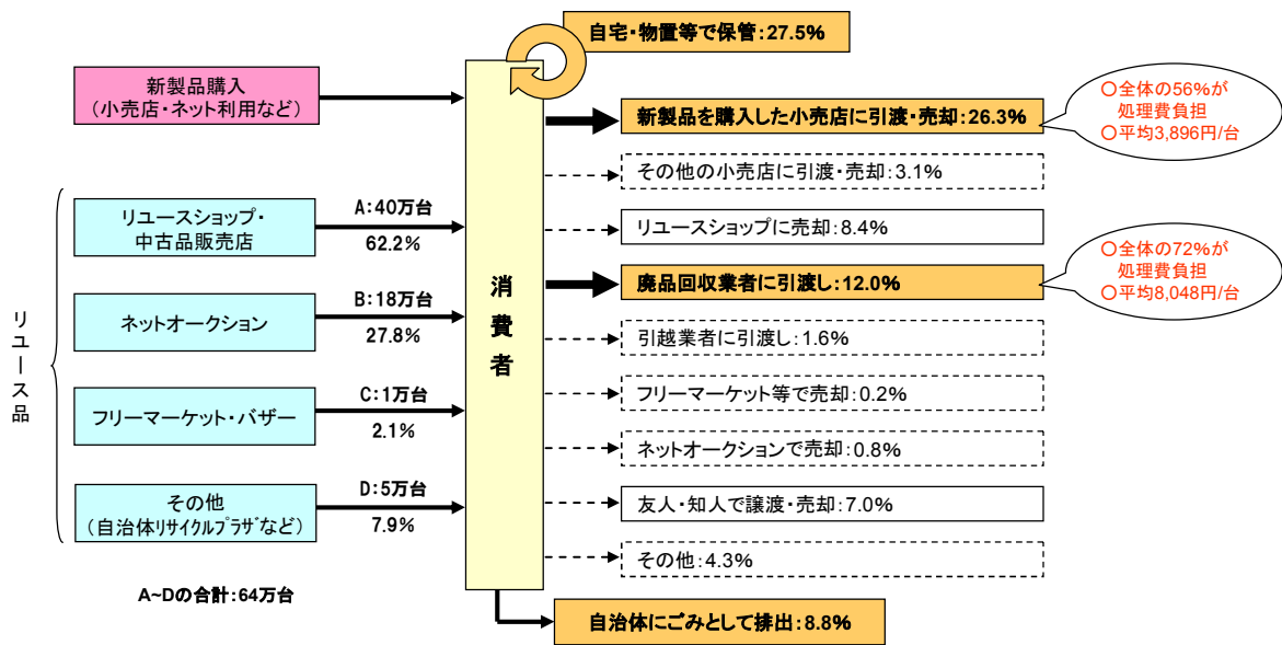
図 71 電気冷蔵庫・冷凍庫の排出・流通実態の推計
